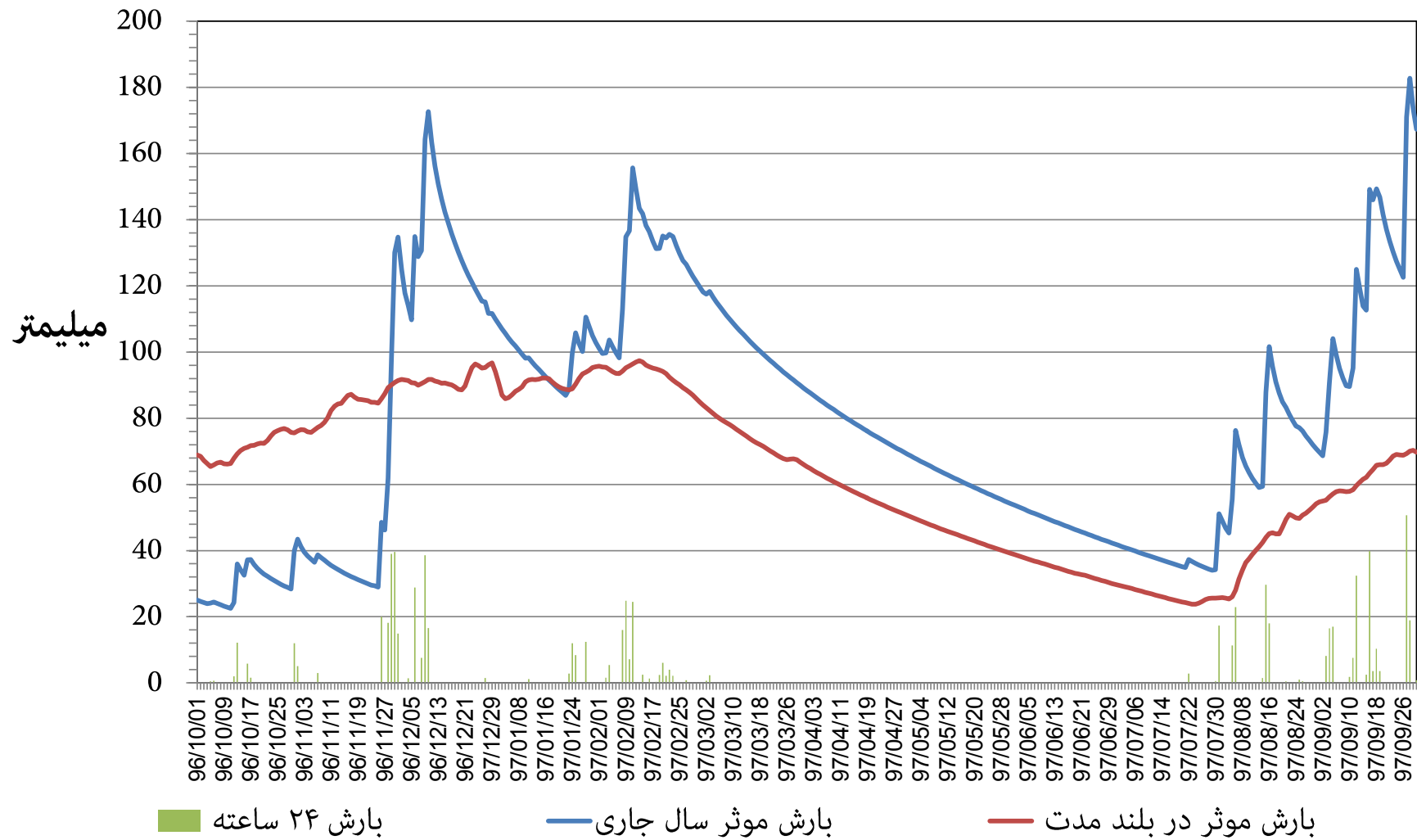
نمودار توزیع زمانی بارش و بارش موثر ۳۶۵ روزه ایستگاه باران سنجی محکمی (وزارت نیرو) استان کرمانشاه دوره ۱۲ ماهه تا پایان آذر ماه ۱۳۹۷
