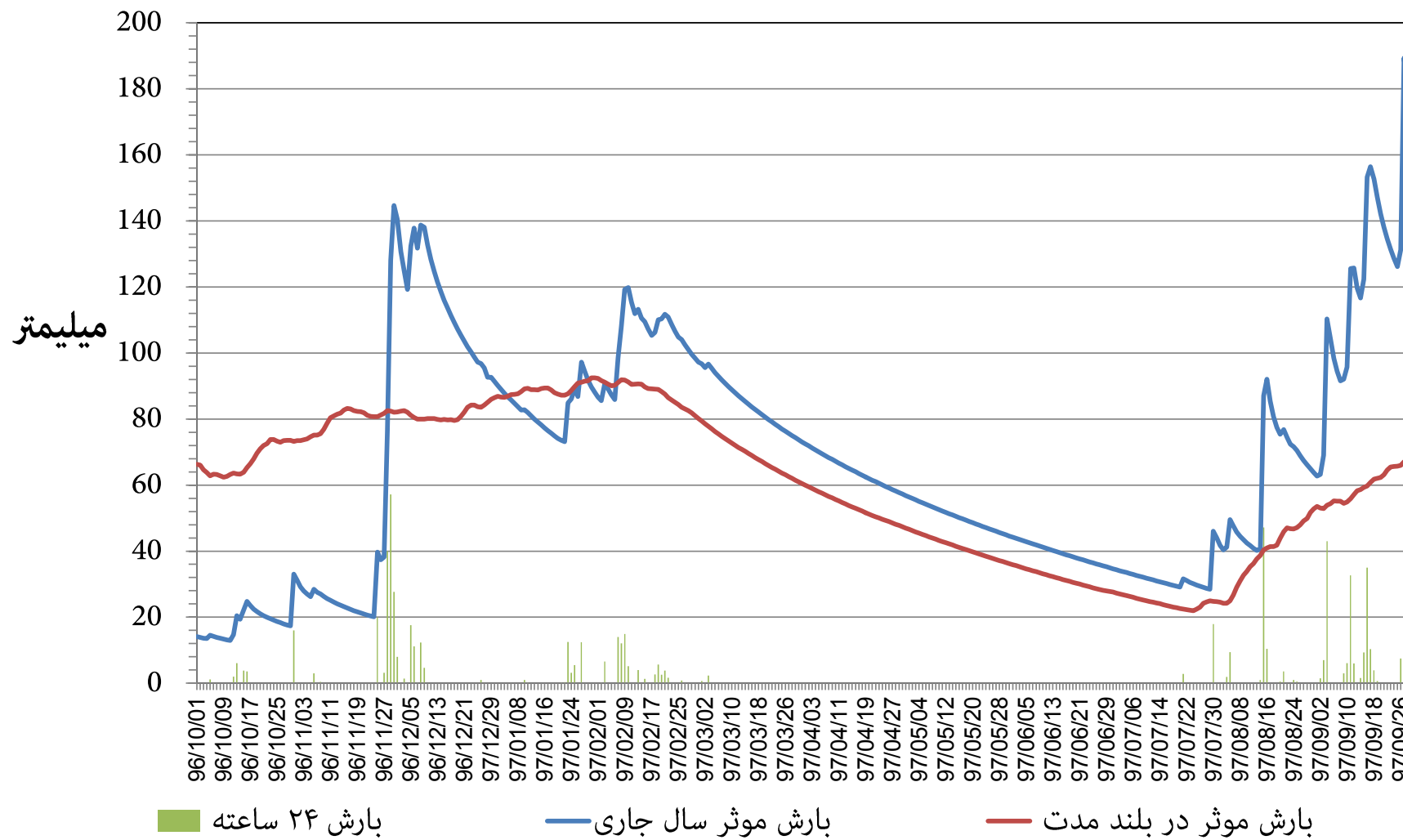
نمودار توزیع زمانی بارش و بارش موثر ۳۶۵ روزه ایستگاه هواشناسی سرپل ذهاب استان کرمانشاه دوره ۱۲ ماهه تا پایان آذر ماه ۱۳۹۷
