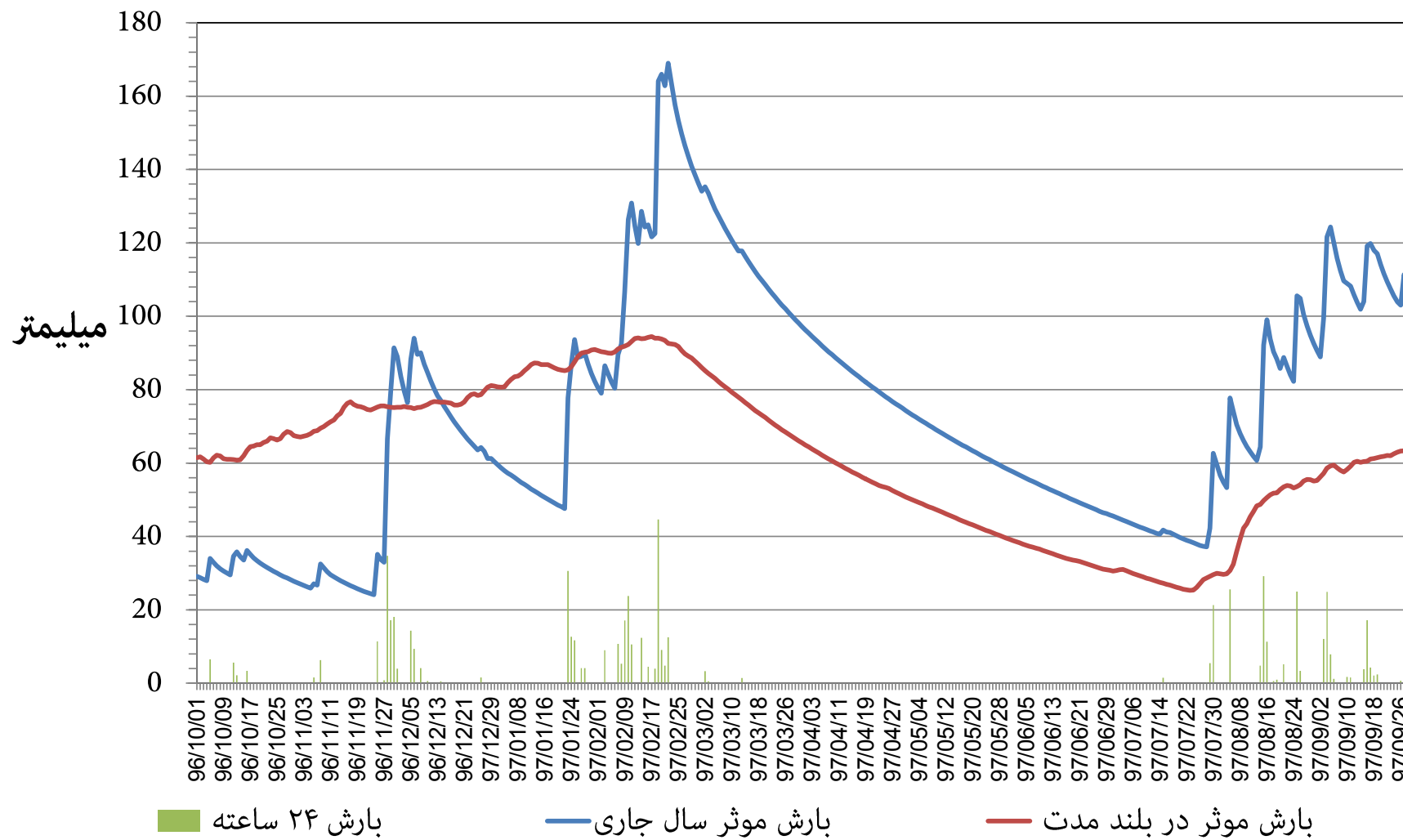
نمودار توزیع زمانی بارش و بارش موثر ۳۶۵ روزه ایستگاه هواشناسی کرمانشاه استان کرمانشاه دوره ۱۲ ماهه تا پایان آذر ماه ۱۳۹۷
