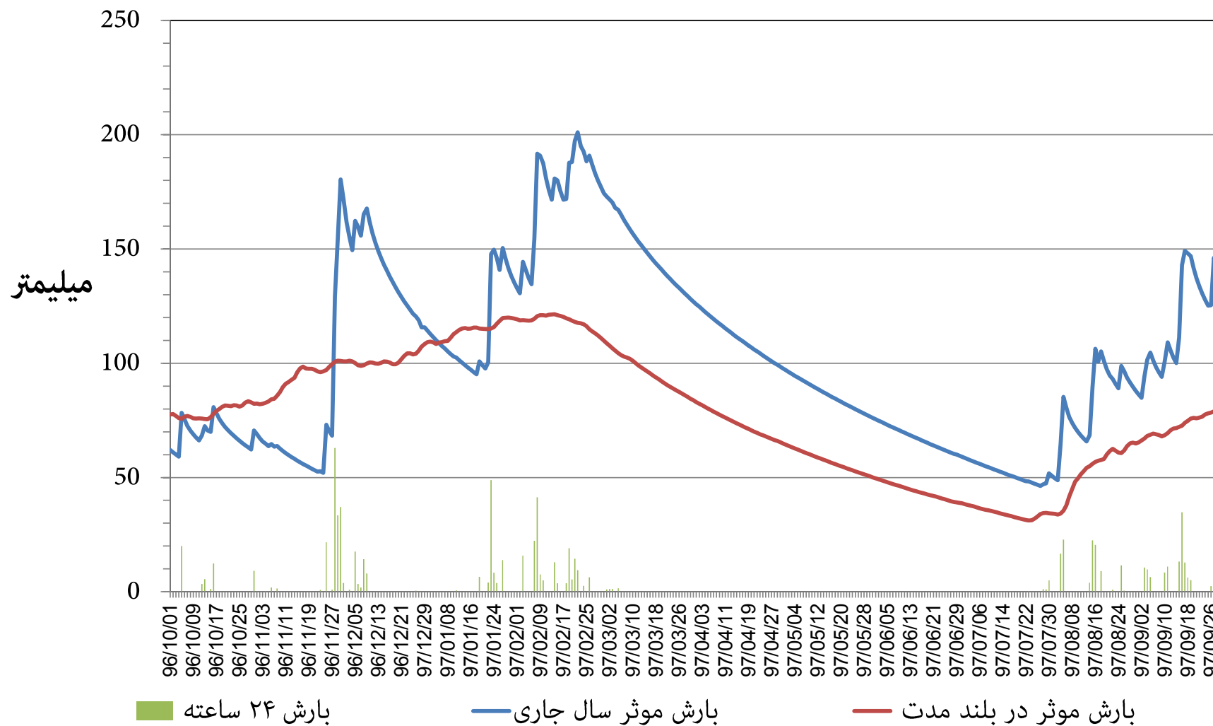
مقدار توزیع زمانی بارش و بارش موثر ۳۶۵ روزه ایستگاه هواشناسی روانسر استان کرمانشاه دوره ۱۲ ماهه تا پایان آذر ماه ۱۳۹۷
