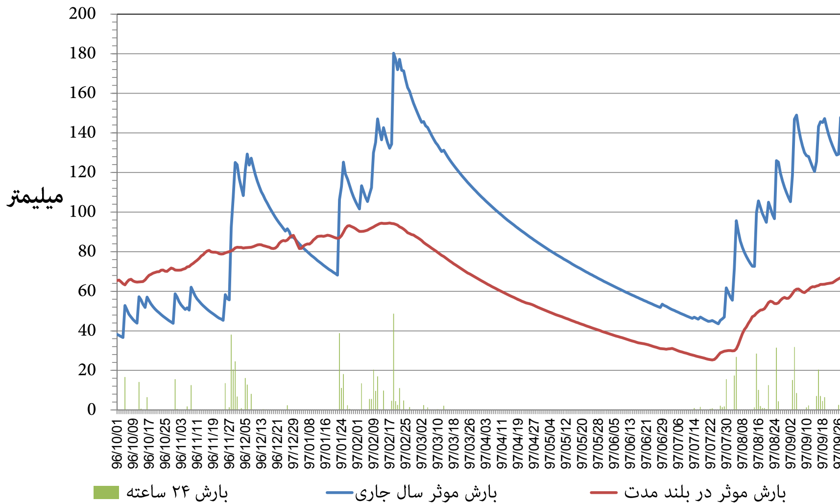
نمودار توزیع زمانی بارش و بارش موثر ۳۶۵ روزه ایستگاه هواشناسی سرآرود (کرمانشاه) استان کرمانشاه دوره ۱۲ ماهه تا پایان آذر ماه ۱۳۹۷
