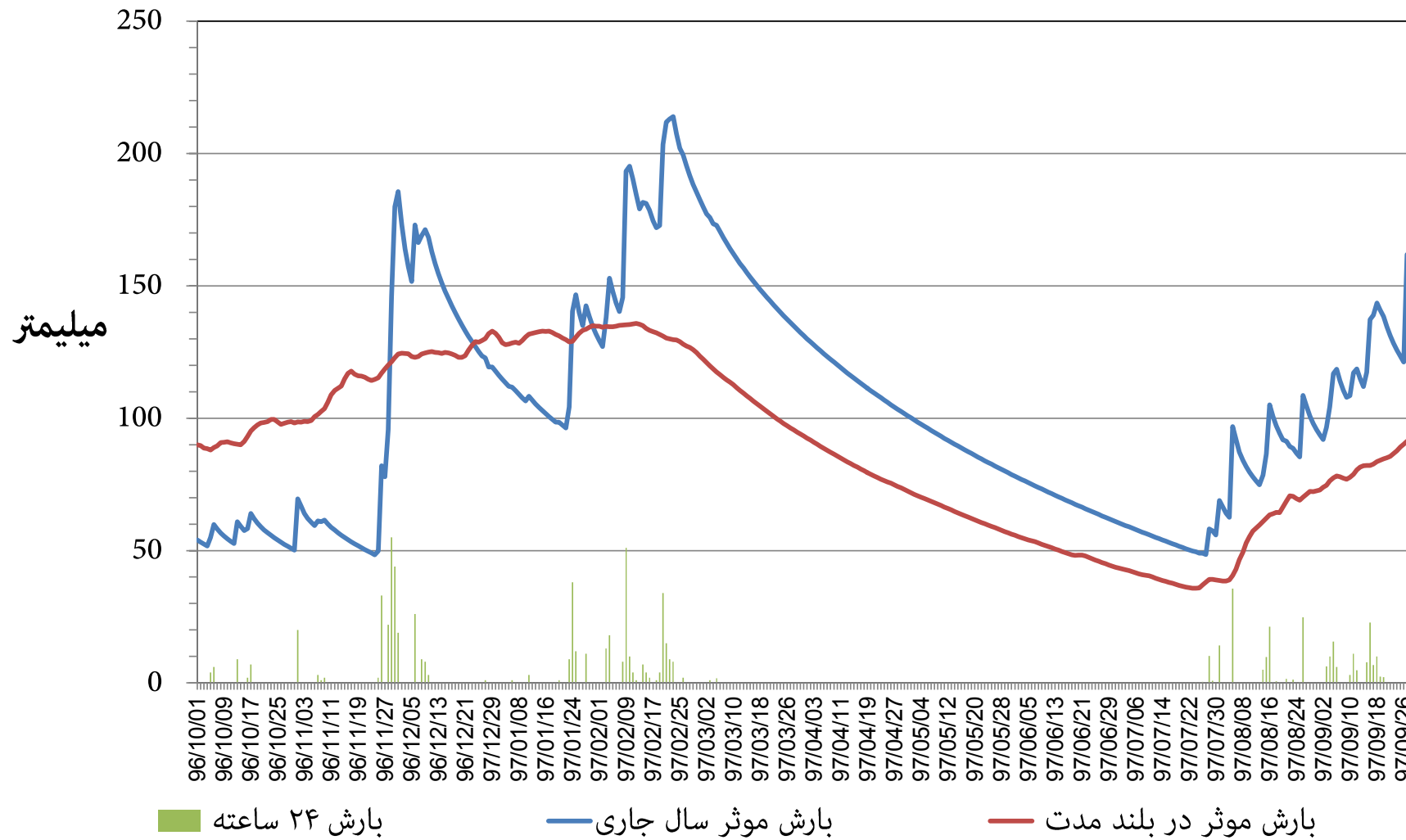
نمودار توزیع زمانی بارش و بارش موثر ۳۶۵ روزه ایستگاه باران سنجی توتشامی (گهواره) (وزارت نیرو) استان کرمانشاه دوره ۱۲ ماهه تا پایان آذر ماه ۱۳۹۷
