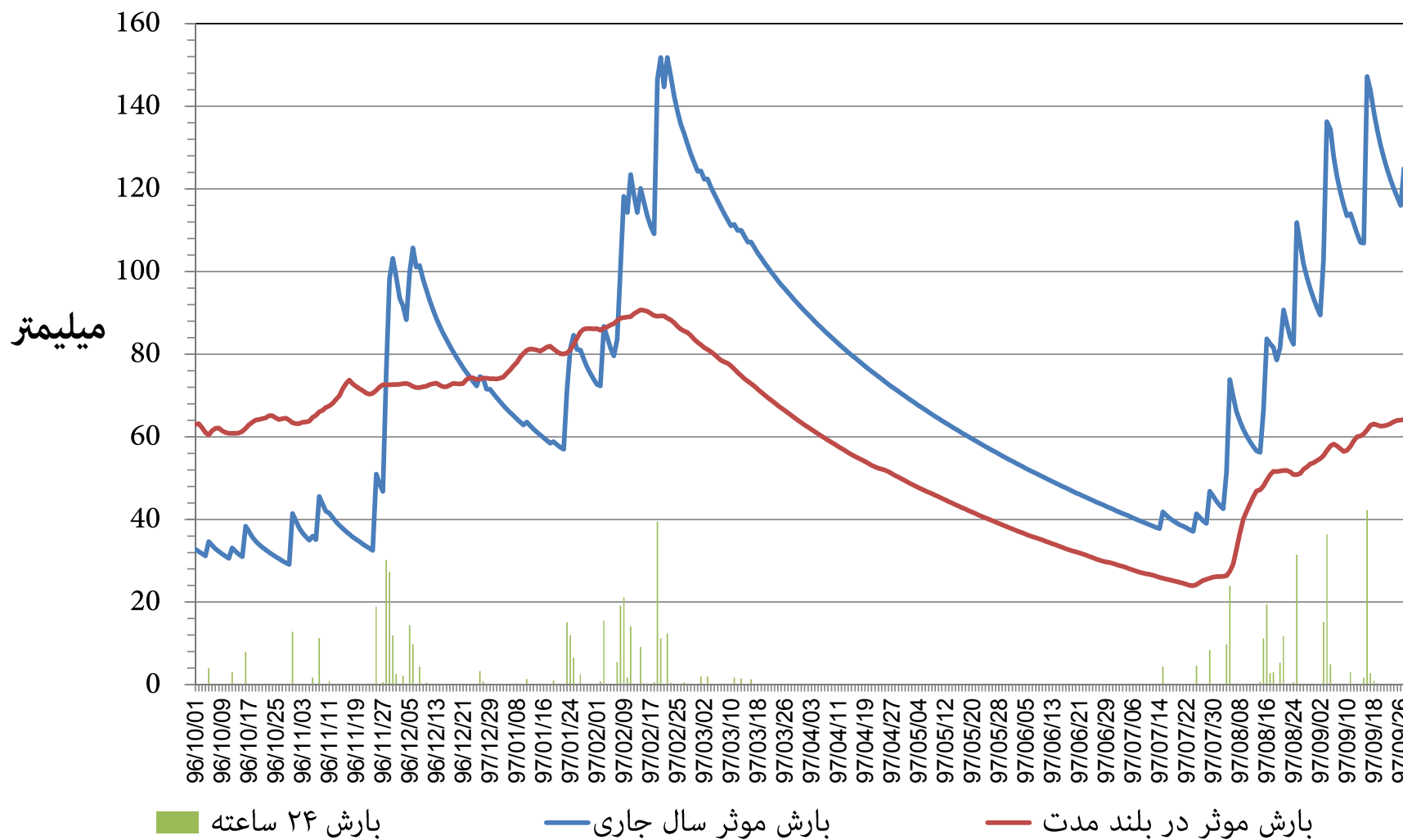
مقدار توزیع زمانی بارش و بارش موثر ۳۶۵ روزه ایستگاه هواشناسی کنگاور استان کرمانشاه دوره ۱۲ ماهه تا پایان آذر ماه ۱۳۹۷
