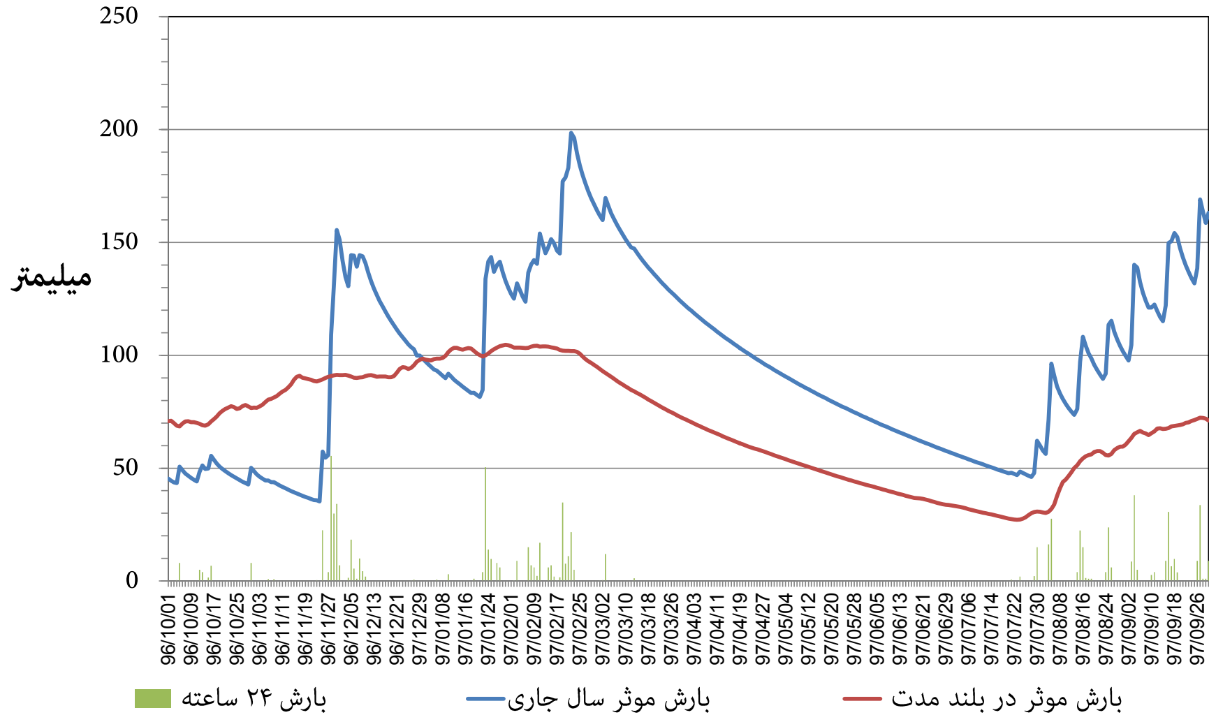
نمودار توزیع زمانی بارش و بارش موثر ۳۶۵ روزه ایستگاه هواشناسی اسلام آباد غرب استان کرمانشاه دوره ۱۲ ماهه تا پایان آذر ماه ۱۳۹۷
