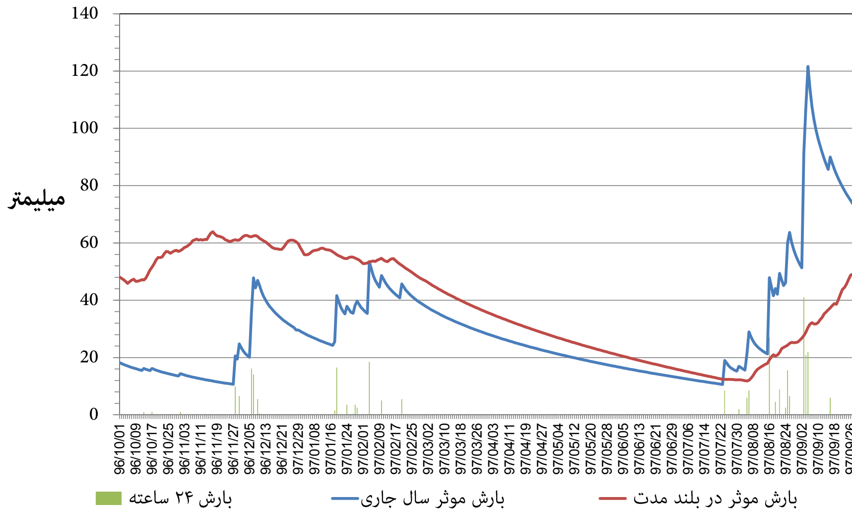
نمودار توزیع زمانی بارش و بارش موثر ۳۶۵ روزه ایستگاه باران سنجی هفت تپه (وزارت نیرو) استان خوزستان دوره ۱۲ ماهه تا پایان آذر ماه ۱۳۹۷
