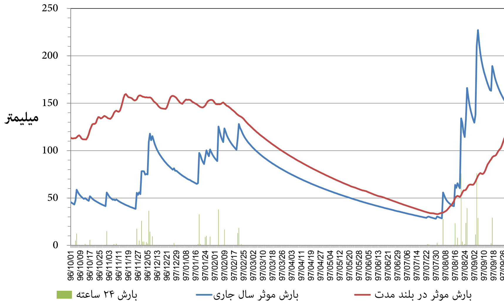
نمودار توزیع زمانی بارش و بارش موثر ۳۶۵ روزه ایستگاه باران سنجی سوسن (وزارت نیرو) استان خوزستان دوره ۱۲ ماهه تا پایان آذر ماه ۱۳۹۷
