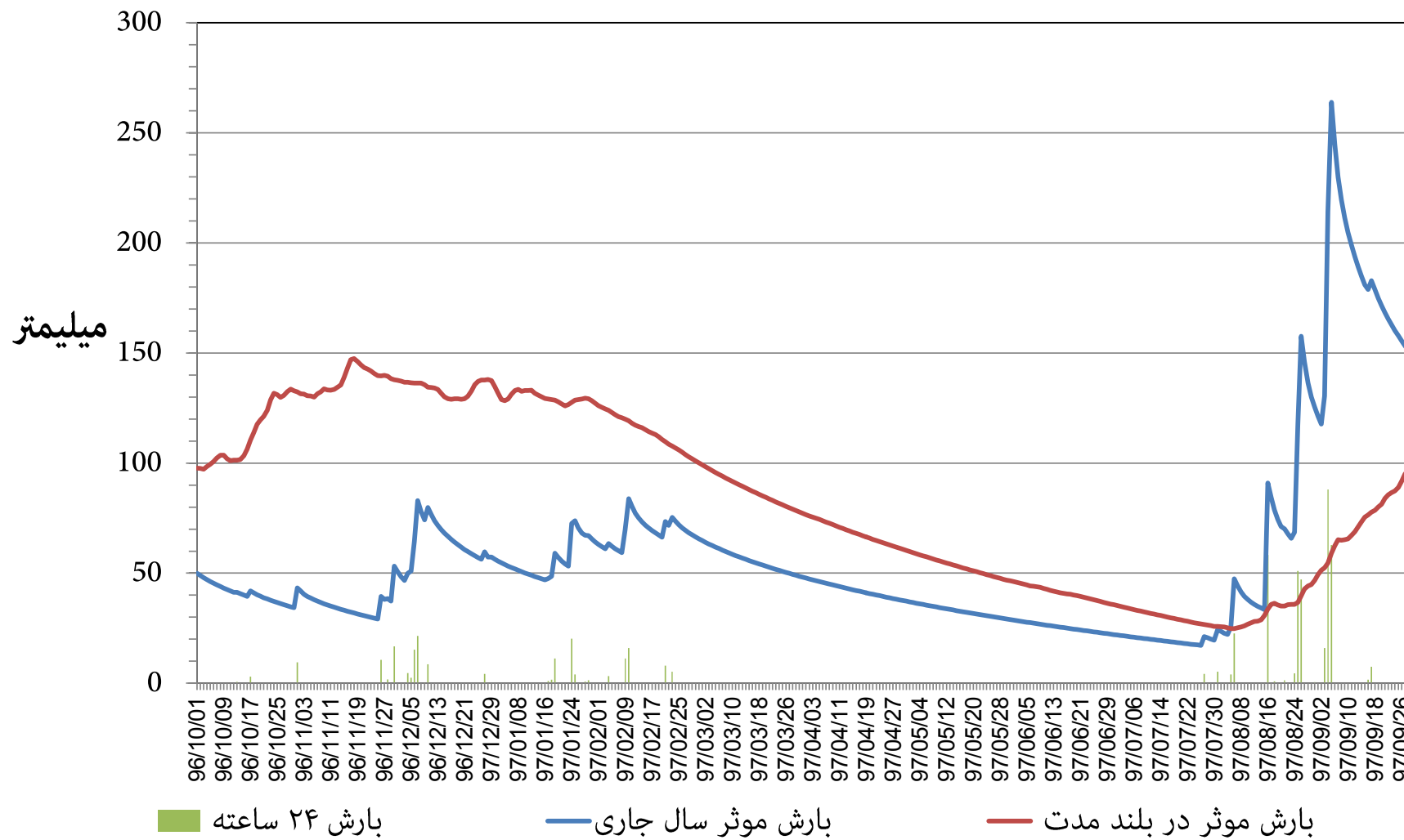
نمودار توزیع زمانی بارش و بارش موثر ۳۶۵ روزه ایستگاه باران سنجی ایدنک (وزارت نیرو) استان خوزستان دوره ۱۲ ماهه تا پایان آذر ماه ۱۳۹۷
