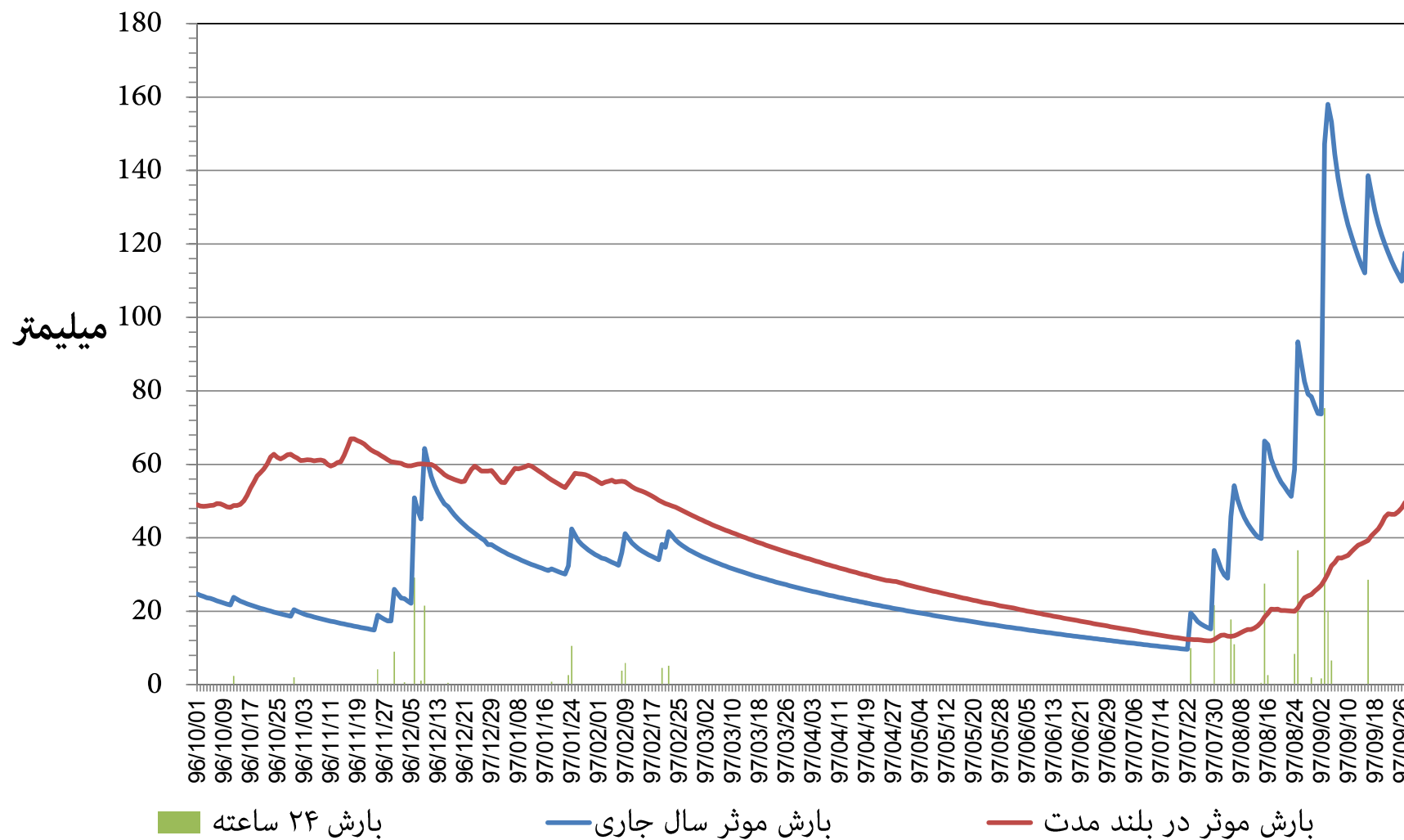
نمودار توزیع زمانی بارش و بارش موثر ۳۶۵ روزه ایستگاه هواشناسی آغاچاری استان خوزستان دوره ۱۲ ماهه تا پایان آذر ماه ۱۳۹۷
