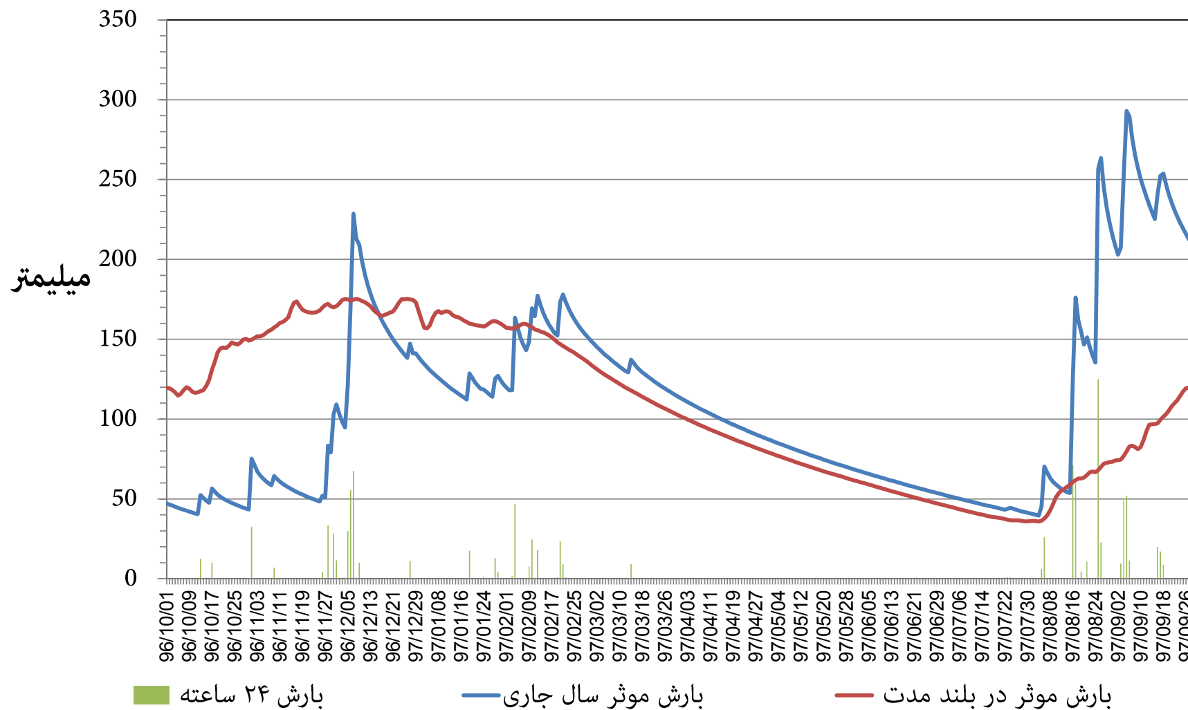
نمودار توزیع زمانی بارش و بارش موثر ۳۶۵ روزه ایستگاه باران سنجی تله زنگ (وزارت نیرو) استان خوزستان دوره ۱۲ ماهه تا پایان آذر ماه ۱۳۹۷
