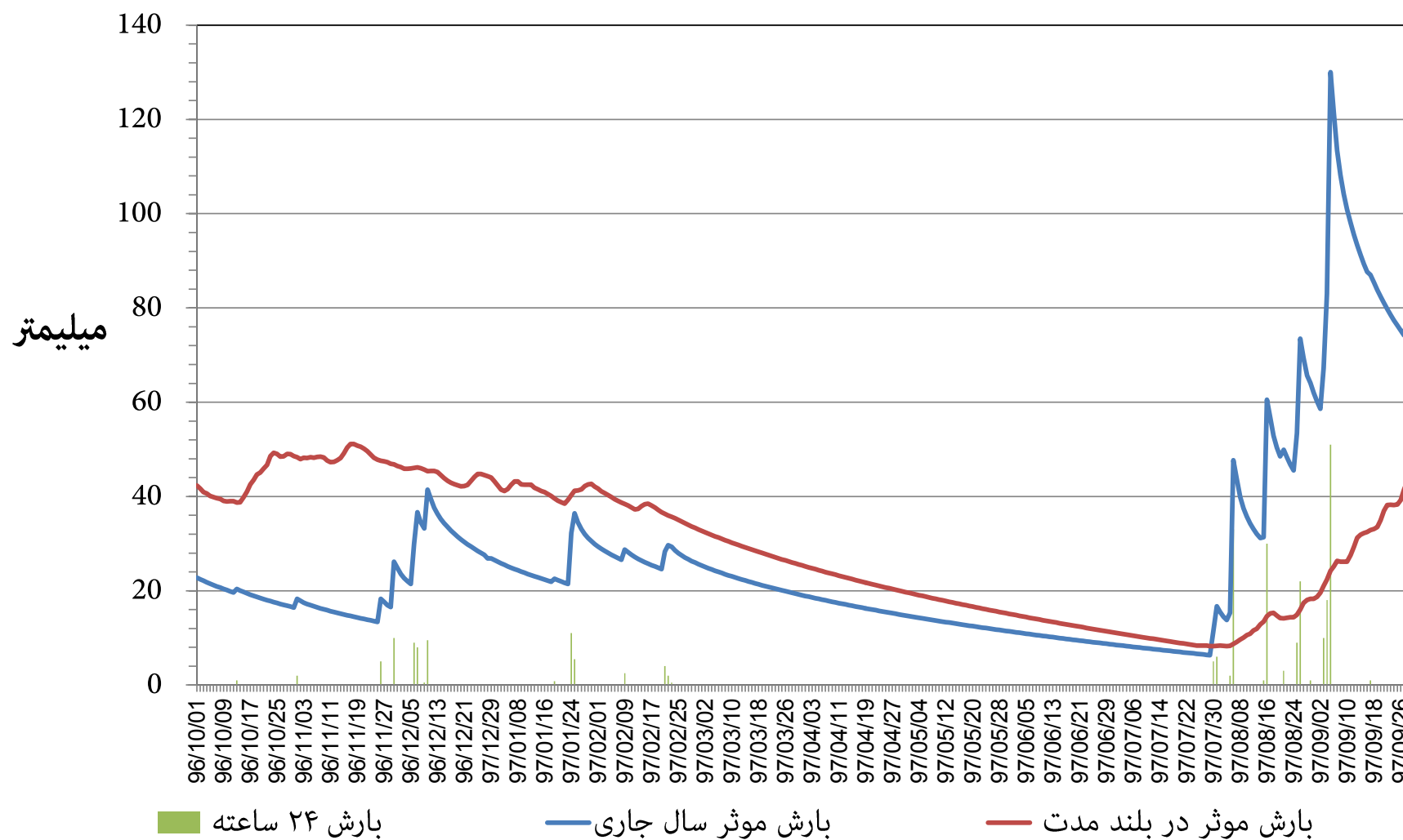
نمودار توزیع زمانی بارش و بارش موثر ۳۶۵ روزه ایستگاه باران سنجی مشراکه (وزارت نیرو) استان خوزستان دوره ۱۲ ماهه تا پایان آذر ماه ۱۳۹۷
