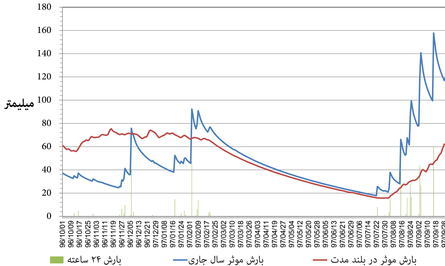
نمودار توزیع زمانی بارش و بارش موثر ۳۶۵ روزه ایستگاه هواشناسی صفی اباد (دزفول) استان خوزستان دوره ۱۲ ماهه تا پایان آذر ماه ۱۳۹۷
