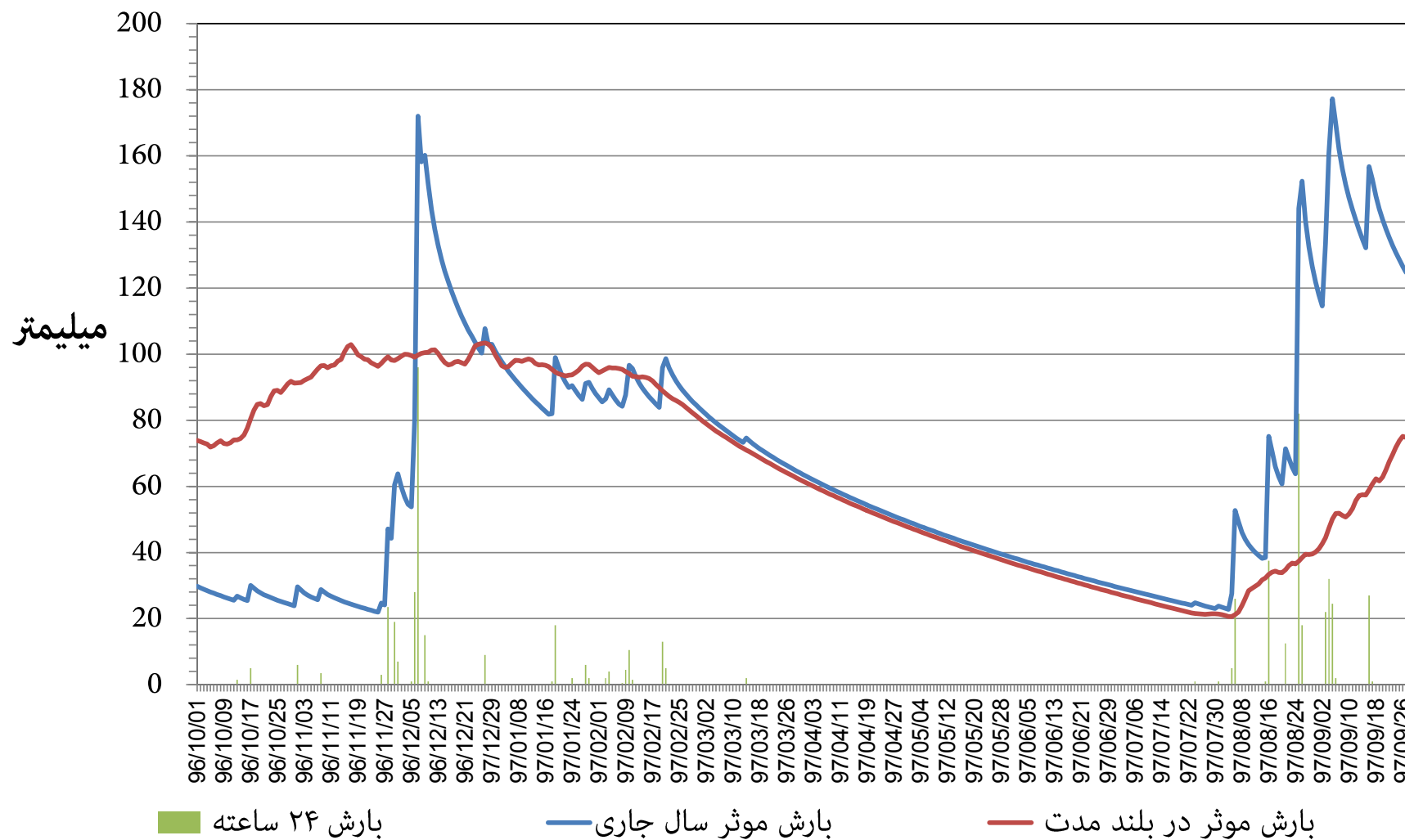
نمودار توزیع زمانی بارش و بارش موثر ۳۶۵ روزه ایستگاه باران سنجی سد دز (وزارت نیرو) استان خوزستان دوره ۱۲ ماهه تا پایان آذر ماه ۱۳۹۷
