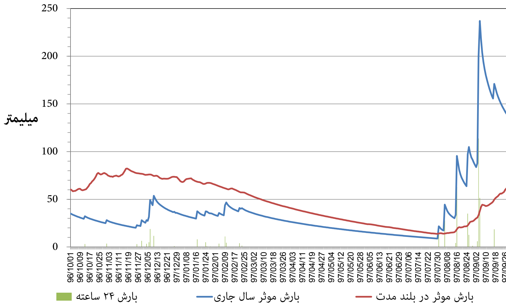
نمودار توزیع زمانی بارش و بارش موثر ۳۶۵ روزه ایستگاه باران سنجی سد شهدا (وزارت نیرو) استان خوزستان دوره ۱۲ ماهه تا پایان آذر ماه ۱۳۹۷
