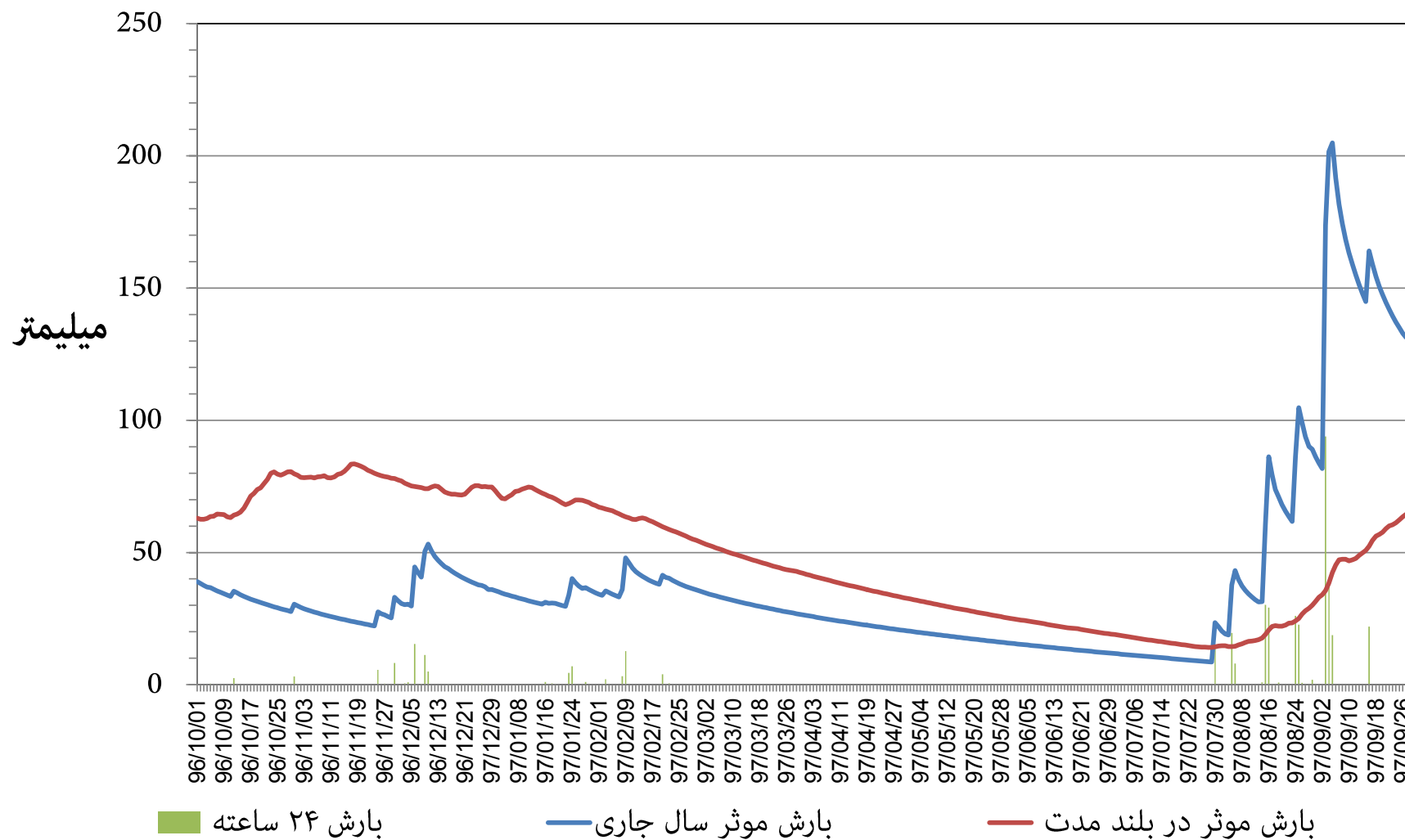
مقدار توزیع زمانی بارش و بارش موثر ۳۶۵ روزه ایستگاه هواشناسی بهبهان استان خوزستان دوره ۱۲ ماهه تا پایان آذر ماه ۱۳۹۷
