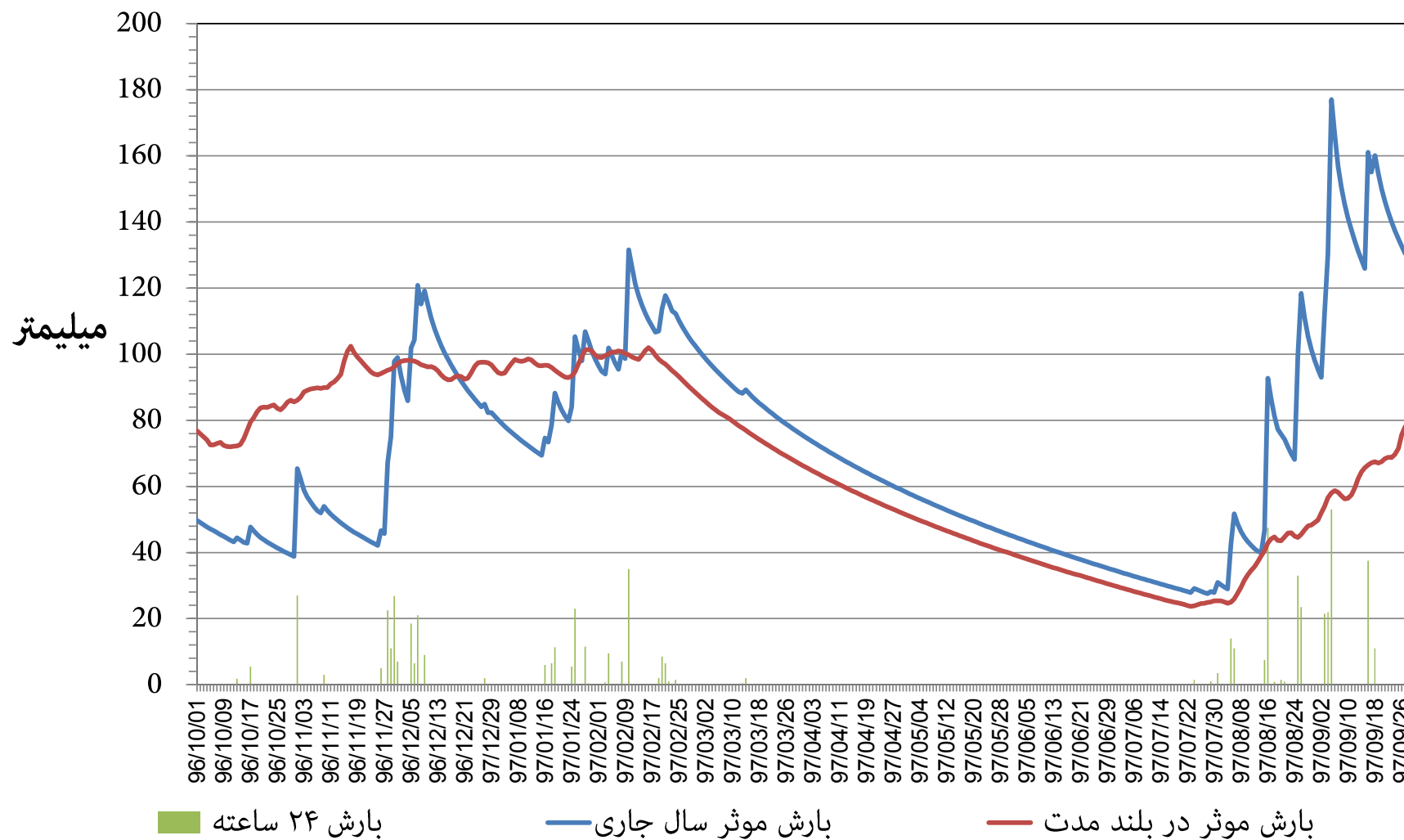
نمودار توزیع زمانی بارش و بارش موثر ۳۶۵ روزه ایستگاه باران سنجی چم گز (وزارت نیرو) استان خوزستان دوره ۱۲ ماهه تا پایان آذر ماه ۱۳۹۷
