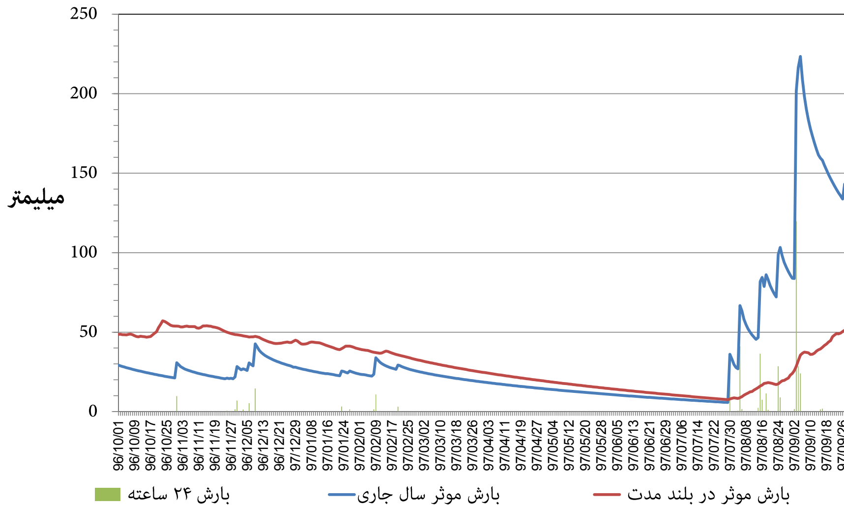
نمودار توزیع زمانی بارش و بارش موثر ۳۶۵ روزه ایستگاه هواشناسی هندیجان استان خوزستان دوره ۱۲ ماهه تا پایان آذر ماه ۱۳۹۷
