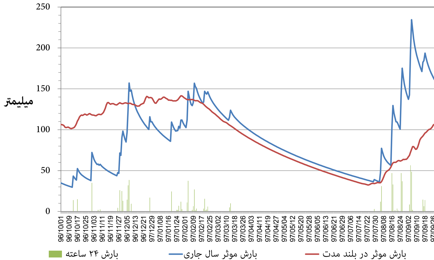
نمودار توزیع زمانی بارش و بارش موثر ۳۶۵ روزه ایستگاه باران سنجی سپیددشت (وزارت نیرو) استان خوزستان دوره ۱۲ ماهه تا پایان آذر ماه ۱۳۹۷
