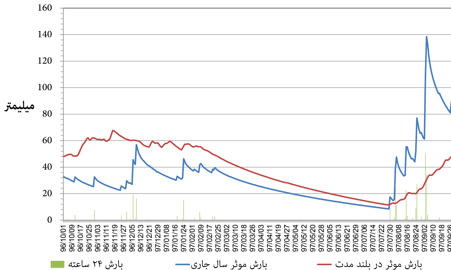
نمودار توزیع زمانی بارش و بارش موثر ۳۶۵ روزه ایستگاه هواشناسی امیدیه (آغاچاری) استان خوزستان دوره ۱۲ ماهه تا پایان آذر ماه ۱۳۹۷
