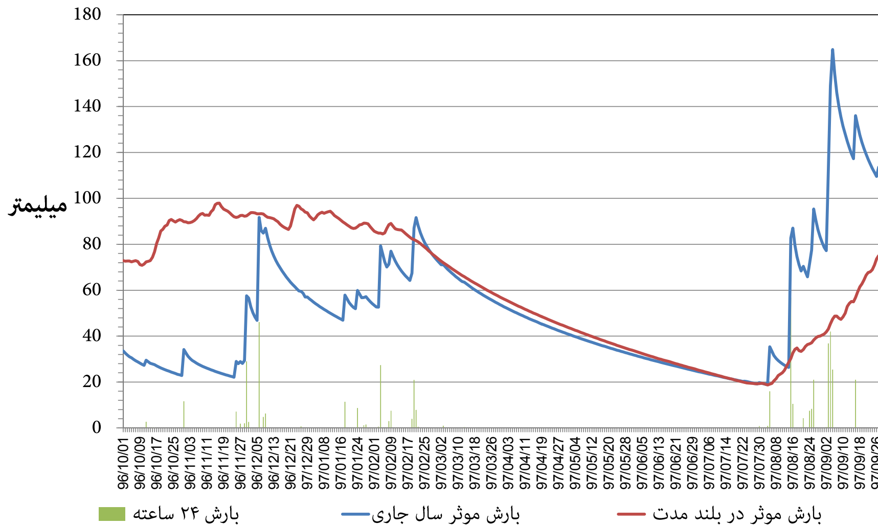
نمودار توزیع زمانی بارش و بارش موثر ۳۶۵ روزه ایستگاه هواشناسی مسجد سلیمان استان خوزستان دوره ۱۲ ماهه تا پایان آذر ماه ۱۳۹۷
