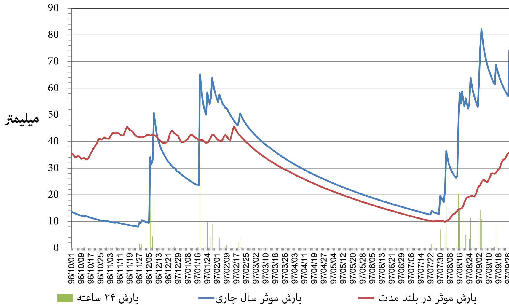
نمودار توزیع زمانی بارش و بارش موثر ۳۶۵ روزه ایستگاه هواشناسی بستان استان خوزستان دوره ۱۲ ماهه تا پایان آذر ماه ۱۳۹۷
