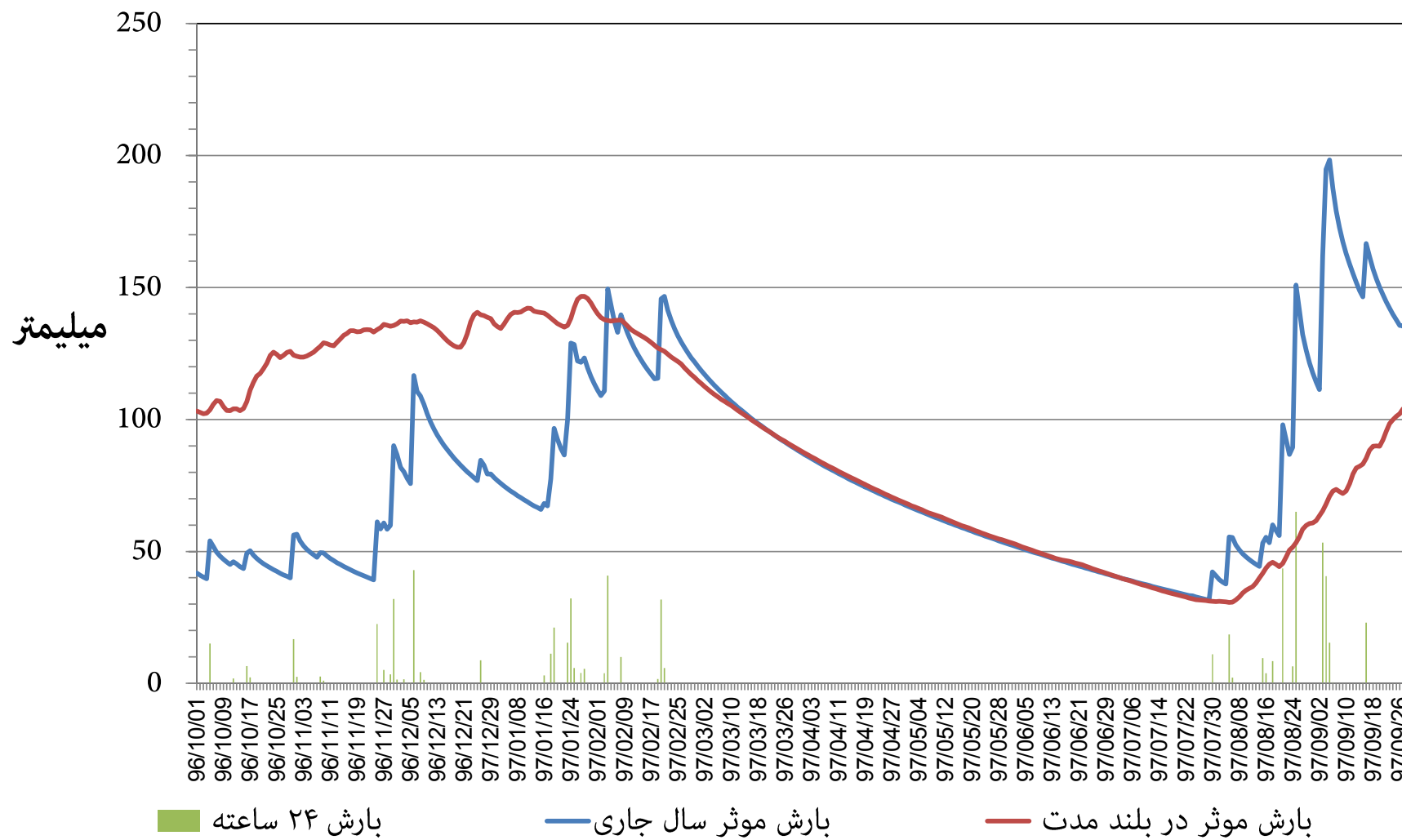
نمودار توزیع زمانی بارش و بارش موثر ۳۶۵ روزه ایستگاه هواشناسی ایذه استان خوزستان دوره ۱۲ ماهه تا پایان آذر ماه ۱۳۹۷
