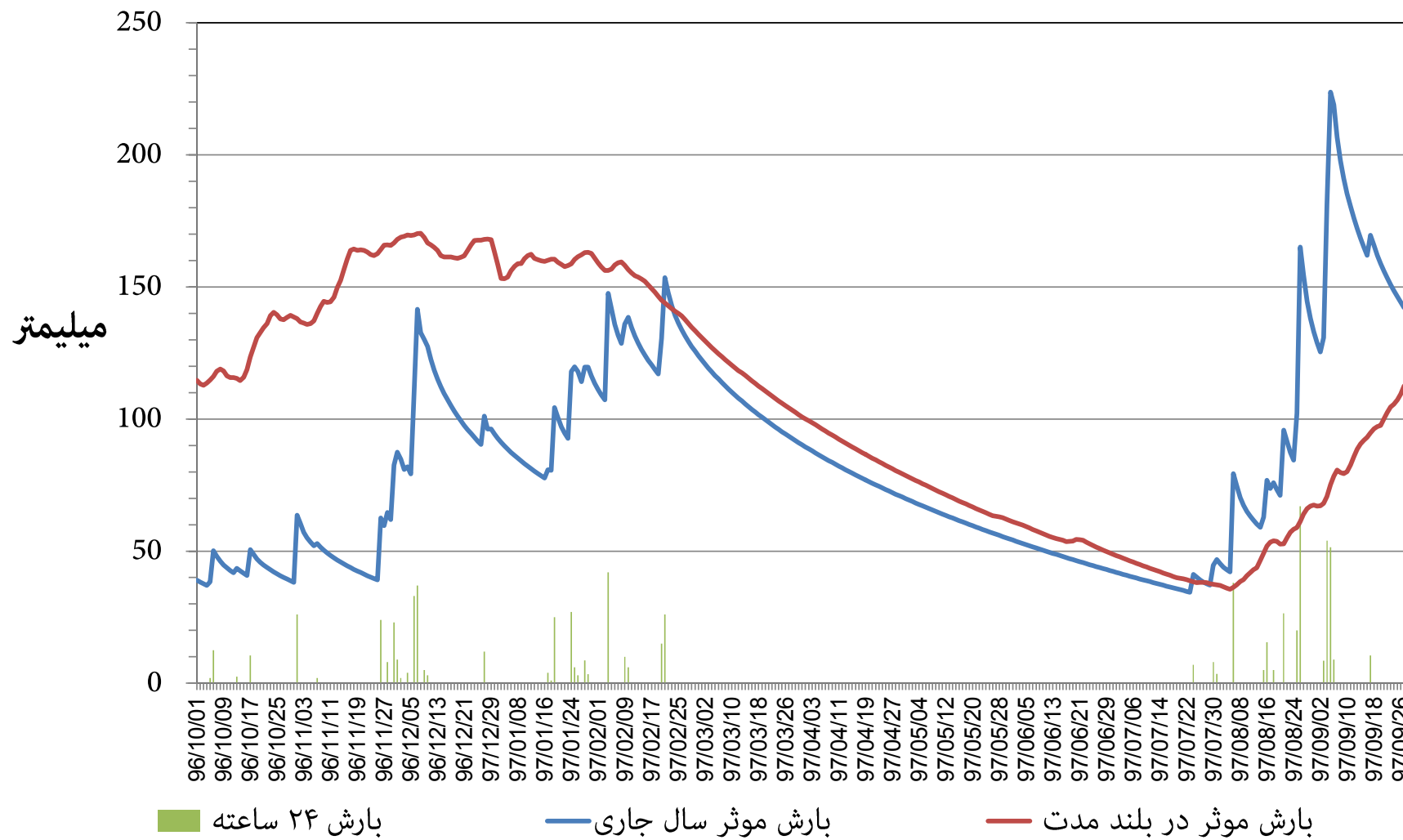
نمودار توزیع زمانی بارش و بارش موثر ۳۶۵ روزه ایستگاه باران سنجی کارون سه (وزارت نیرو) استان خوزستان دوره ۱۲ ماهه تا پایان آذر ماه ۱۳۹۷
