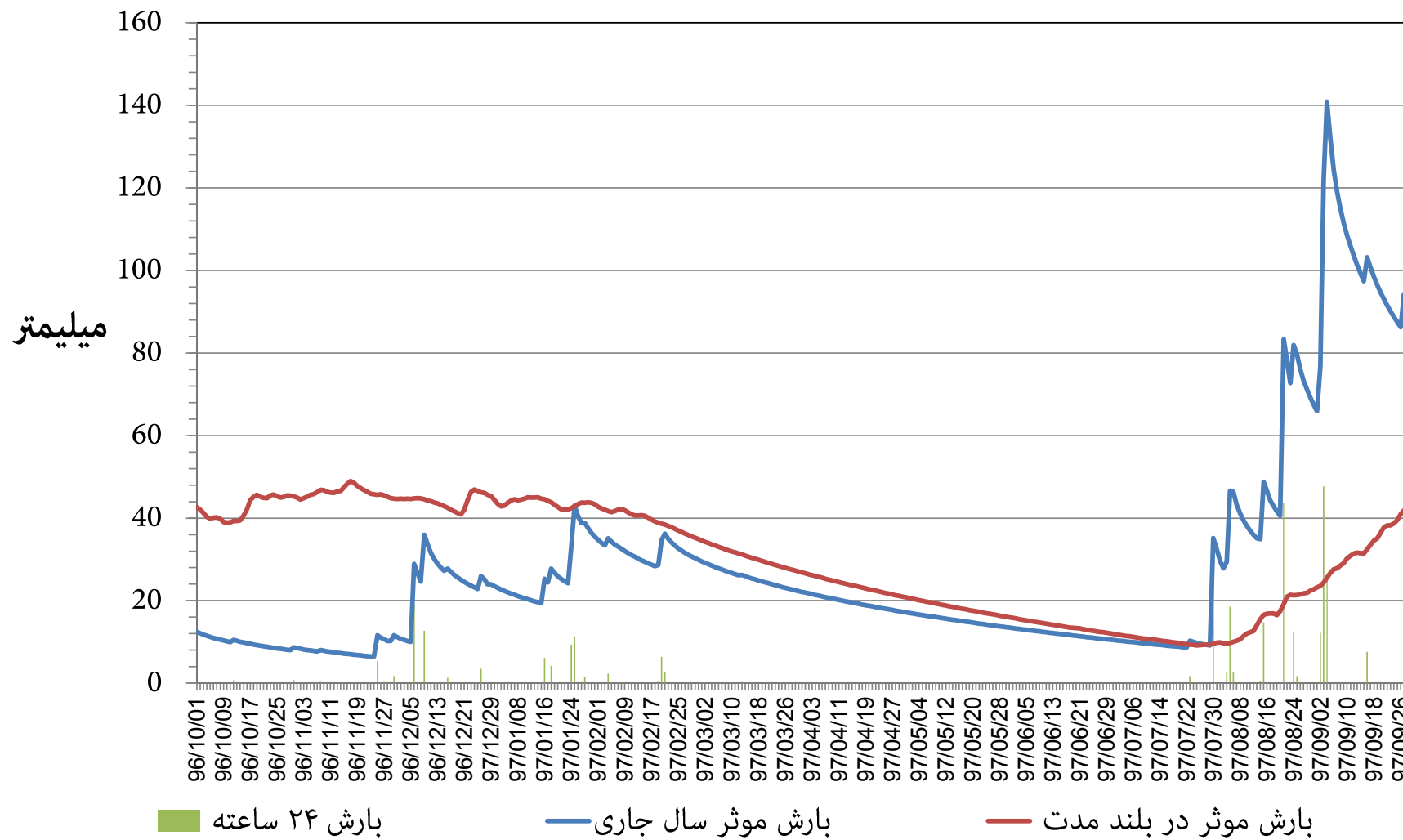
نمودار توزیع زمانی بارش و بارش موثر ۳۶۵ روزه ایستگاه هواشناسی اهواز استان خوزستان دوره ۱۲ ماهه تا پایان آذر ماه ۱۳۹۷
