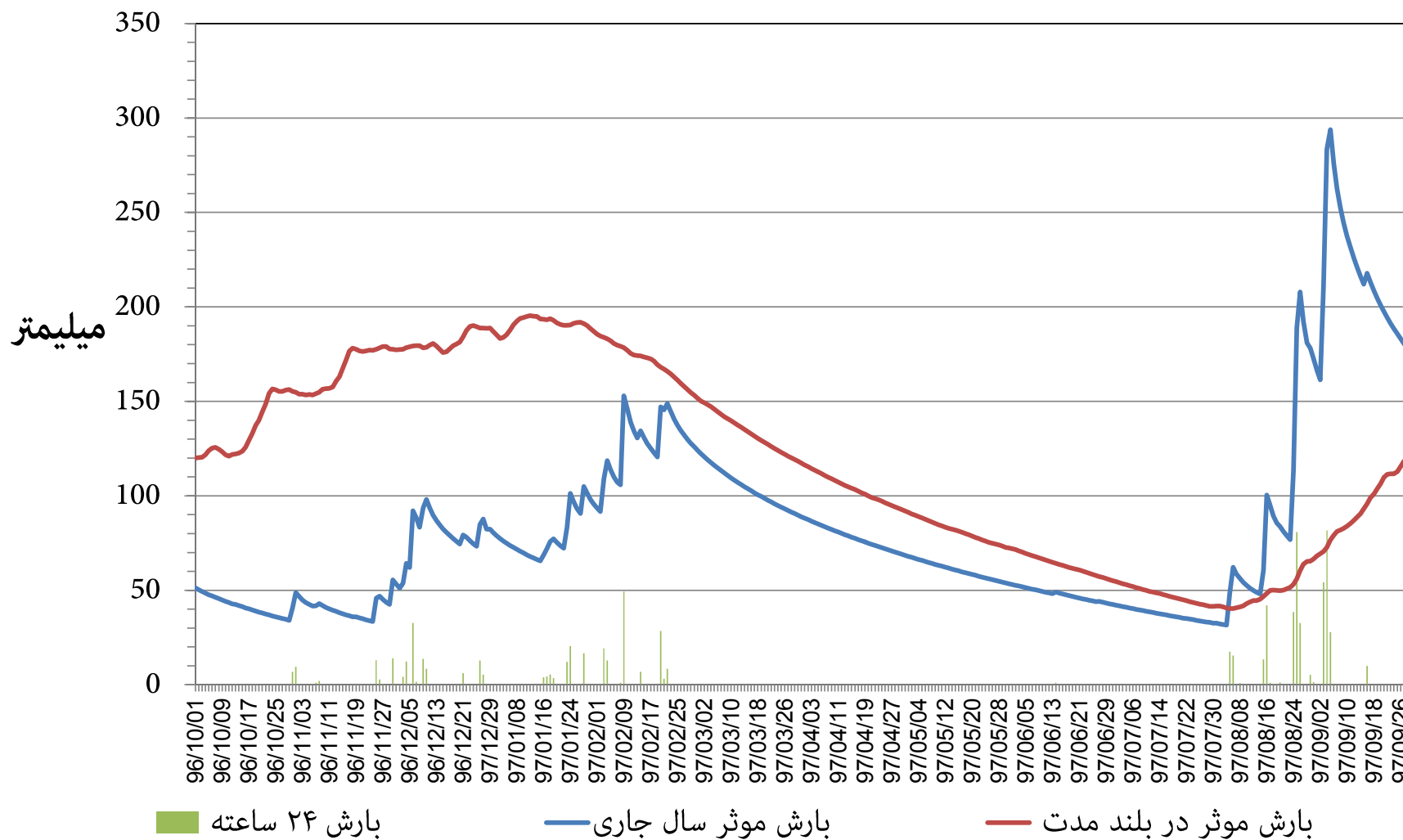
نمودار توزیع زمانی بارش و بارش موثر ۳۶۵ روزه ایستگاه هواشناسی یاسوج استان کهگیلویه و بویراحمد دوره ۱۲ ماهه تا پایان آذر ماه ۱۳۹۷
