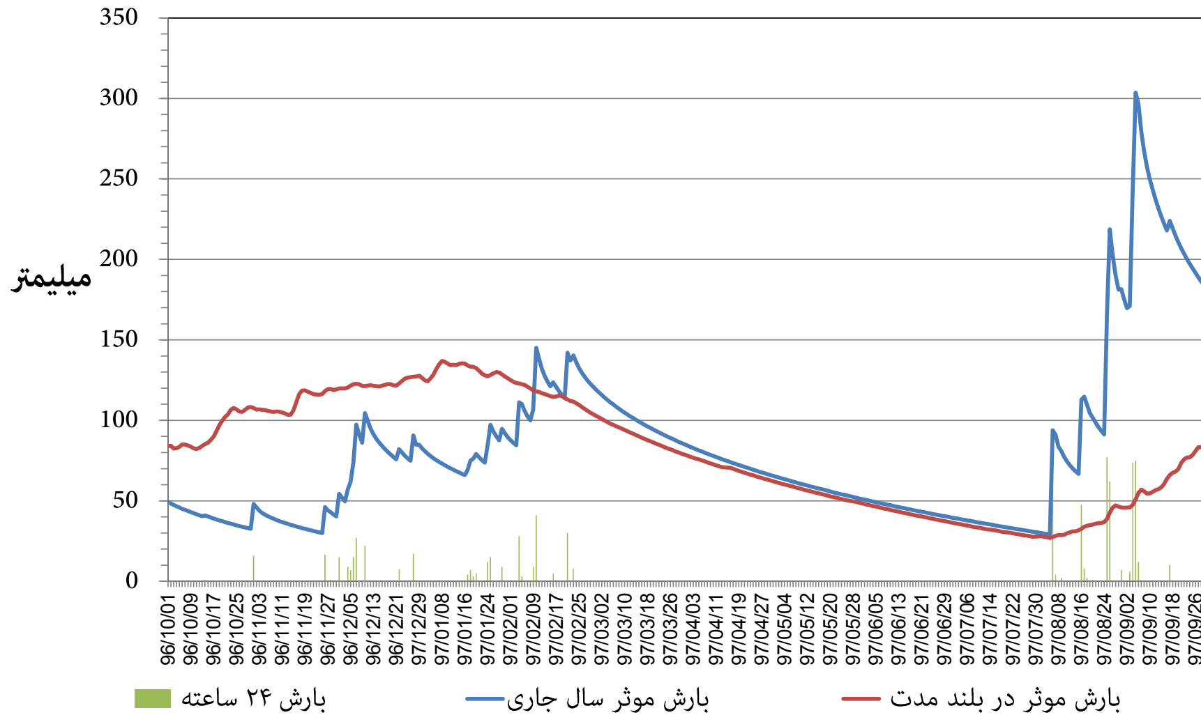
نمودار توزیع زمانی بارش و بارش موثر ۳۶۵ روزه ایستگاه باران سنجی یاسوج (وزارت نیرو) استان کهگیلویه و بویراحمد دوره ۱۲ ماهه تا پایان آذر ماه ۱۳۹۷
