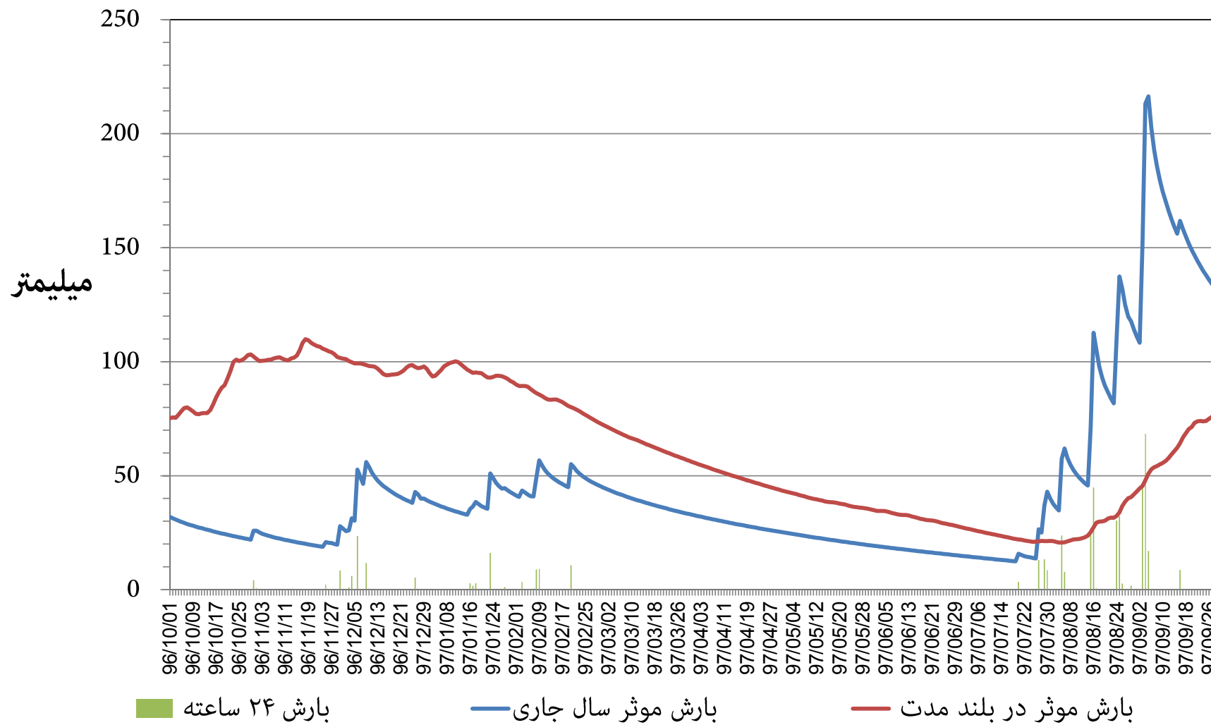
نمودار توزیع زمانی بارش و بارش موثر ۳۶۵ روزه ایستگاه هواشناسی دو گنبدان استان کهگیلویه و بویراحمد دوره ۱۲ ماهه تا پایان آذر ماه ۱۳۹۷
