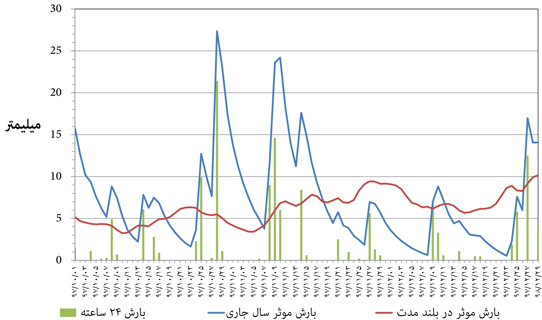
نمودار توزیع زمانی بارش و بارش موثر ۱۴ روزه ایستگاه هواشناسی معلم کلايه استان قزوین فصل زمستان ۱۳۹۷
