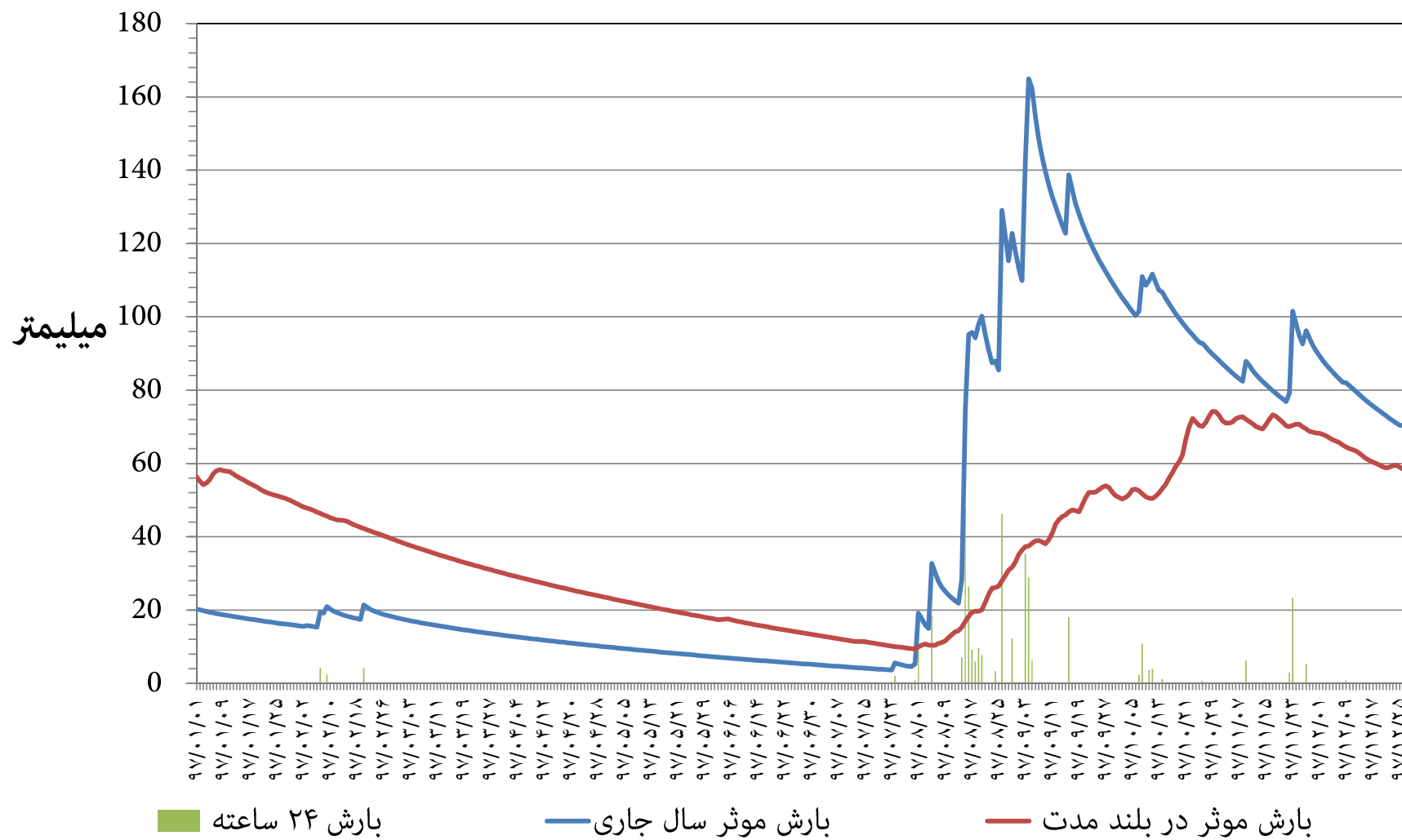
نمودار توزیع زمانی بارش و بارش موثر ۳۶۵ روزه ایستگاه هواشناسی فرودگاه بوشهر استان بوشهر سال شمسی ۱۳۹۷
