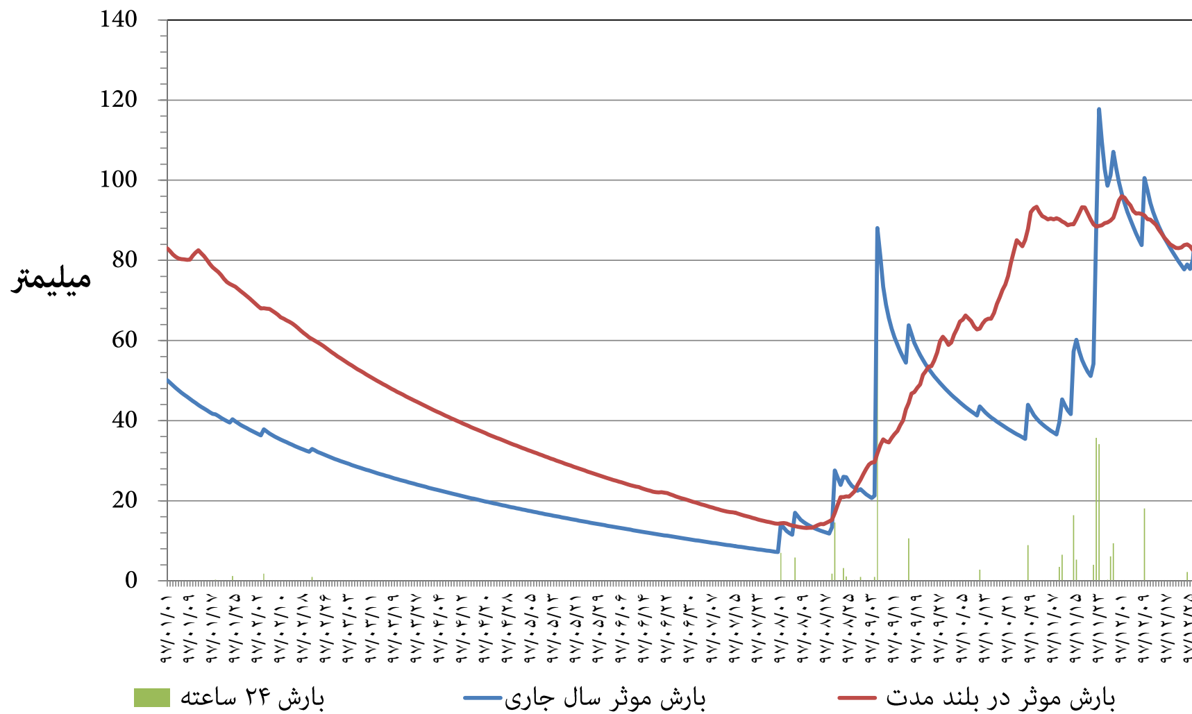
نمودار توزیع زمانی بارش و بارش موثر ۳۶۵ روزه ایستگاه هواشناسی جم استان بوشهر سال شمسی ۱۳۹۷
