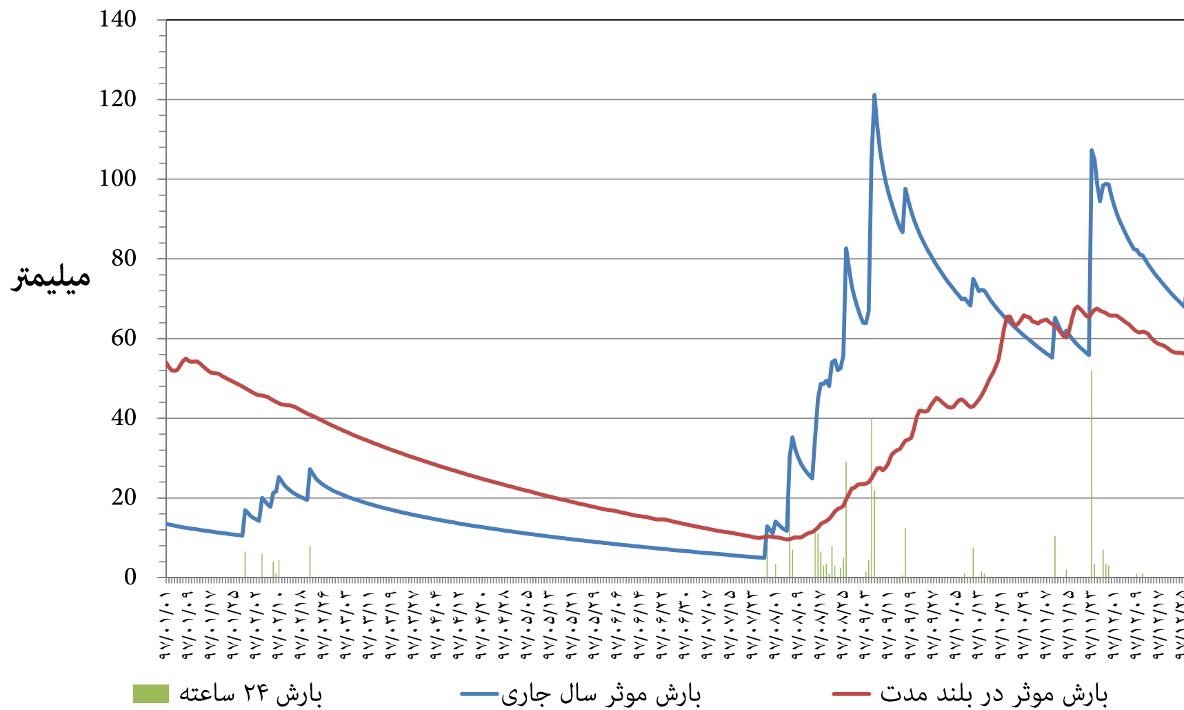
نمودار توزیع زمانی بارش و بارش موثر ۳۶۵ روزه ایستگاه باران سنجی سعد آباد (وزارت نیرو) استان بوشهر سال شمسی ۱۳۹۷
