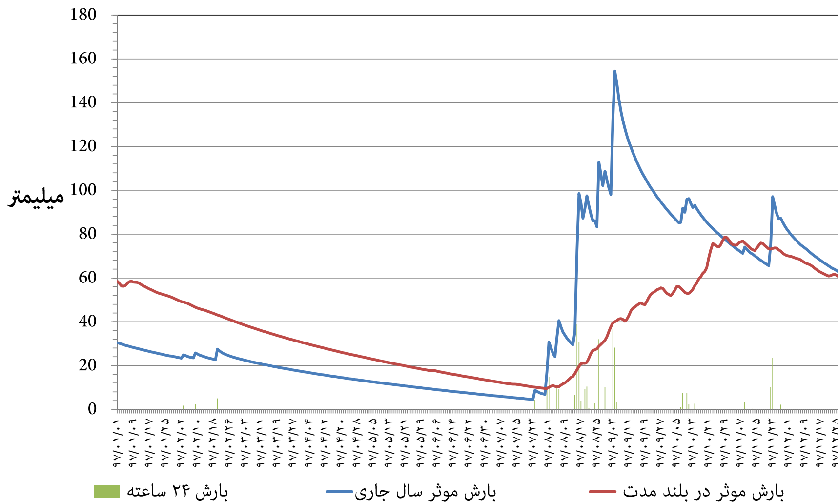
نمودار توزیع زمانی بارش و بارش موثر ۳۶۵ روزه ایستگاه هواشناسی بوشهر (ساحلی) استان بوشهر سال شمسی ۱۳۹۷
