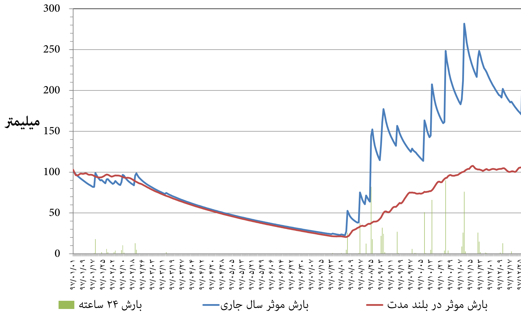
نمودار توزیع زمانی بارش و بارش موثر ۳۶۵ روزه ایستگاه باران سنجی سد دز (وزارت نیرو) استان خوزستان سال شمسی ۱۳۹۷
