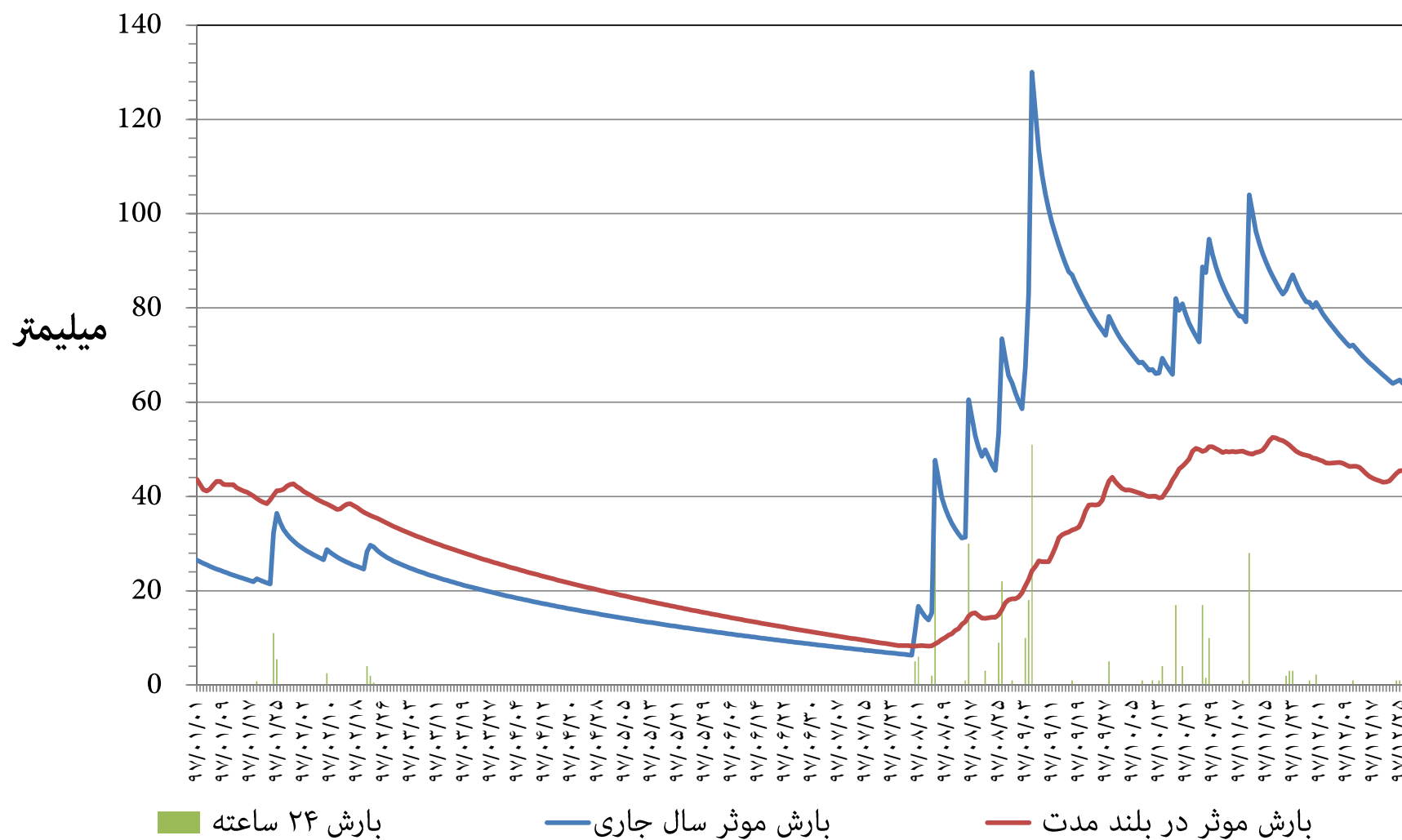
نمودار توزیع زمانی بارش و بارش موثر ۳۶۵ روزه ایستگاه باران سنجی مشراکه (وزارت نیرو) استان خوزستان سال شمسی ۱۳۹۷
