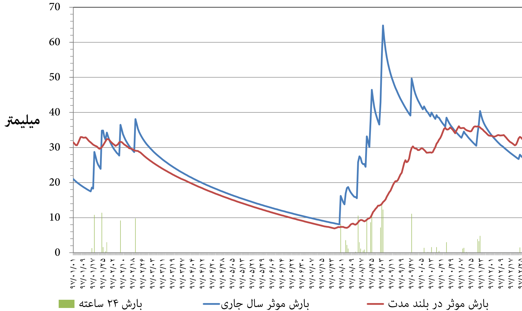
نمودار توزیع زمانی بارش و بارش موثر ۳۶۵ روزه ایستگاه هواشناسی آبادان استان خوزستان سال شمسی ۱۳۹۷
