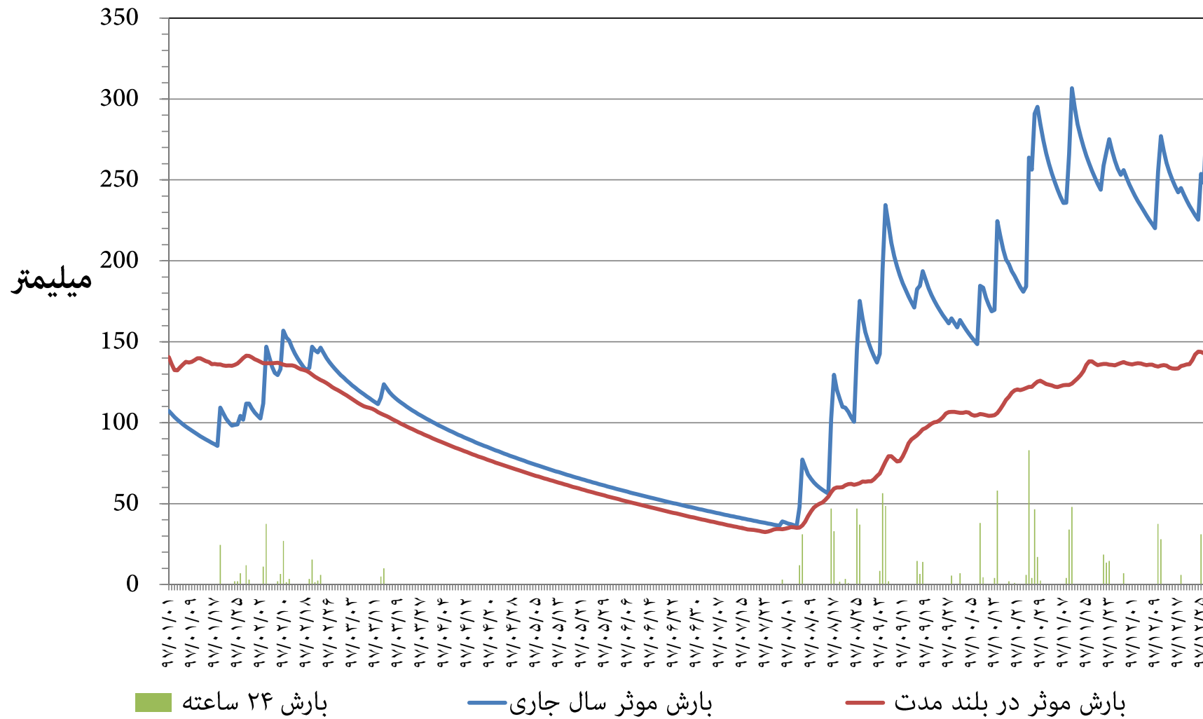
نمودار توزیع زمانی بارش و بارش موثر ۳۶۵ روزه ایستگاه باران سنجی سپیددشت (وزارت نیرو) استان خوزستان سال شمسی ۱۳۹۷
