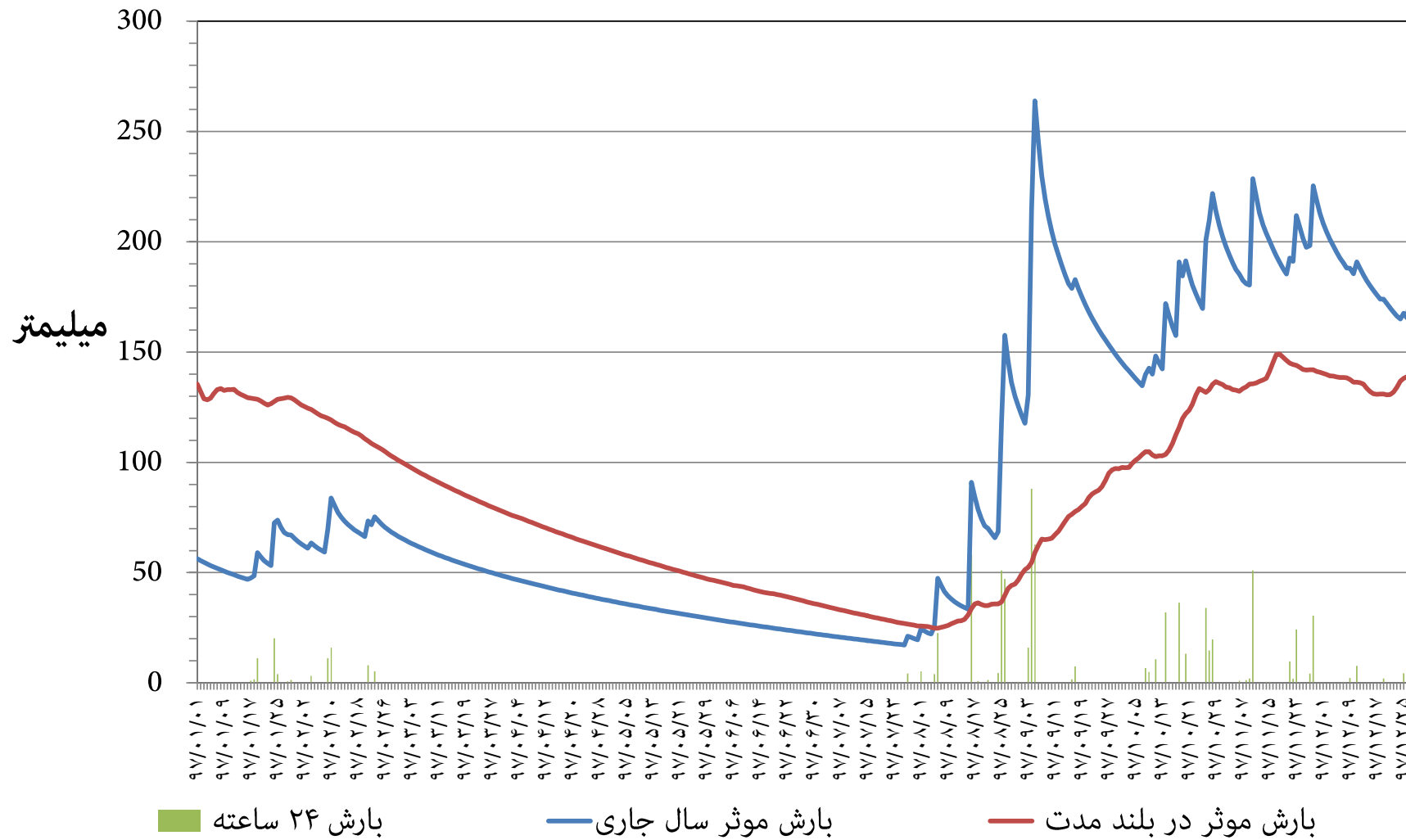
نمودار توزیع زمانی بارش و بارش موثر ۳۶۵ روزه ایستگاه باران سنجی ایدنک (وزارت نیرو) استان خوزستان سال شمسی ۱۳۹۷
