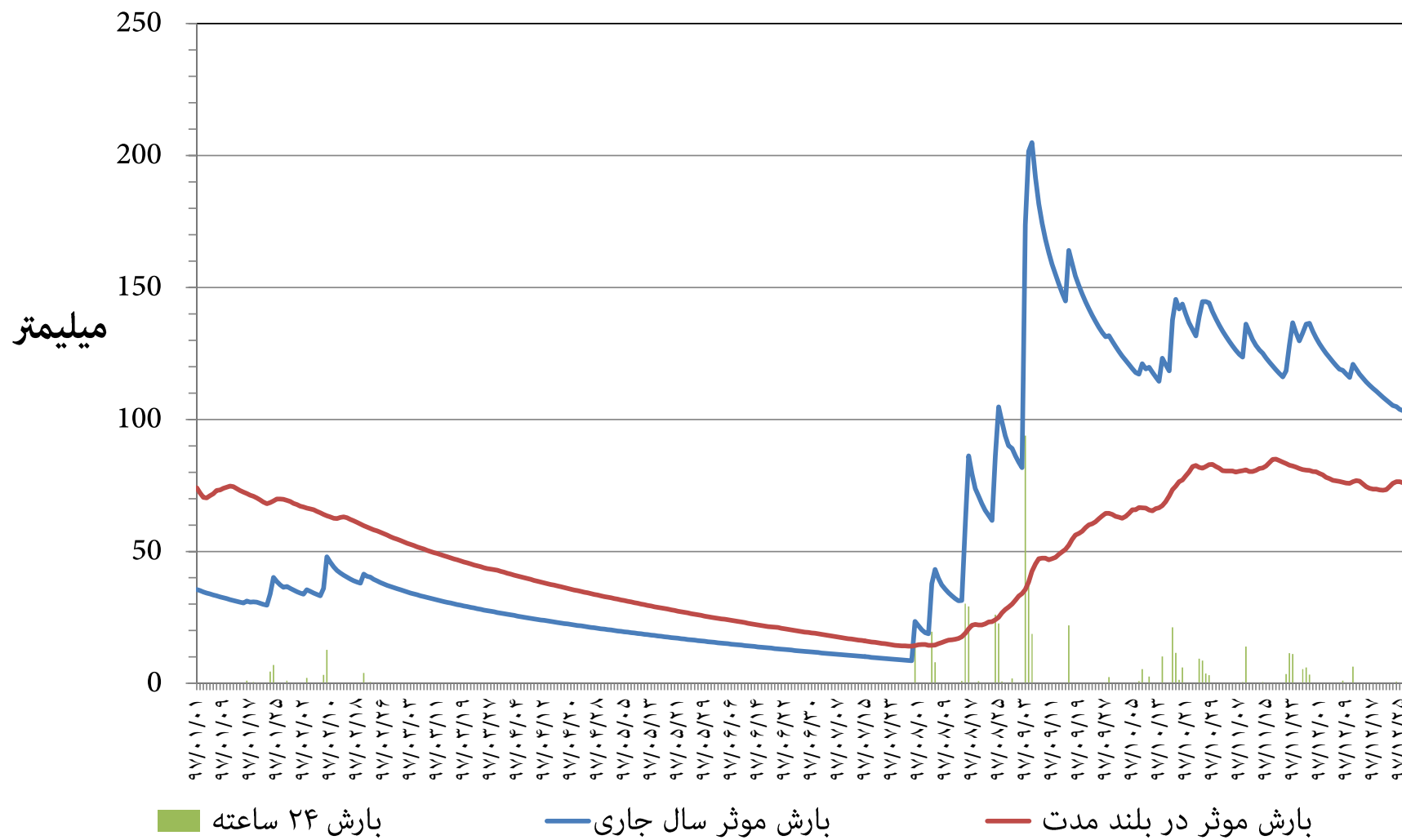
نمودار توزیع زمانی بارش و بارش موثر ۳۶۵ روزه ایستگاه هواشناسی بهبهان استان خوزستان سال شمسی ۱۳۹۷
