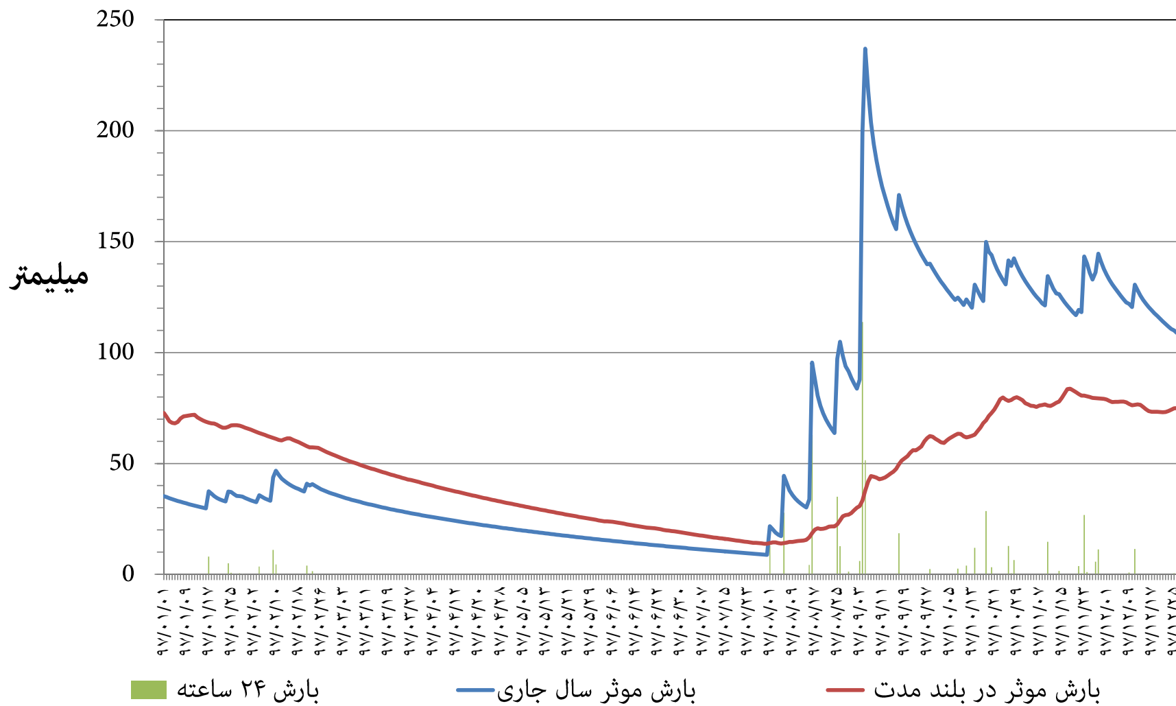
مردار توزیع زمانی بارش و بارش موثر ۳۶۵ روزه ایستگاه باران سنجی سد شهدا (وزارت نیرو) استان خوزستان سال شمسی ۱۳۹۷
