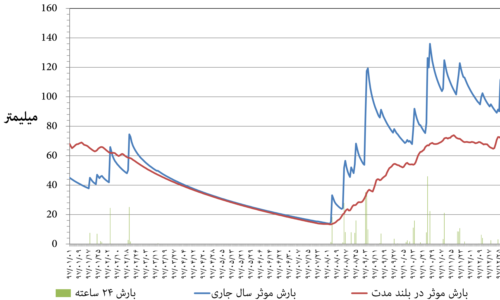
مقدار توزیع زمانی بارش و بارش موثر ۳۶۵ روزه ایستگاه هواشناسی شوشتر استان خوزستان سال شمسی ۱۳۹۷
