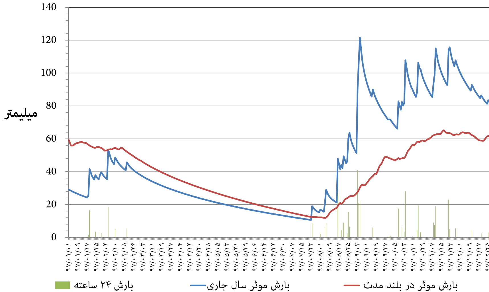
نمودار توزیع زمانی بارش و بارش موثر ۳۶۵ روزه ایستگاه باران سنجی هفت تپه (وزارت نیرو) استان خوزستان سال شمسی ۱۳۹۷
