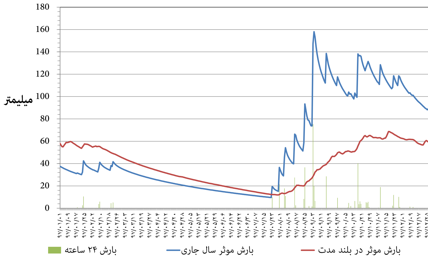
نمودار توزیع زمانی بارش و بارش موثر ۳۶۵ روزه ایستگاه هواشناسی آغاچاری استان خوزستان سال شمسی ۱۳۹۷
