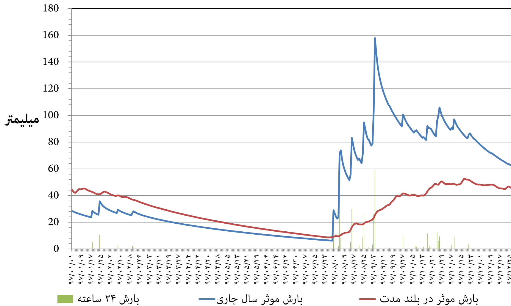
نمودار توزیع زمانی بارش و بارش موثر ۳۶۵ روزه ایستگاه هواشناسی بندر ماهشهر استان خوزستان سال شمسی ۱۳۹۷
