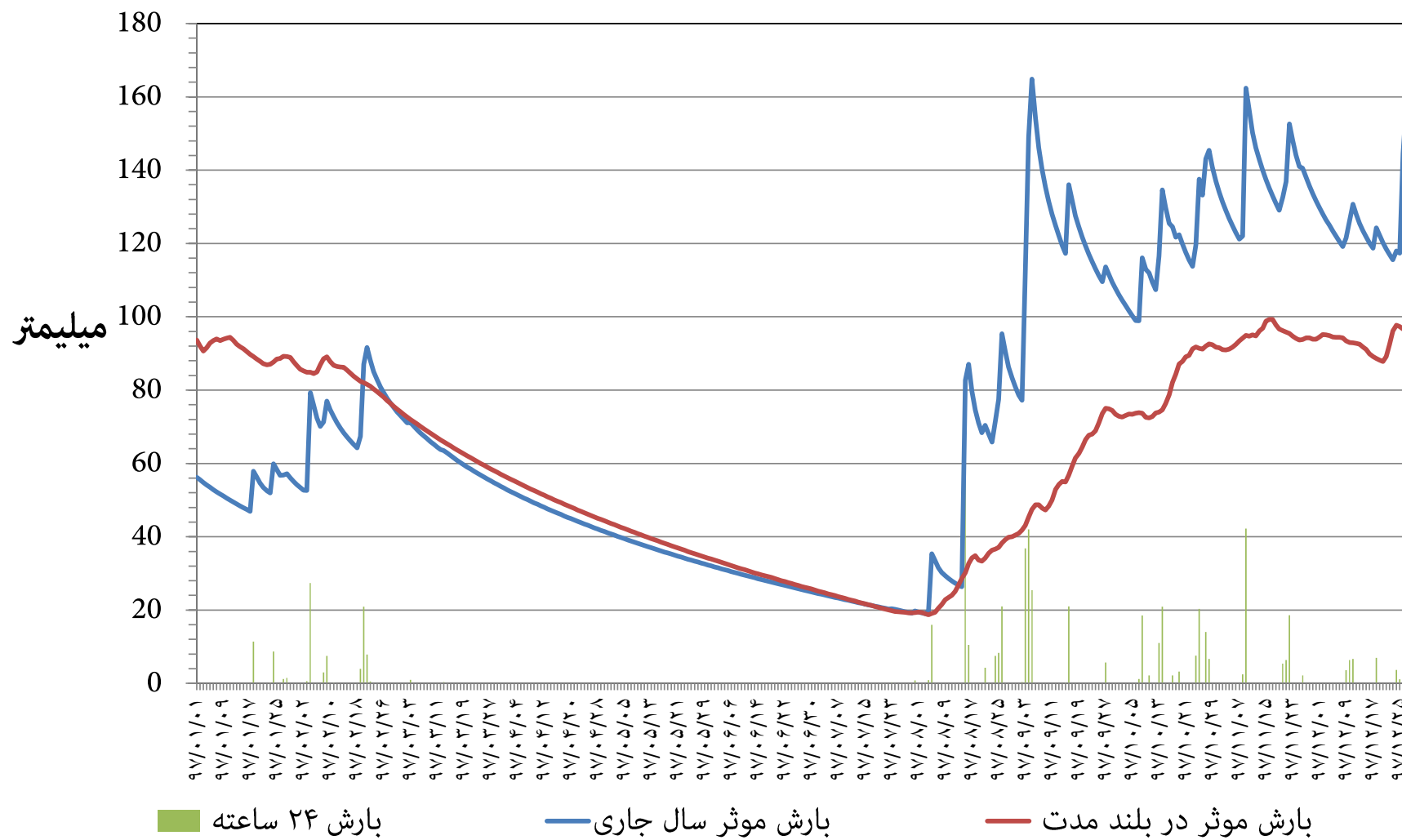
نمودار توزیع زمانی بارش و بارش موثر ۳۶۵ روزه ایستگاه هواشناسی مسجد سلیمان استان خوزستان سال شمسی ۱۳۹۷
