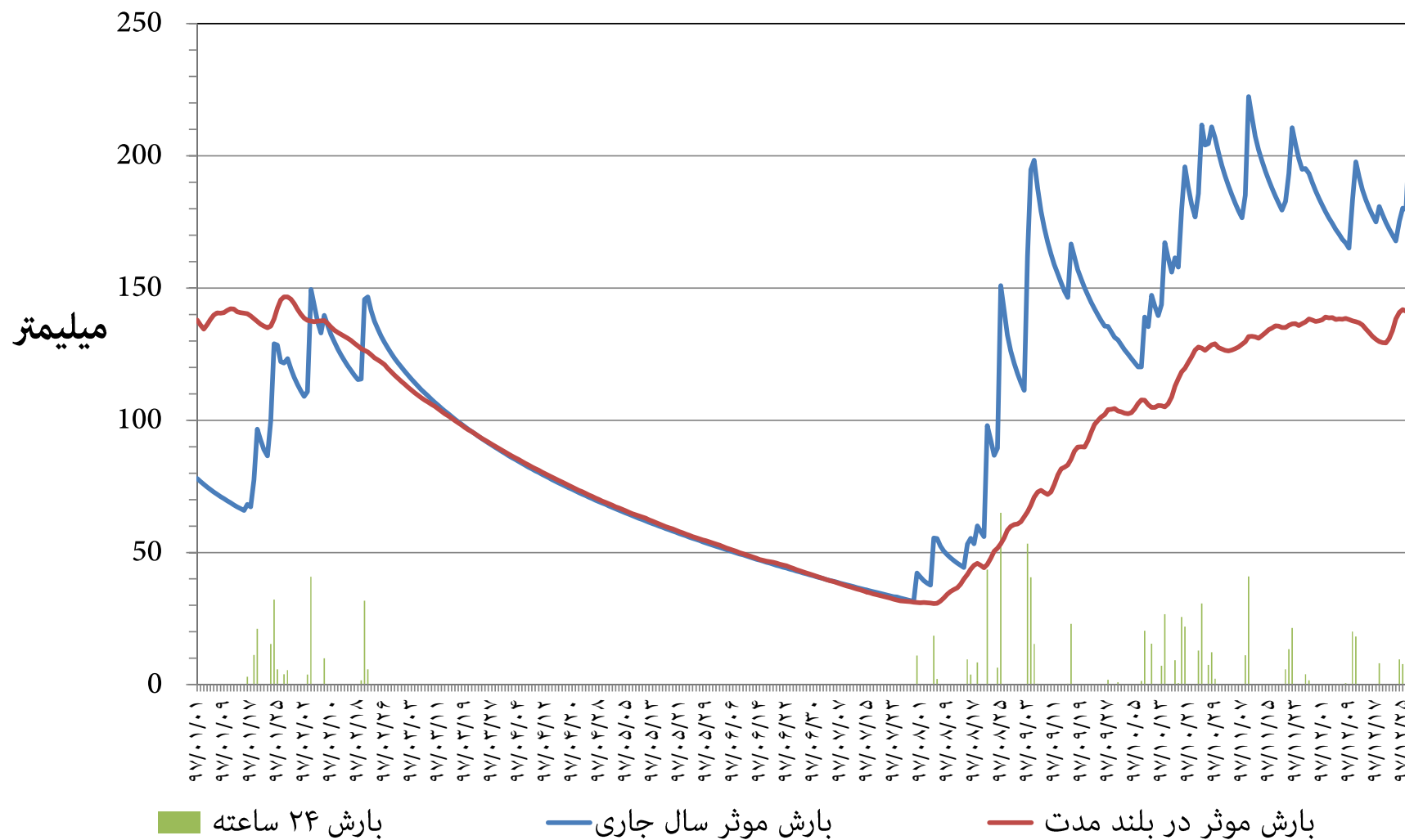
نمودار توزیع زمانی بارش و بارش موثر ۳۶۵ روزه ایستگاه هواشناسی ایذه استان خوزستان سال شمسی ۱۳۹۷
