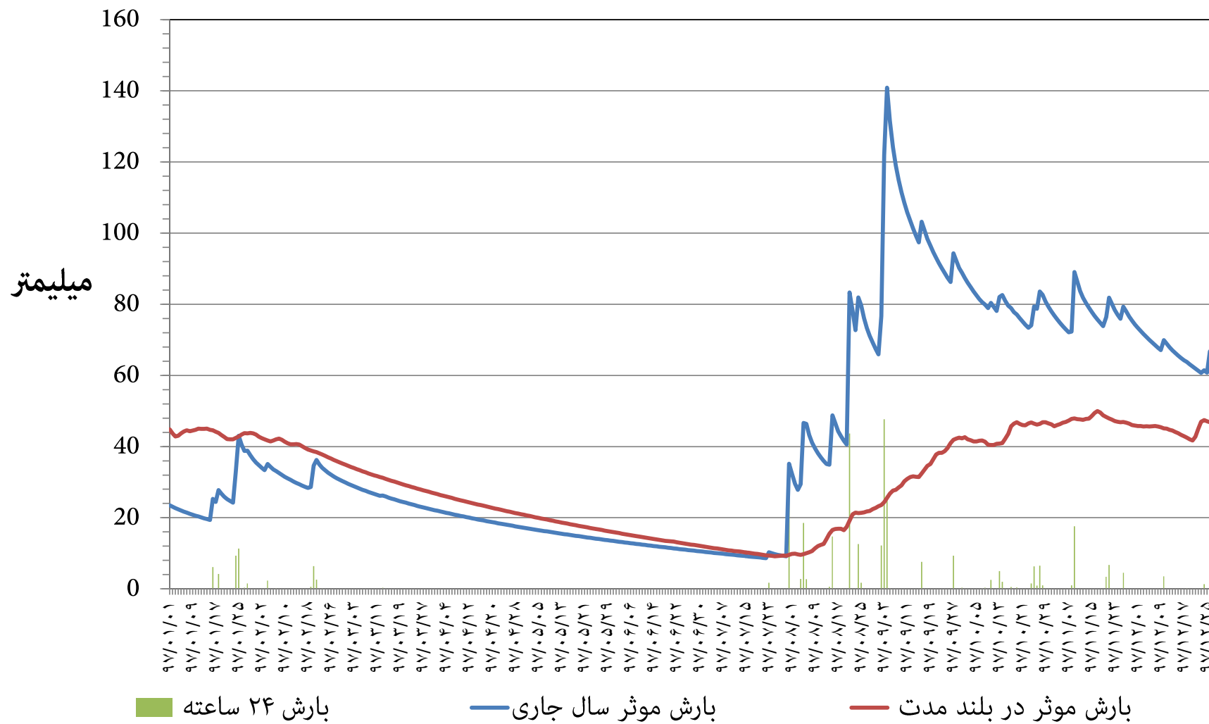
نمودار توزیع زمانی بارش و بارش موثر ۳۶۵ روزه ایستگاه هواشناسی اهواز استان خوزستان سال شمسی ۱۳۹۷
