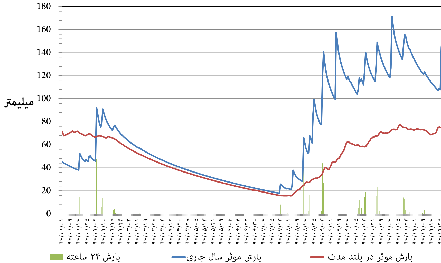
نمودار توزیع زمانی بارش و بارش موثر ۳۶۵ روزه ایستگاه هواشناسی صفی اباد (دزفول) استان خوزستان سال شمسی ۱۳۹۷
