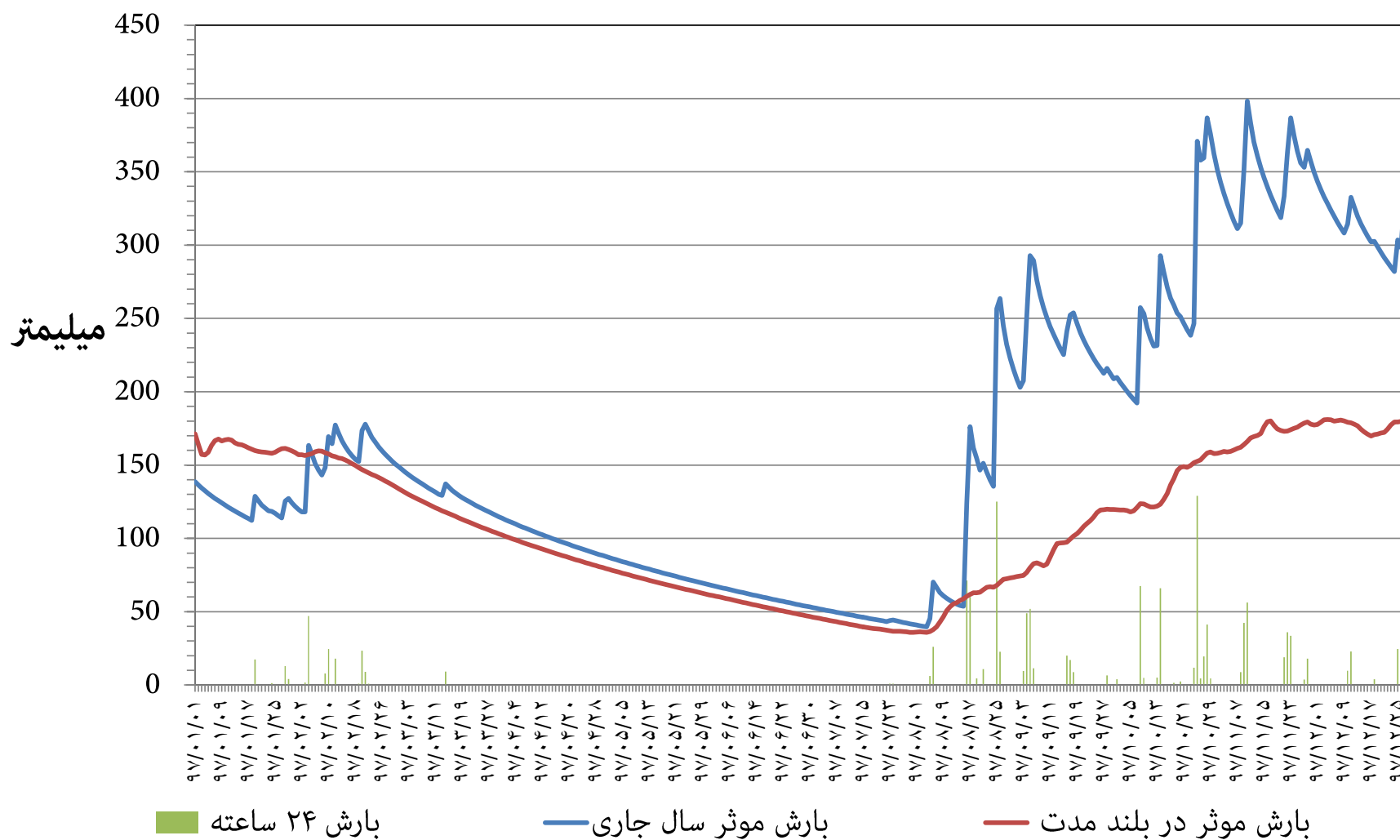
نمودار توزیع زمانی بارش و بارش موثر ۳۶۵ روزه ایستگاه باران سنجی تله زنگ (وزارت نیرو) استان خوزستان سال شمسی ۱۳۹۷
