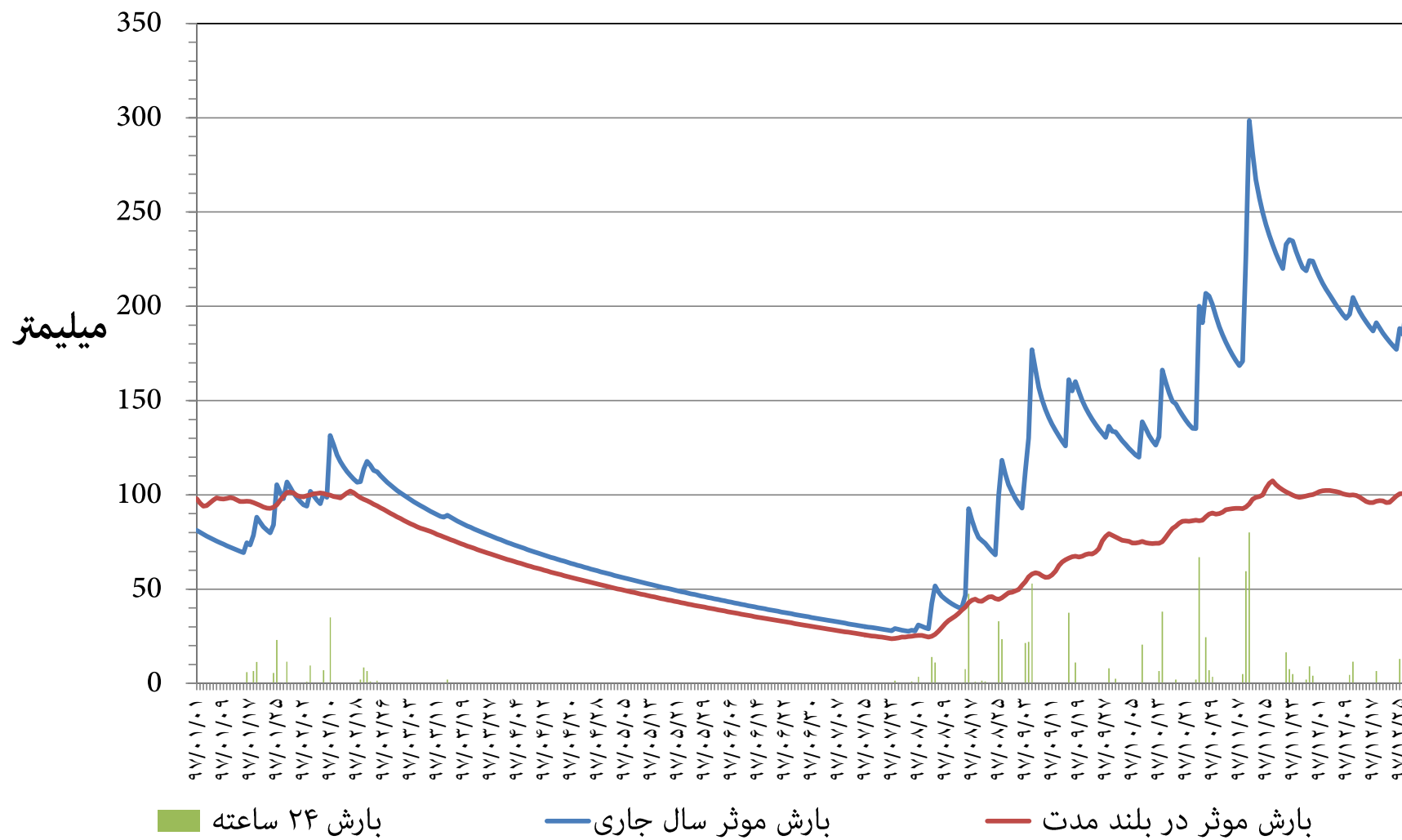
نمودار توزیع زمانی بارش و بارش موثر ۳۶۵ روزه ایستگاه باران سنجی چم گز (وزارت نیرو) استان خوزستان سال شمسی ۱۳۹۷
