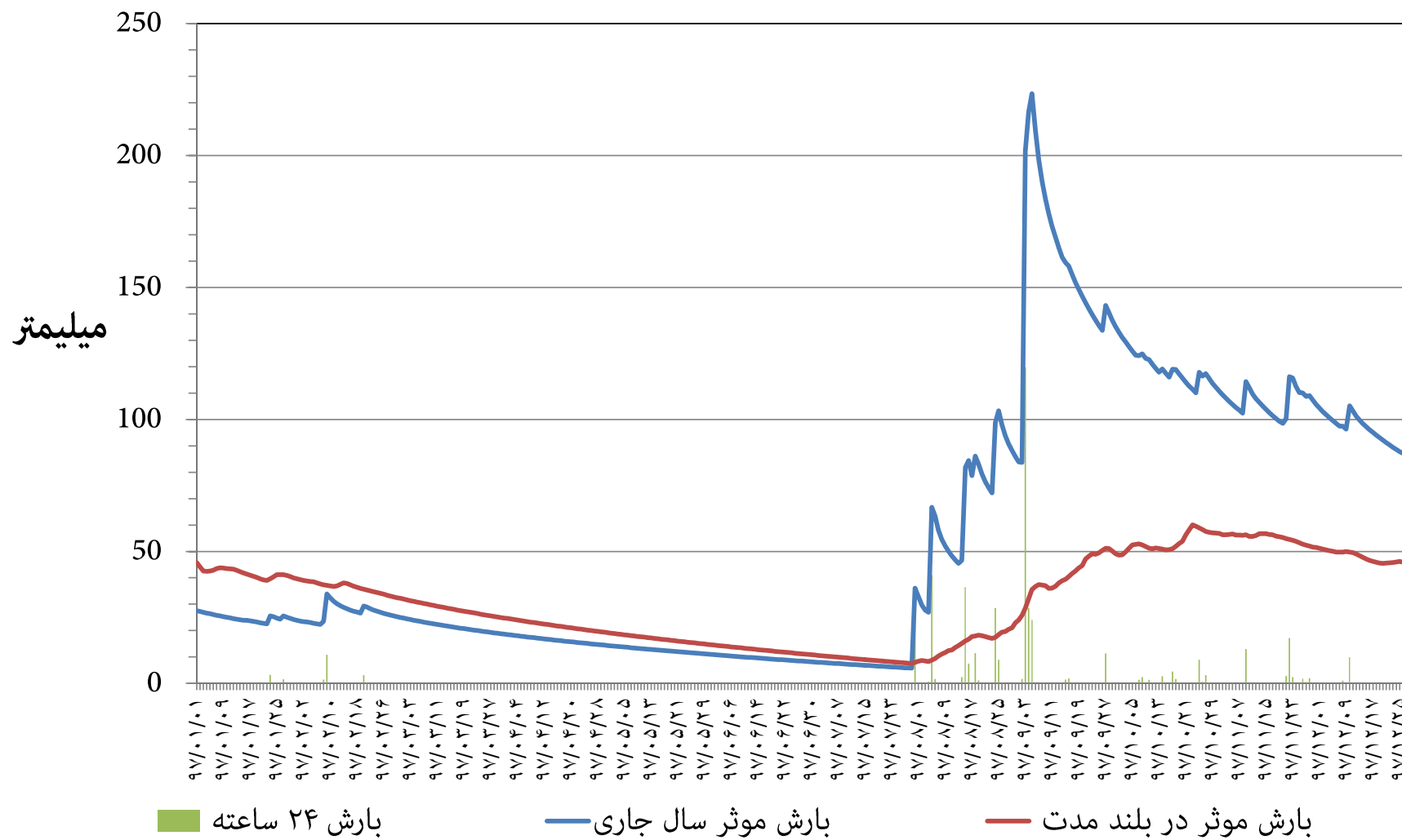
نمودار توزیع زمانی بارش و بارش موثر ۳۶۵ روزه ایستگاه هواشناسی هندیجان استان خوزستان سال شمسی ۱۳۹۷
