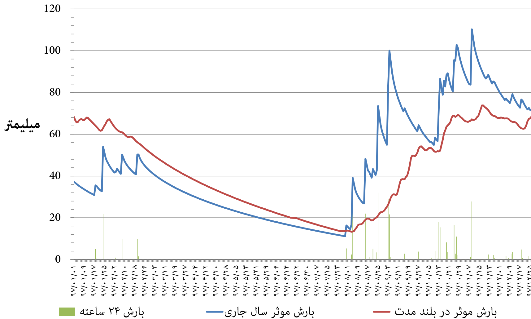
نمودار توزیع زمانی بارش و بارش موثر ۳۶۵ روزه ایستگاه هواشناسی رامهرمز استان خوزستان سال شمسی ۱۳۹۷
