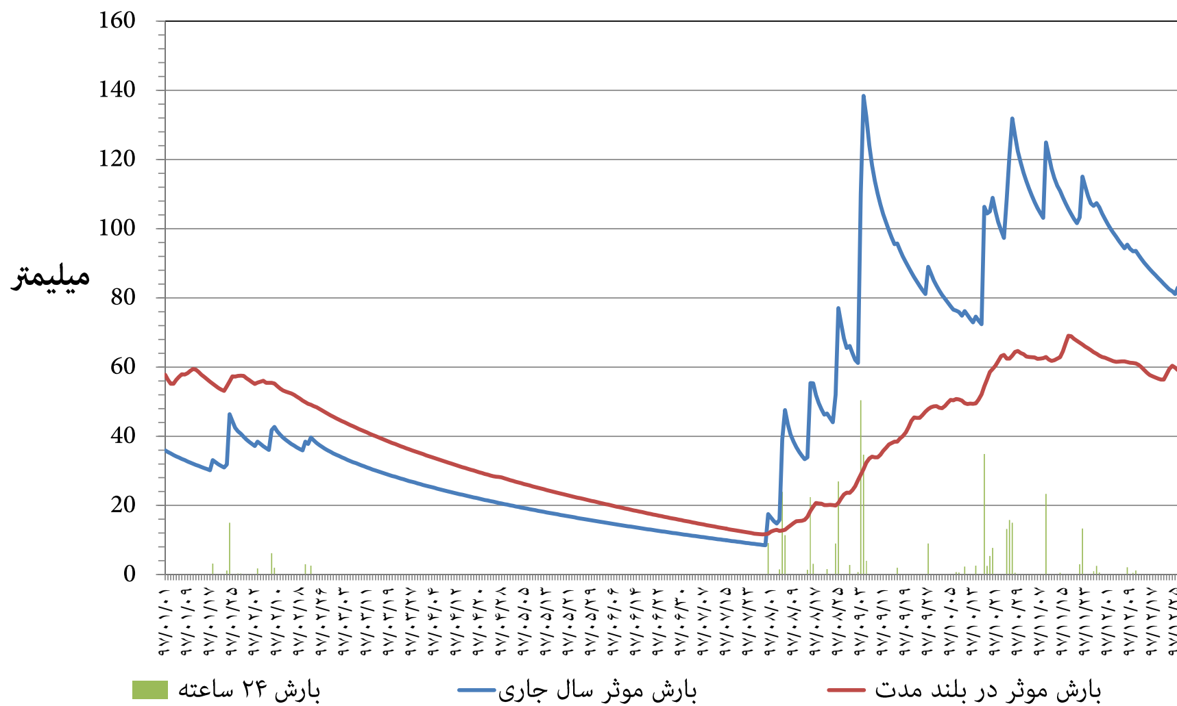
نمودار توزیع زمانی بارش و بارش موثر ۳۶۵ روزه ایستگاه هواشناسی امیدیه (آغاچاری) استان خوزستان سال شمسی ۱۳۹۷
