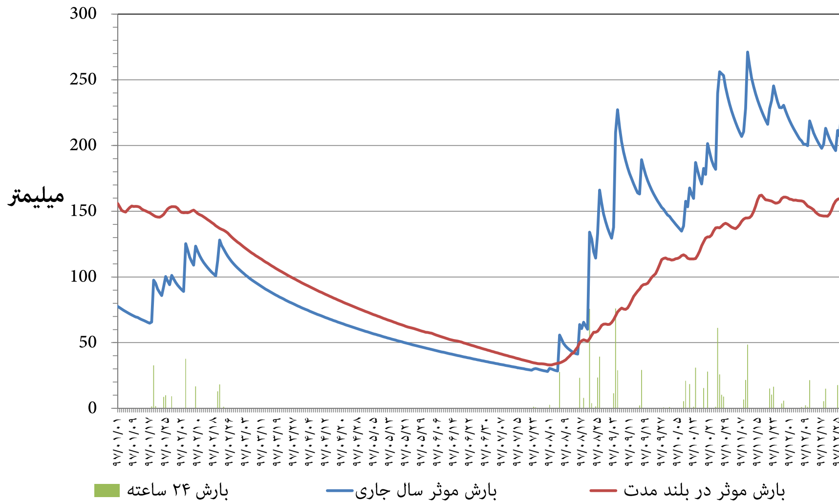
نمودار توزیع زمانی بارش و بارش موثر ۳۶۵ روزه ایستگاه باران سنجی سوسن (وزارت نیرو) استان خوزستان سال شمسی ۱۳۹۷
