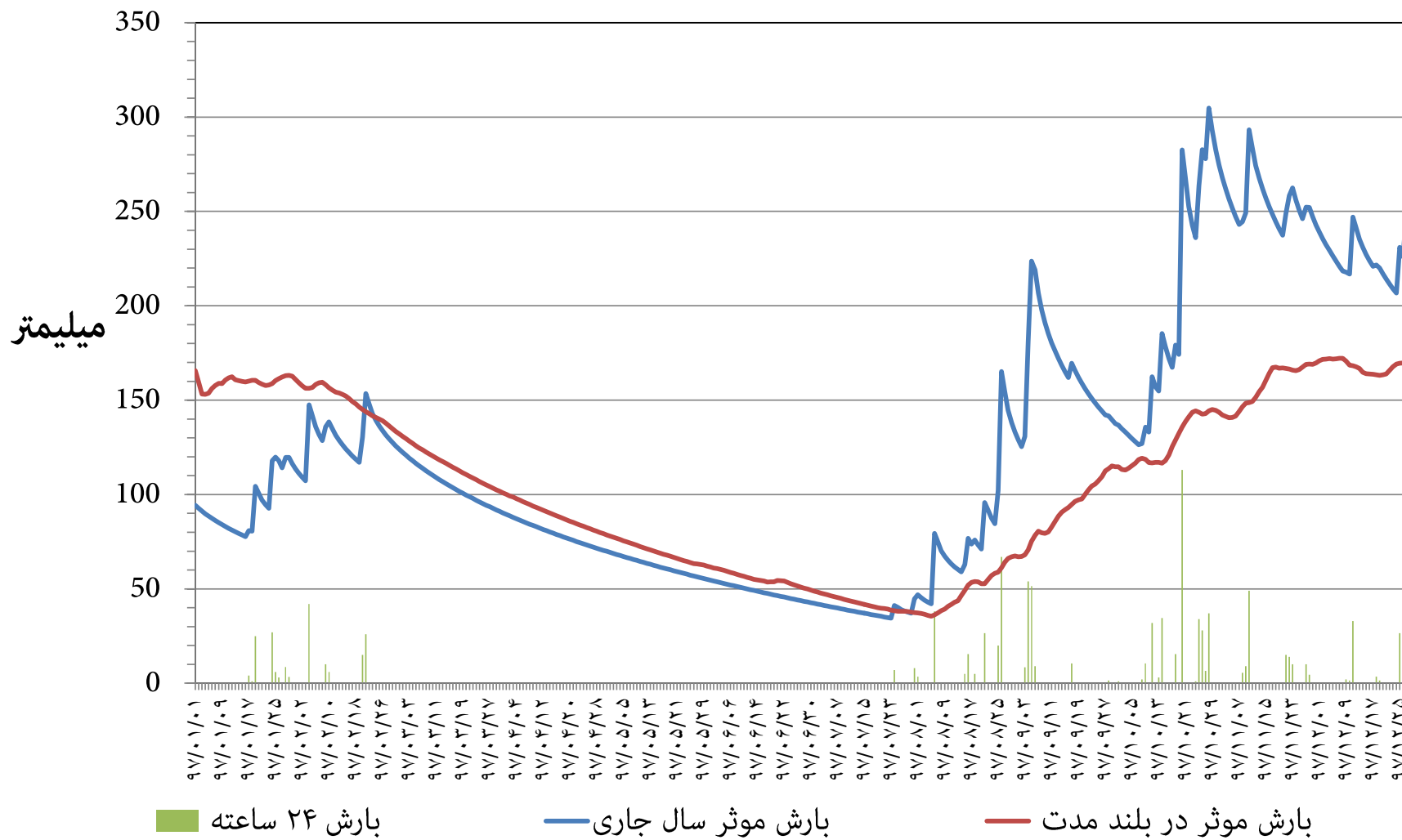
نمودار توزیع زمانی بارش و بارش موثر ۳۶۵ روزه ایستگاه باران سنجی کارون سه (وزارت نیرو) استان خوزستان سال شمسی ۱۳۹۷
