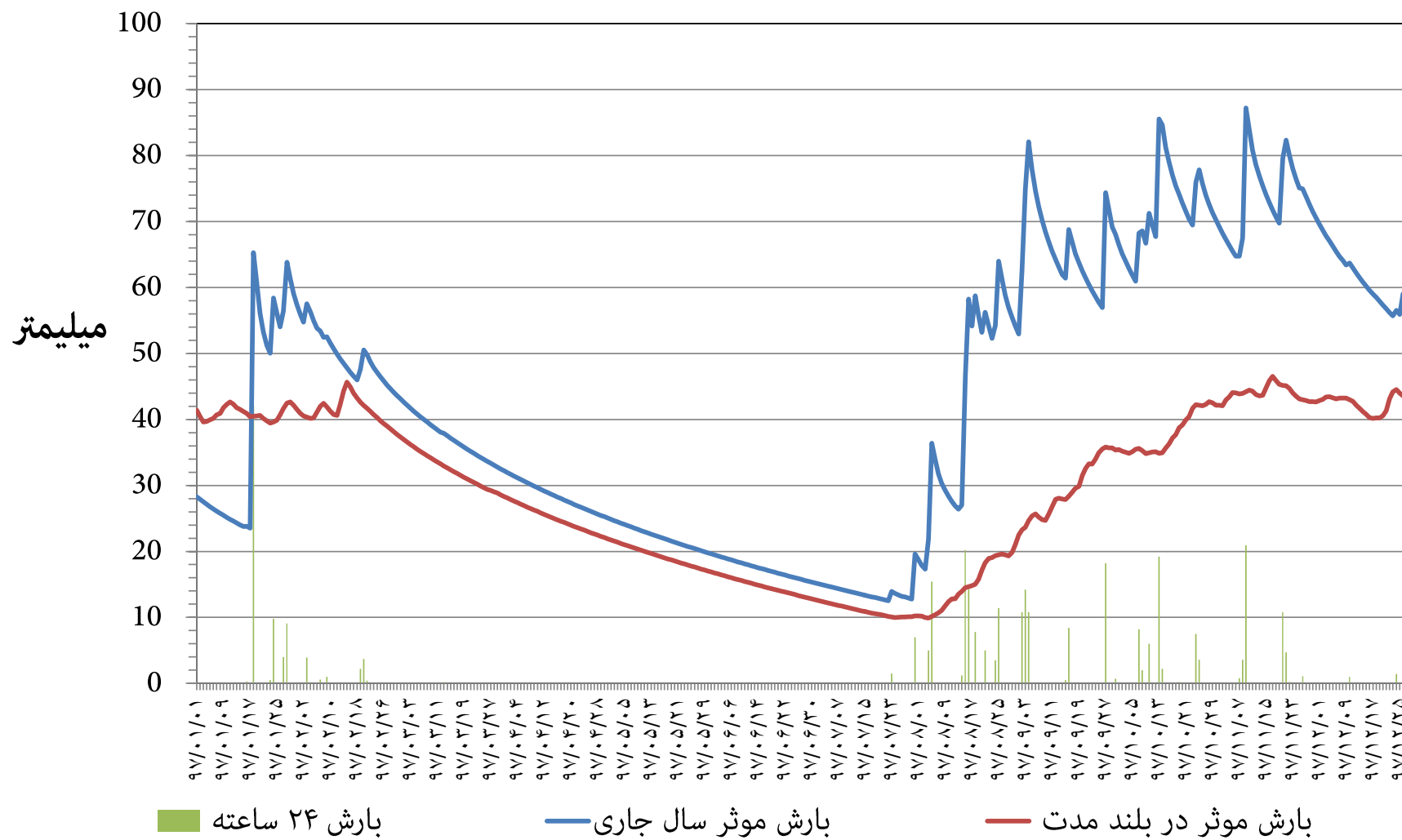
نمودار توزیع زمانی بارش و بارش موثر ۳۶۵ روزه ایستگاه هواشناسی بستان استان خوزستان سال شمسی ۱۳۹۷
