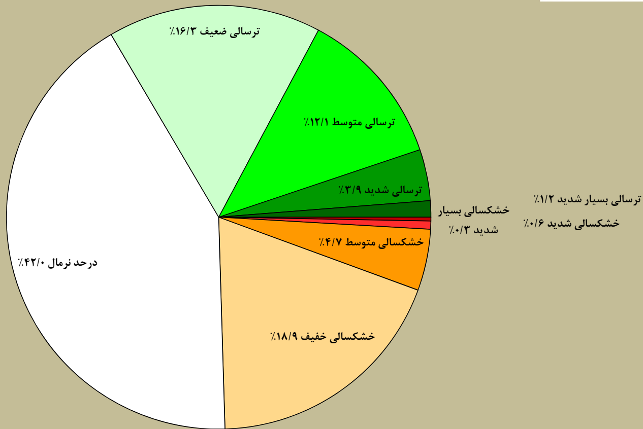
درصد مساحت تحت تاثیر خشکسالی براساس شاخص SPEI دوره یک ساله تا پایان خرداد ماه ۱۳۹۸ در سطح استان مازندران
