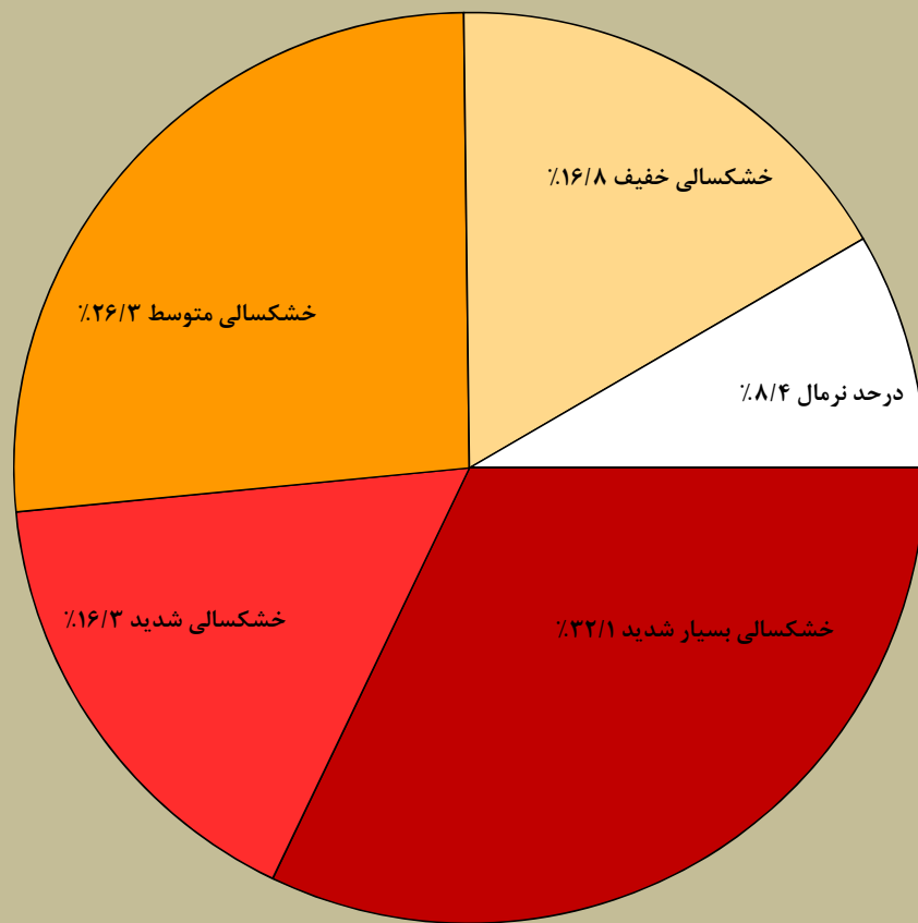
درصد مساحت تحت تاثیر خشکسالی براساس شاخص SPEI دوره ده ساله تا پایان خرداد ماه ۱۳۹۸ در سطح استان کرمان
