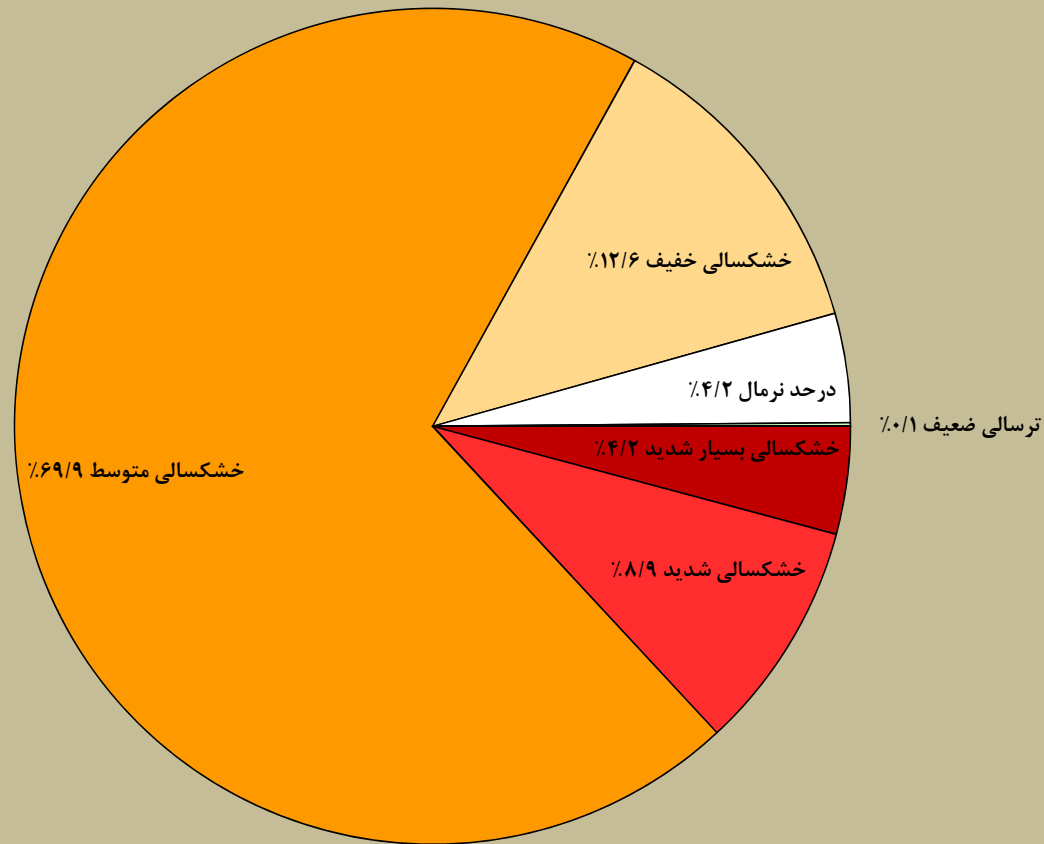
درصد مساحت تحت تاثیر خشکسالی براساس شاخص SPEI دوره ده ساله تا پایان خرداد ماه ۱۳۹۸ در سطح استان فارس
