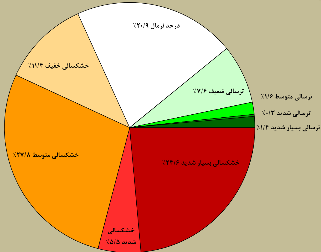
درصد مساحت تحت تاثیر خشکسالی براساس شاخص SPEI دوره ده ساله تا پایان خرداد ماه ۱۳۹۸ در سطح استان خراسان شمالی
