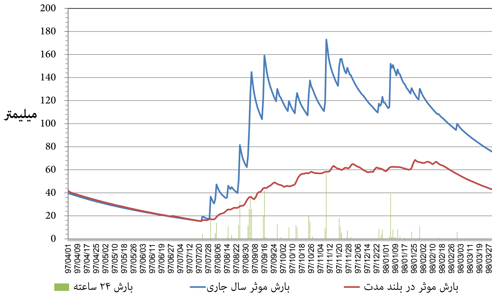
مقدار توزیع زمانی بارش و بارش موثر ۳۶۵ روزه ایستگاه هواشناسی دهلران استان ایلام دوره ۱۲ ماهه تا پایان خرداد ماه ۱۳۹۸
