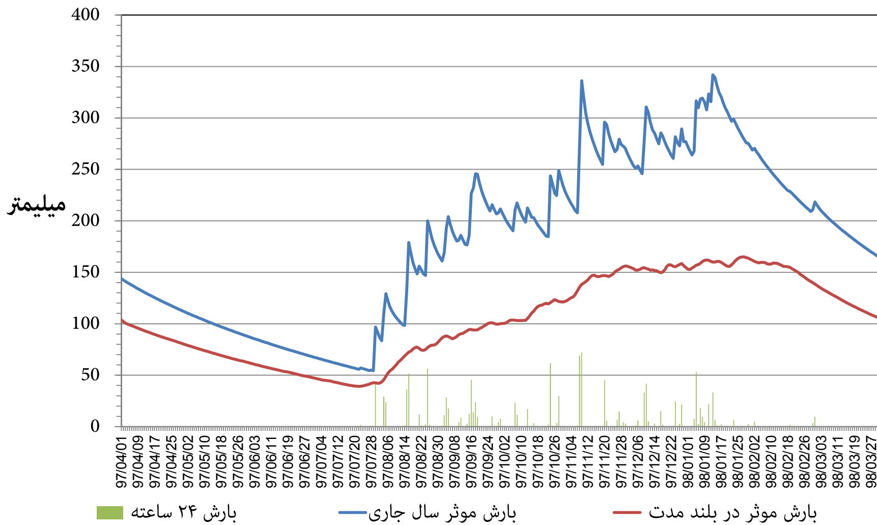
نمودار توزیع زمانی بارش و بارش موثر ۳۶۵ روزه ایستگاه هواشناسی ایوان استان ایلام دوره ۱۲ ماهه تا پایان خرداد ماه ۱۳۹۸
