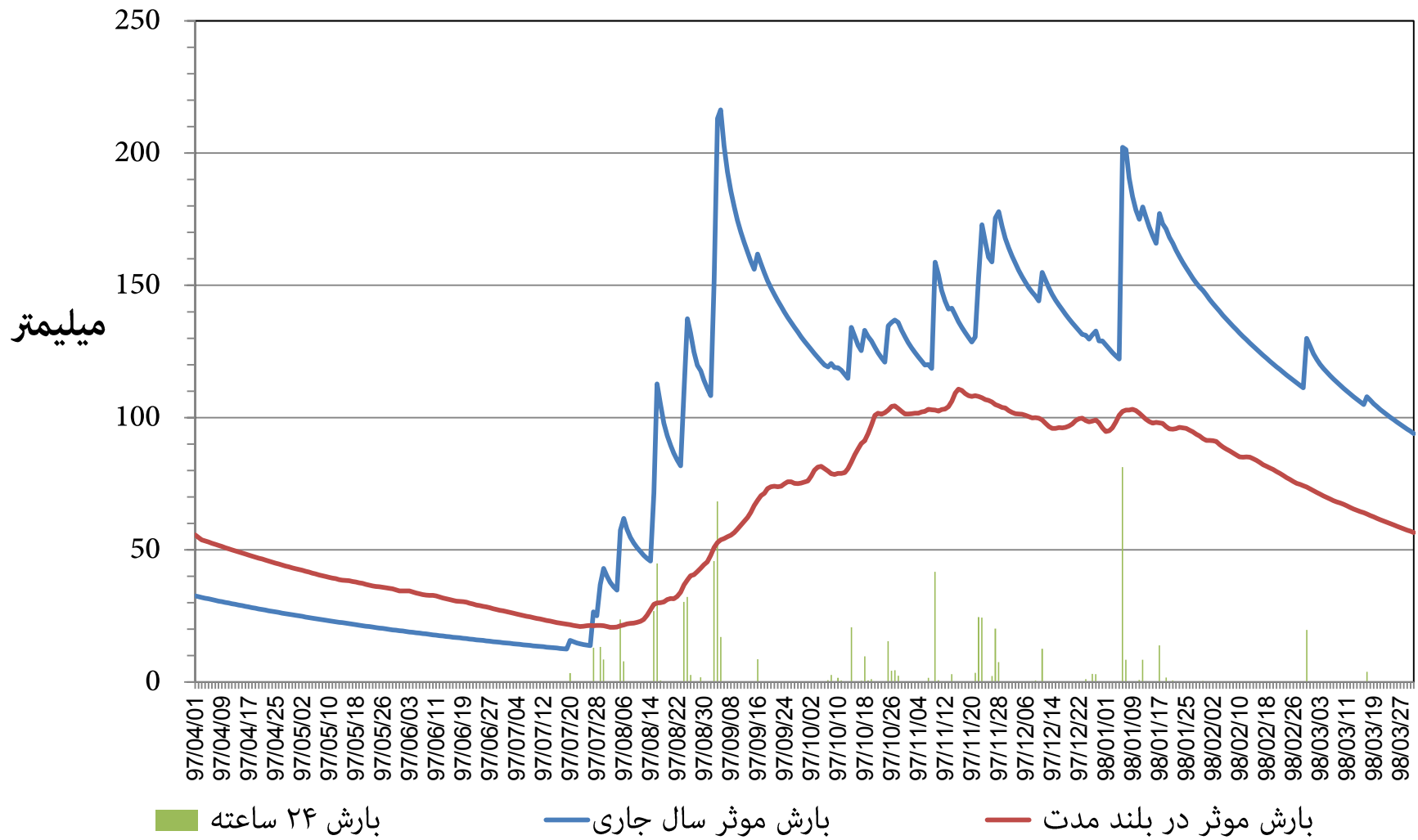
نمودار توزیع زمانی بارش و بارش موثر ۳۶۵ روزه ایستگاه هواشناسی دو گنبدان استان کهگیلویه و بویراحمد دوره ۱۲ ماهه تا پایان خرداد ماه ۱۳۹۸
