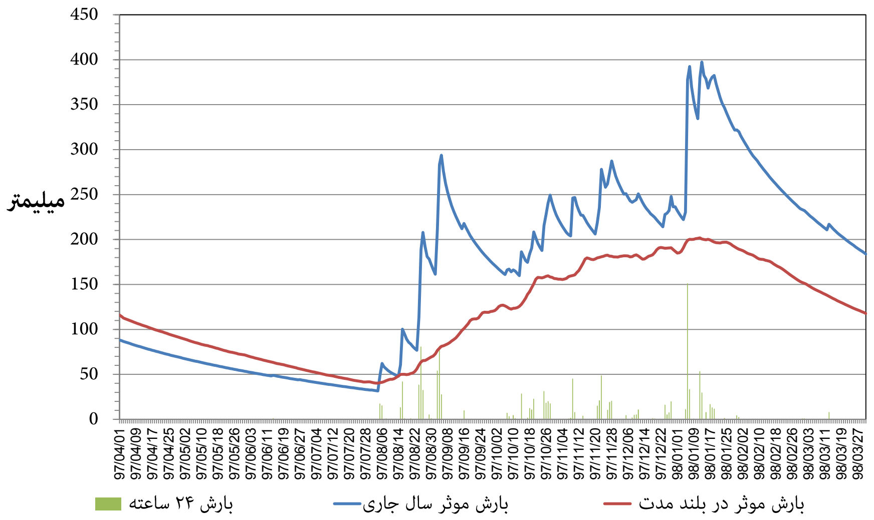
نمودار توزیع زمانی بارش و بارش موثر ۳۶۵ روزه ایستگاه هواشناسی یاسوج استان کهگیلویه و بویراحمد دوره ۱۲ ماهه تا پایان خرداد ماه ۱۳۹۸
