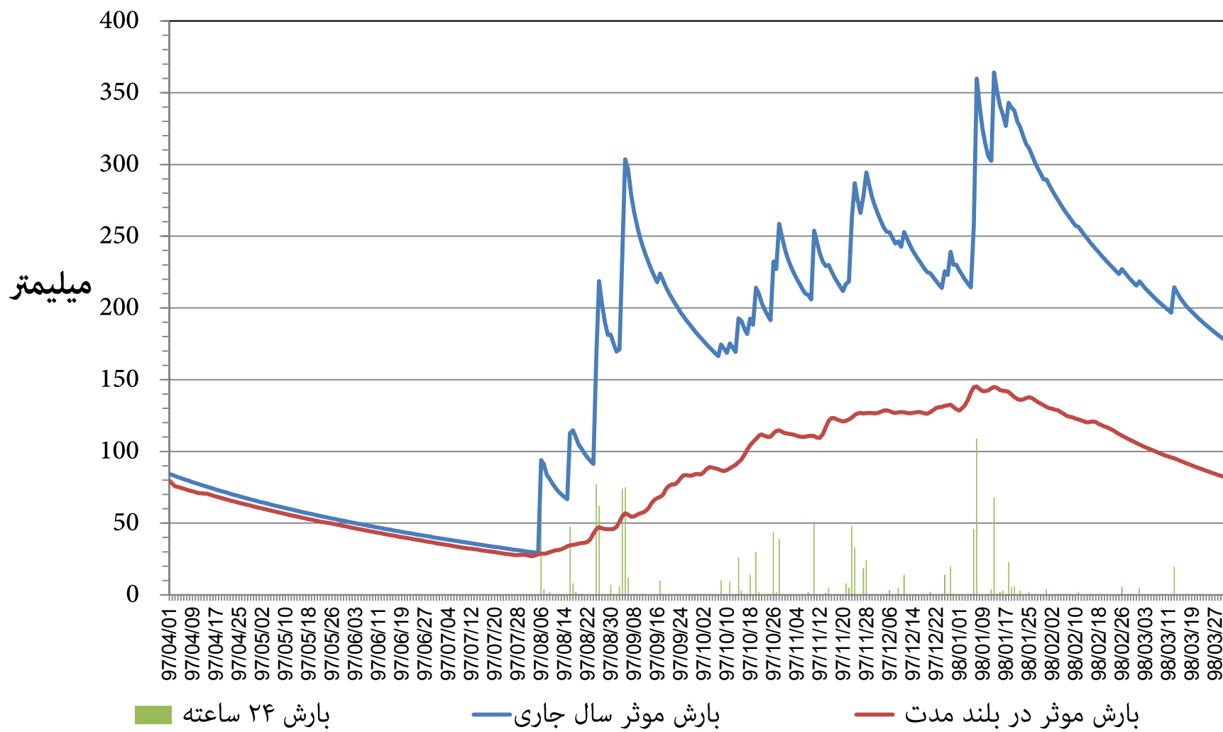
نمودار توزیع زمانی بارش و بارش موثر ۳۶۵ روزه ایستگاه باران سنجی یاسوج (وزارت نیرو) استان کهگیلویه و بویراحمد دوره ۱۲ ماهه تا پایان خرداد ماه ۱۳۹۸
