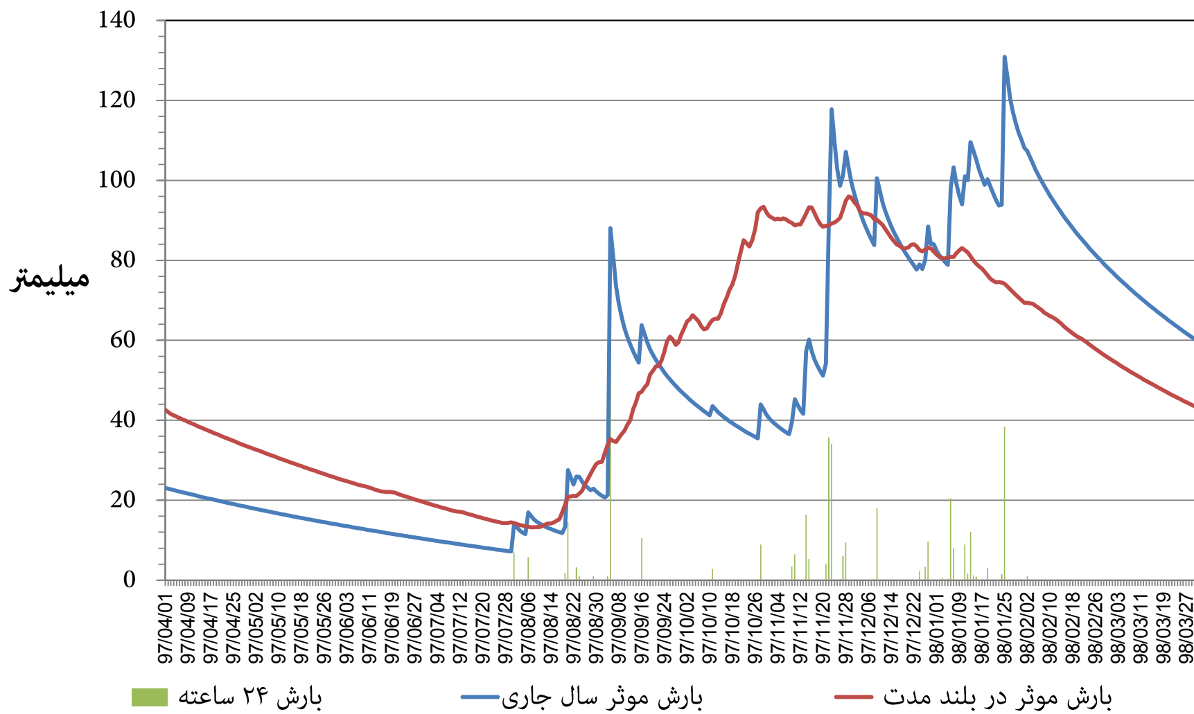
نمودار توزیع زمانی بارش و بارش موثر ۳۶۵ روزه ایستگاه هواشناسی جم استان بوشهر دوره ۱۲ ماهه تا پایان خرداد ماه ۱۳۹۸
