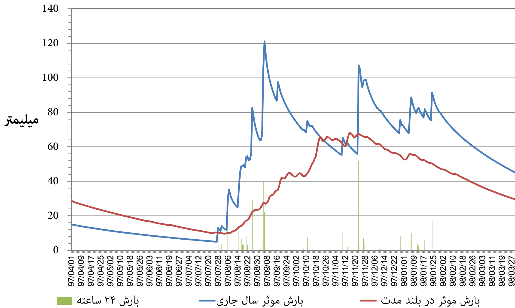
مقدار توزیع زمانی بارش و بارش موثر ۳۶۵ روزه ایستگاه باران سنجی سعد آباد (وزارت نیرو) استان بوشهر دوره ۱۲ ماهه تا پایان خرداد ماه ۱۳۹۸
