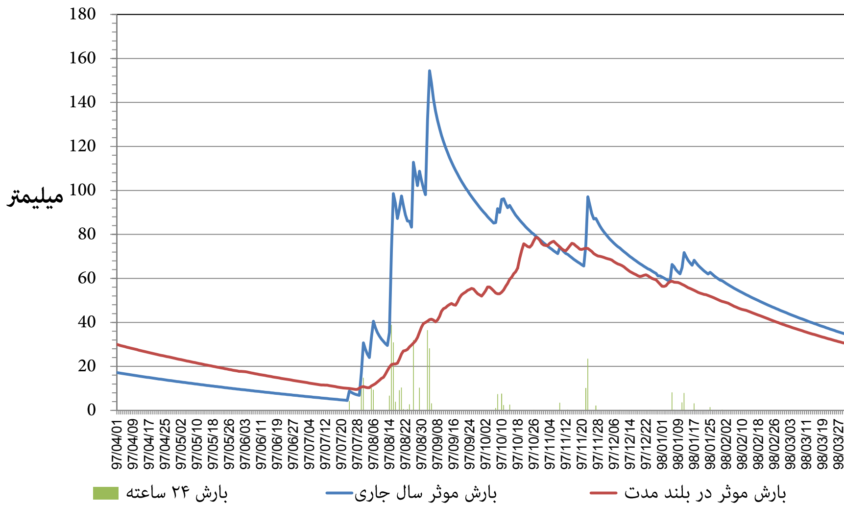
مقدار توزیع زمانی بارش و بارش موثر ۳۶۵ روزه ایستگاه هواشناسی بوشهر (ساحلی) استان بوشهر دوره ۱۲ ماهه تا پایان خرداد ماه ۱۳۹۸
