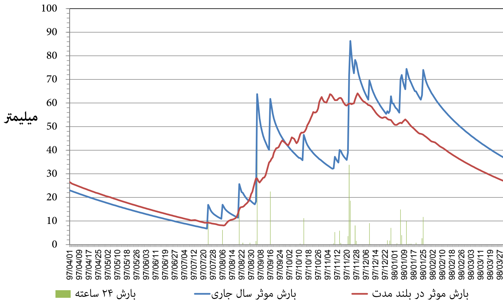
نمودار توزیع زمانی بارش و بارش موثر ۳۶۵ روزه ایستگاه هواشناسی بندر دیر استان بوشهر دوره ۱۲ ماهه تا پایان خرداد ماه ۱۳۹۸
