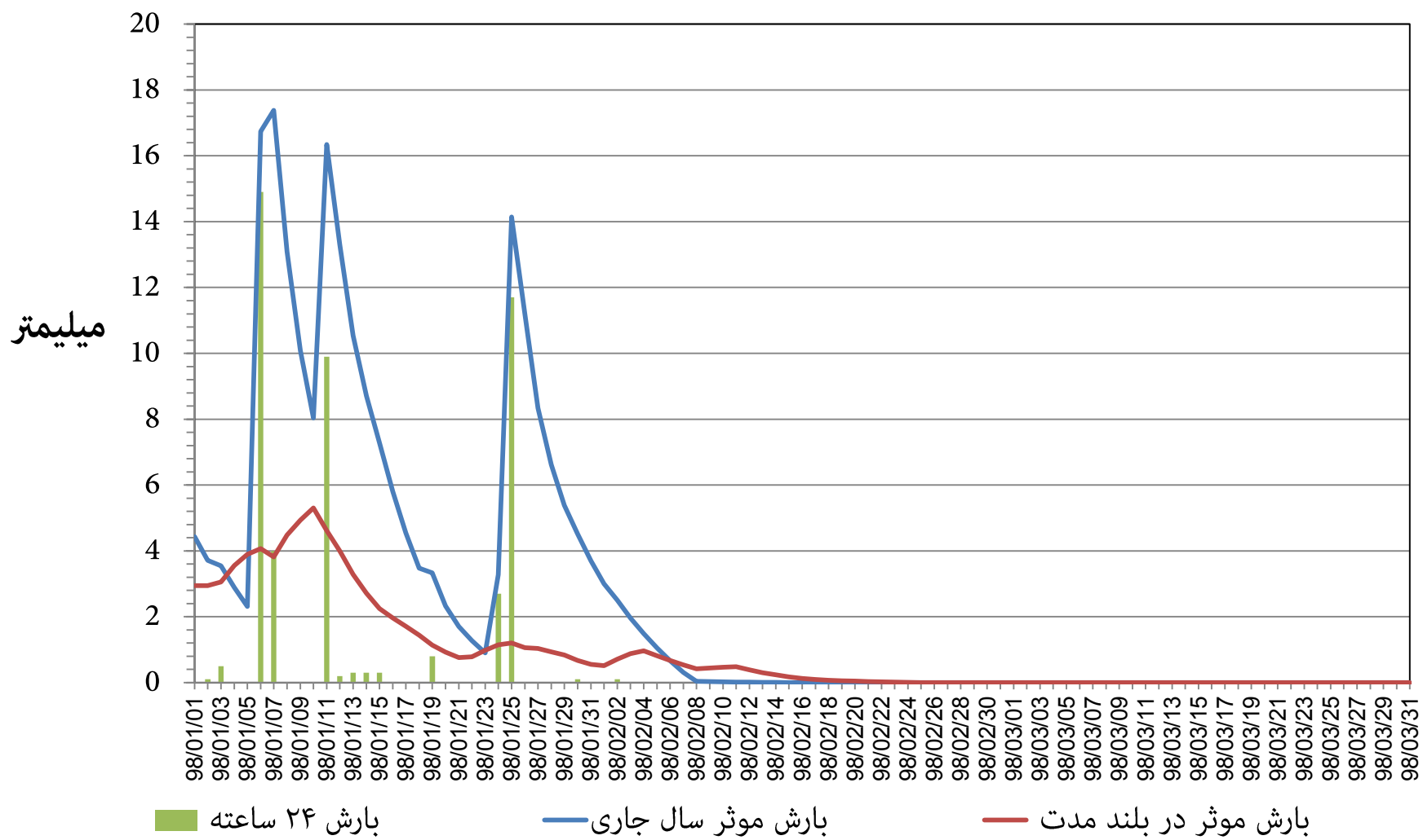
نمودار توزیع زمانی بارش و بارش موثر ۱۴ روزه ایستگاه هواشناسی بندر دیر استان بوشهر فصل بهار ۱۳۹۸
