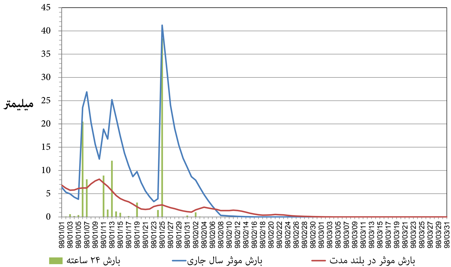
نمودار توزیع زمانی بارش و بارش موثر ۱۴ روزه ایستگاه هواشناسی جم استان بوشهر فصل بهار ۱۳۹۸
