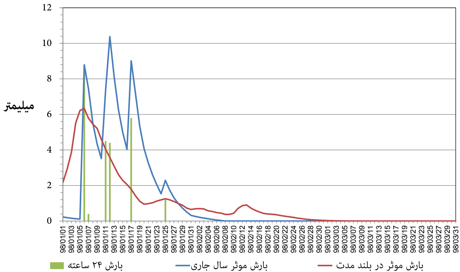
نمودار توزیع زمانی بارش و بارش موثر ۱۴ روزه ایستگاه هواشناسی فرودگاه بوشهر استان بوشهر فصل بهار ۱۳۹۸
