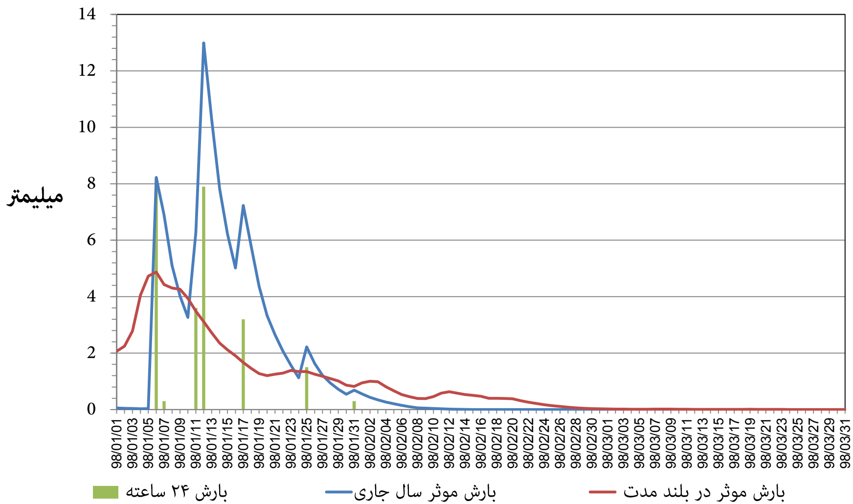
نمودار توزیع زمانی بارش و بارش موثر ۱۴ روزه ایستگاه هواشناسی بوشهر (ساحلی) استان بوشهر فصل بهار ۱۳۹۸
