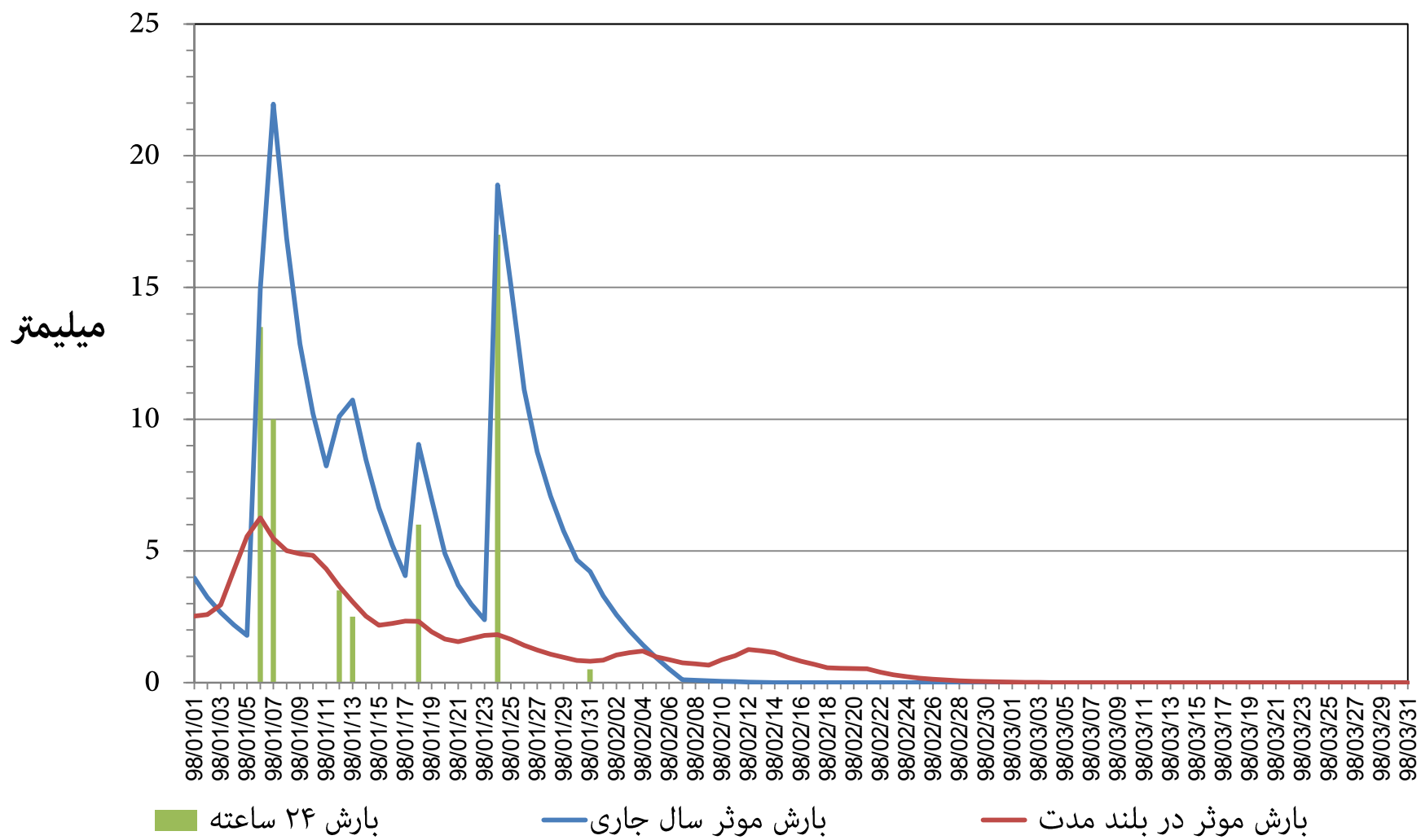
نمودار توزیع زمانی بارش و بارش موثر ۱۴ روزه ایستگاه باران سنجی سعد آباد (وزارت نیرو) استان بوشهر فصل بهار ۱۳۹۸
