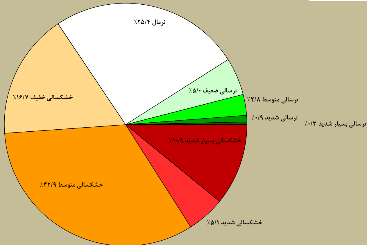
درصد مساحت تحت تاثیر خشکسالی براساس شاخص SPEI دوره ده ساله تا پایان تیر ماه ۱۳۹۸ در سطح استان مازندران
