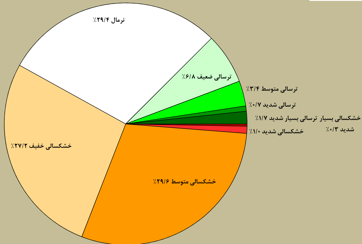
درصد مساحت تحت تاثیر خشکسالی براساس شاخص SPEI دوره ده ساله تا پایان تیر ماه ۱۳۹۸ در سطح استان کردستان
