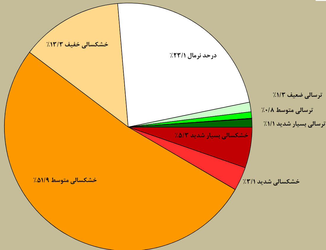
درصد جمعیت تحت تاثیر خشکسالی براساس شاخص SPEI دوره ده ساله تا پایان تیر ماه ۱۳۹۸ در سطح استان چهارمحال و بختیاری
