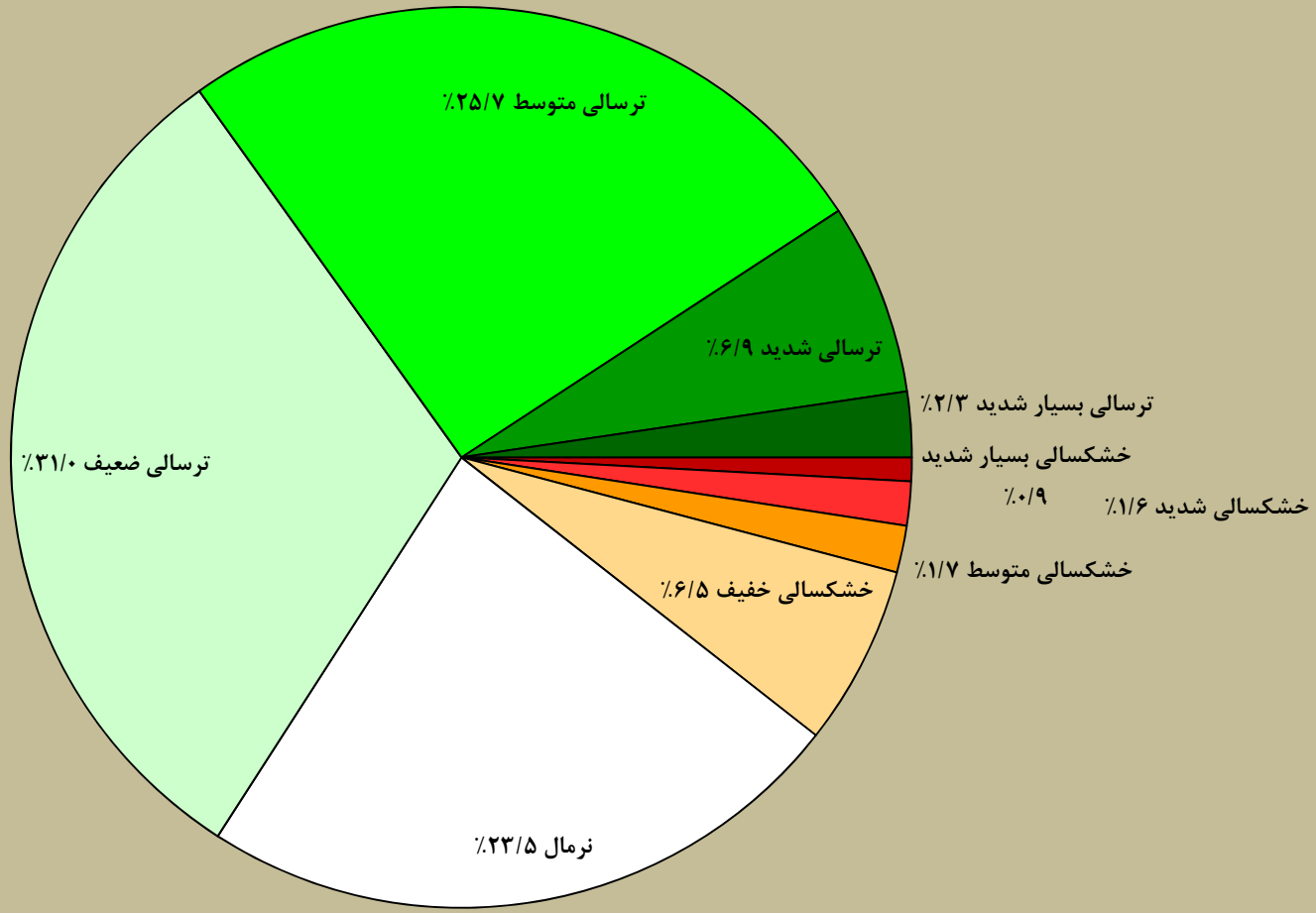
درصد مساحت تحت تاثیر خشکسالی براساس شاخص SPEI دوره یک ساله تا پایان مرداد ماه ۱۳۹۸ در سطح استان خراسان شمالی
