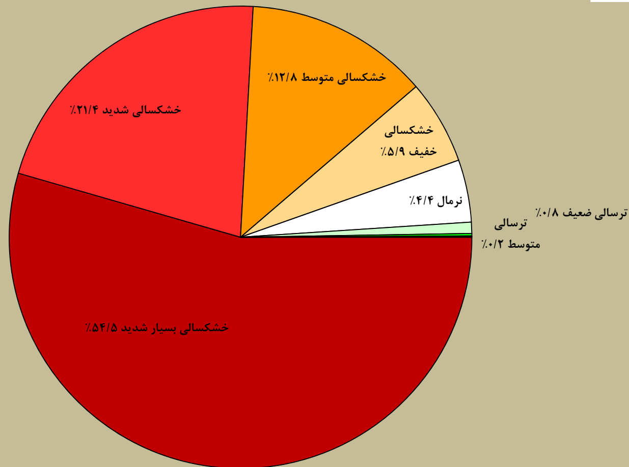
درصد مساحت تحت تاثیر خشکسالی براساس شاخص SPEI دوره ده ساله تا پایان مرداد ماه ۱۳۹۸ در سطح استان اصفهان
