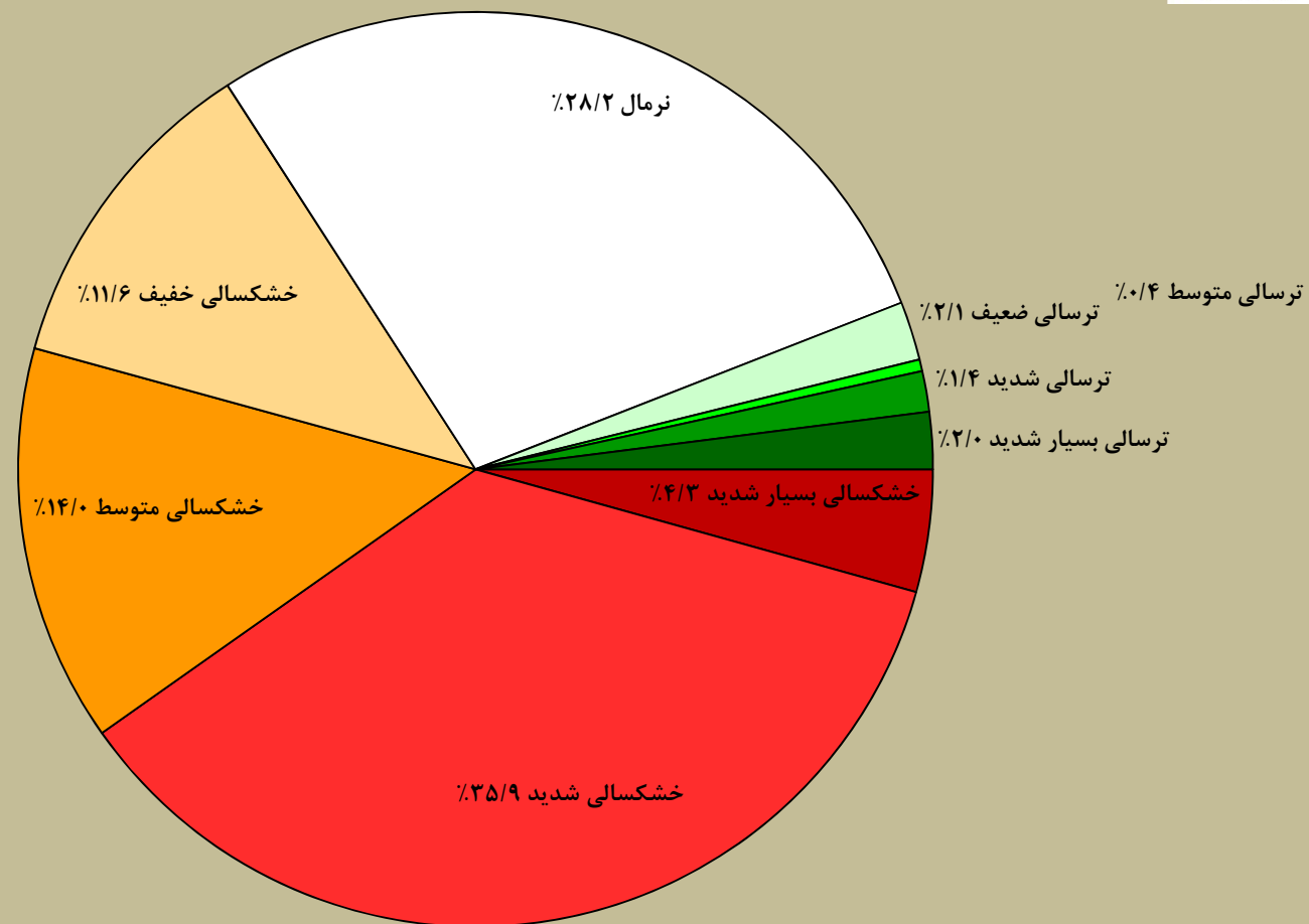
درصد مساحت تحت تاثیر خشکسالی براساس شاخص SPEI دوره ده ساله تا پایان مرداد ماه ۱۳۹۸ در سطح استان چهارمحال و بختیاری
