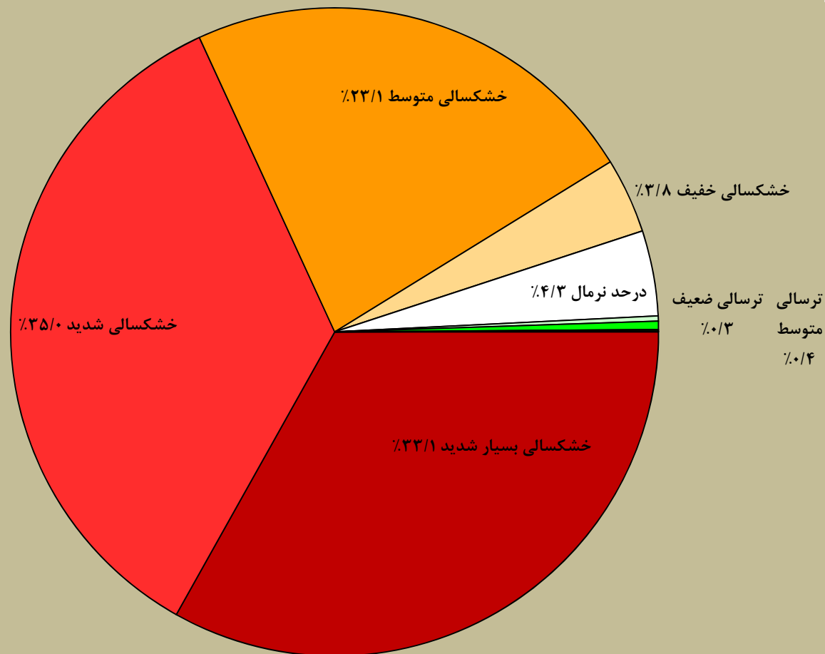
درصد جمعیت تحت تاثیر خشکسالی براساس شاخص SPEI دوره ده ساله تا پایان مرداد ماه ۱۳۹۸ در سطح استان اصفهان
