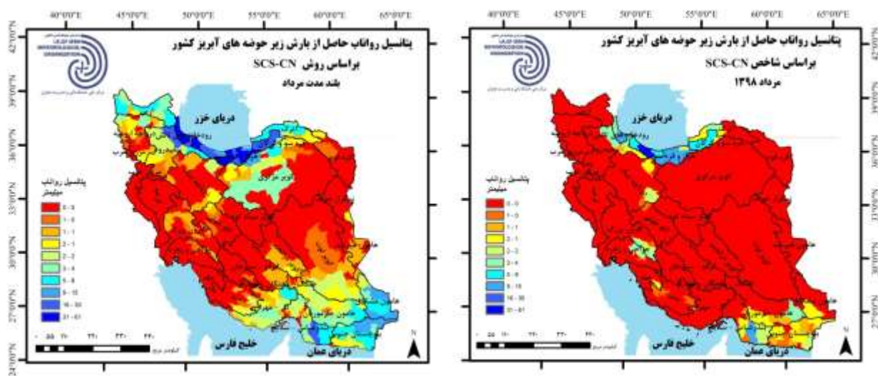
شکل ۲- پتانسیل رواناب حوزه‌های آبریز کشور در مرداد ماه ۹۸ و دوره بلندمدت با استفاده از روش SCS-CN
