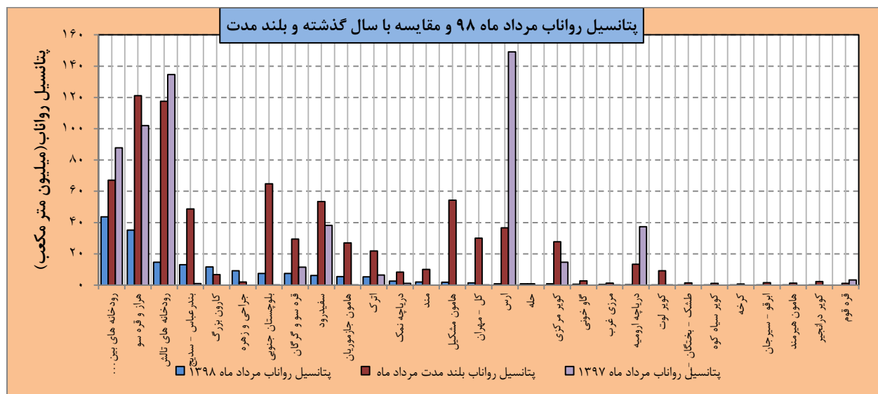
شکل ۳- نمودار پتانسیل رواناب مرداد ماه ۹۸ و مقایسه با بلندمدت به تفکیک حوزه‌های آبریز درجه ۲ کشور
