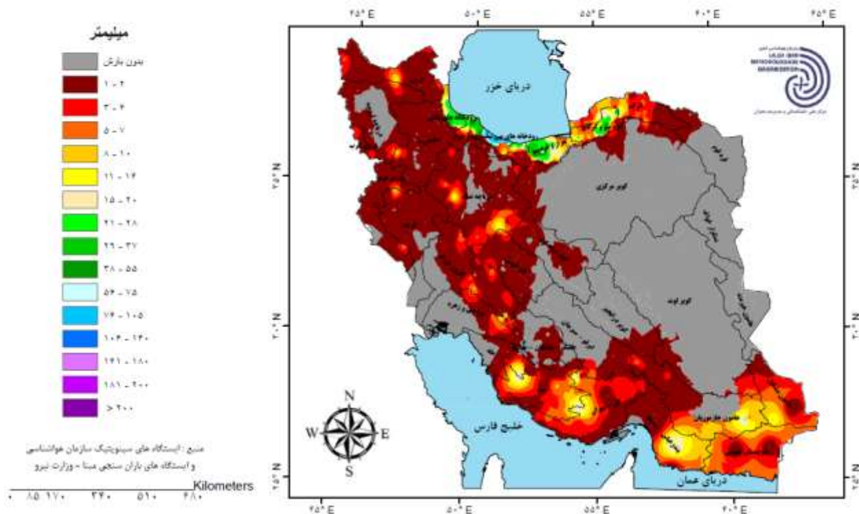
شکل ۱- پهنه بندی مجموع بارش در سطح حوضه های آبریز کشور در مرداد ماه ۱۳۹۸
