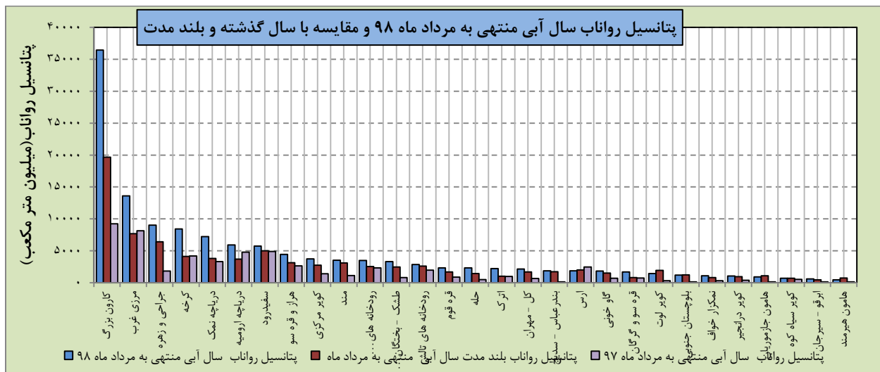
شکل ۵- نمودار پتانسیل رواناب سال آبی منتهی به مرداد ماه ۹۸ و مقایسه با بلندمدت به تفکیک حوضه‌های آبریز درجه ۲ کشور
