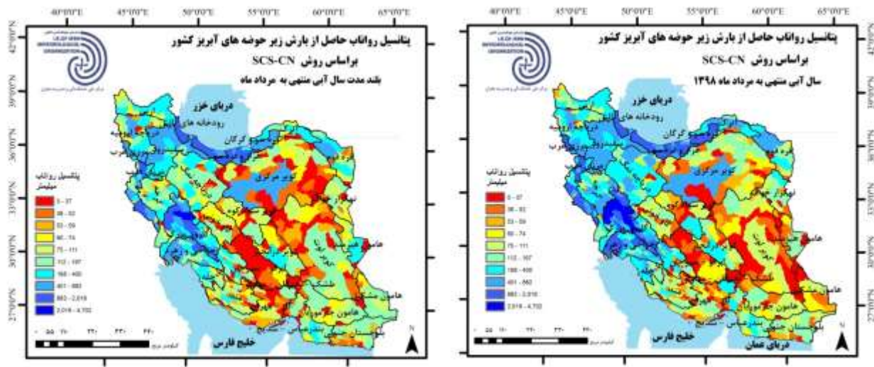
شکل ۴- پتانسیل رواناب حوضه‌های آبریز کشور در سال آبی منتهی به مرداد ماه و دوره بلندمدت با استفاده از روش SCS-CN
