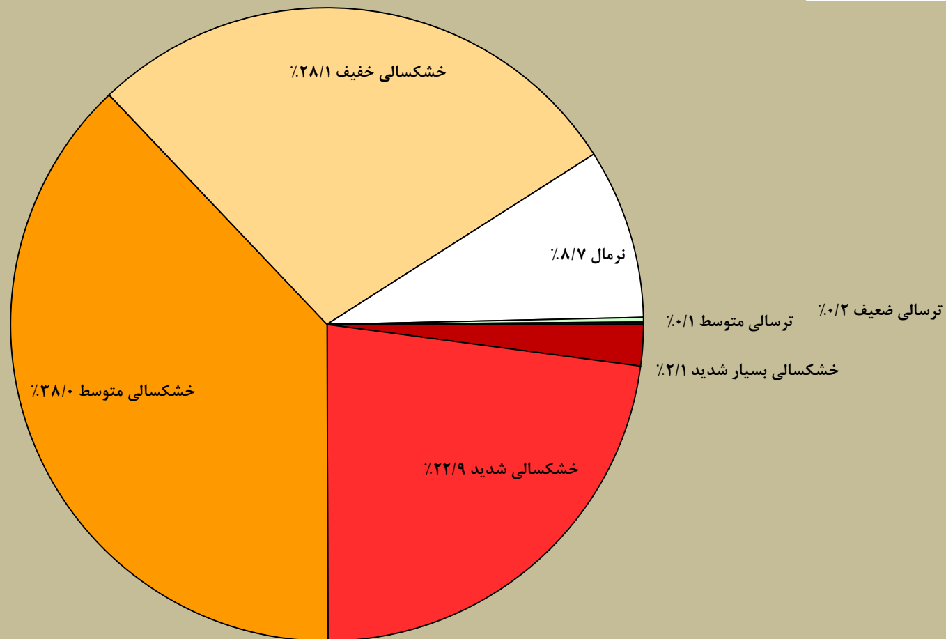
درصد مساحت تحت تاثیر خشکسالی براساس شاخص SPEI دوره ده ساله تا پایان شهریور ماه ۱۳۹۸ در سطح استان زنجان
