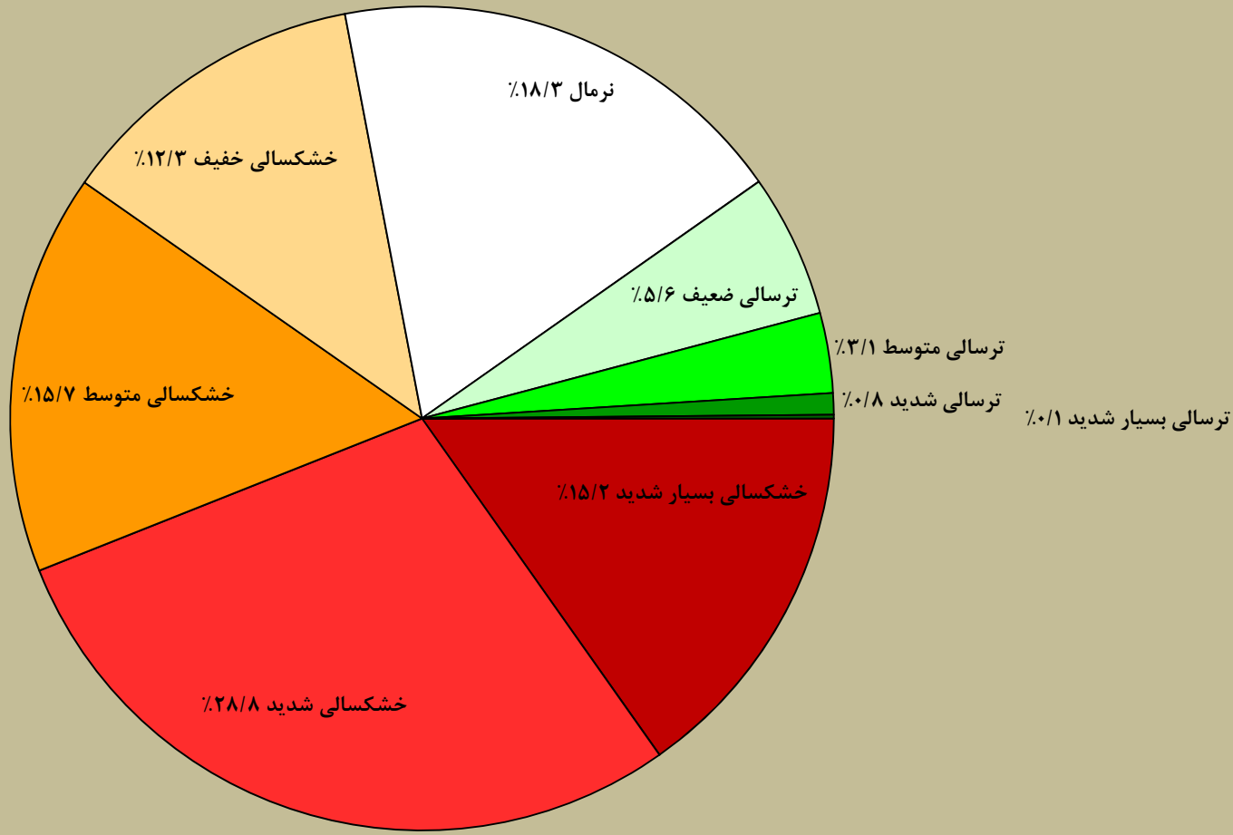
درصد مساحت تحت تاثیر خشکسالی براساس شاخص SPEI دوره ده ساله تا پایان شهریور ماه ۱۳۹۸ در سطح استان خراسان شمالی
