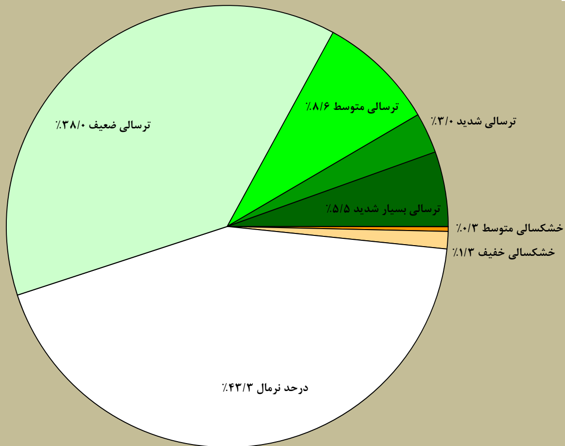
درصد جمعیت تحت تاثیر خشکسالی براساس شاخص SPEI دوره یک ساله تا پایان شهریور ماه ۱۳۹۸ در سطح استان کردستان
