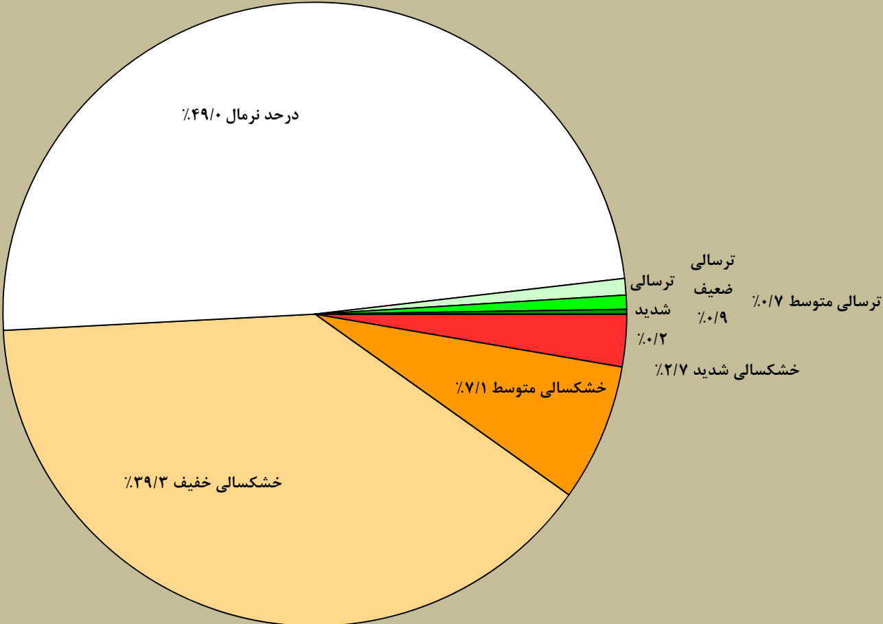
درصد جمعیت تحت تاثیر خشکسالی براساس شاخص SPEI دوره ده ساله تا پایان شهریور ماه ۱۳۹۸ در سطح استان همدان
