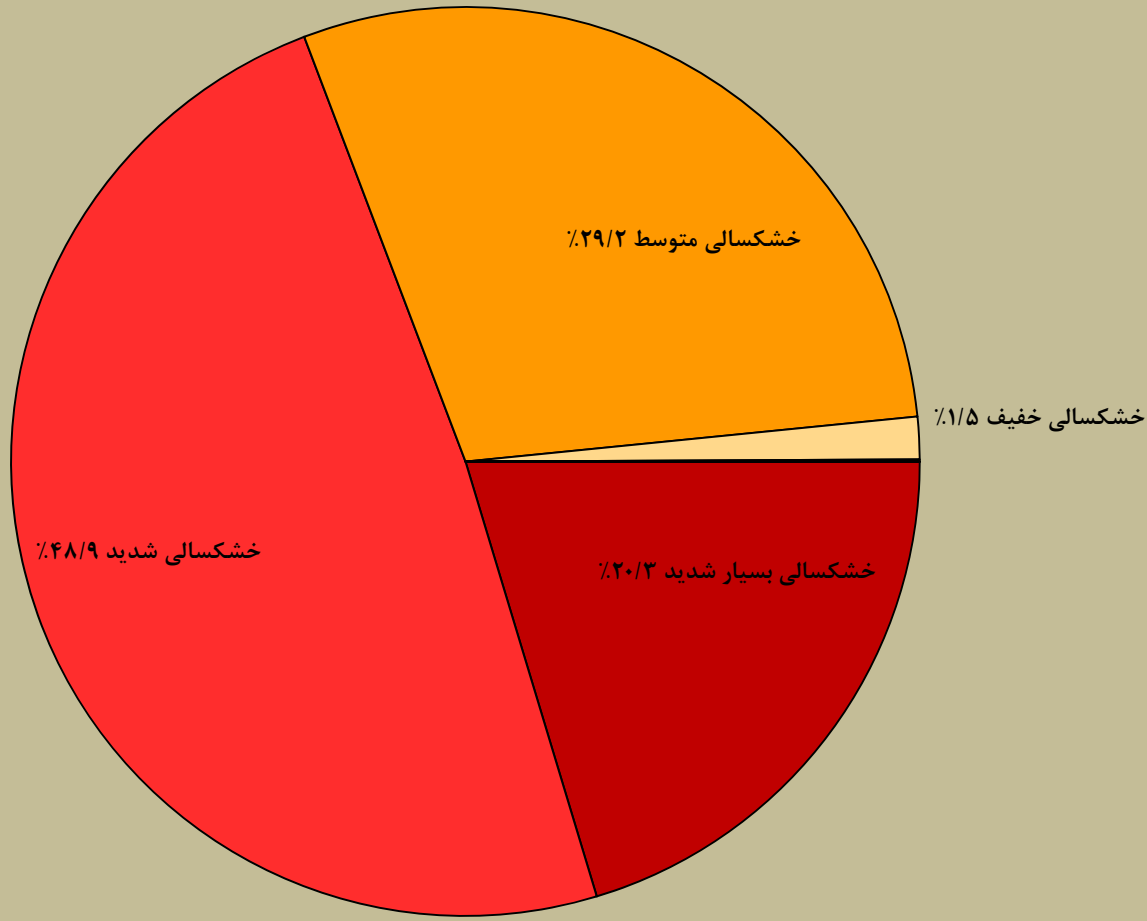
درصد جمعیت تحت تاثیر خشکسالی براساس شاخص SPEI دوره ده ساله تا پایان شهریور ماه ۱۳۹۸ در سطح استان سیستان و بلوچستان
