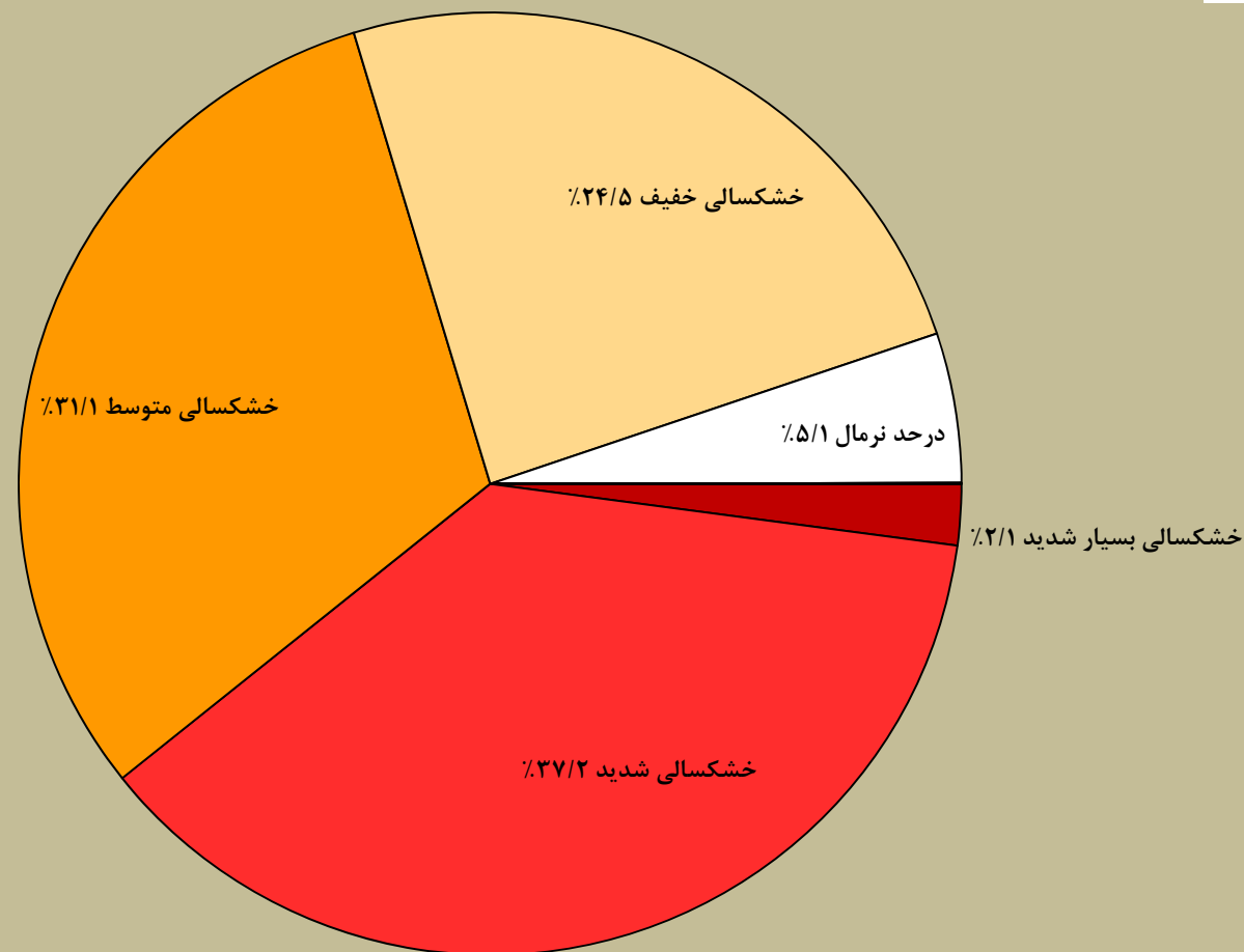
درصد جمعیت تحت تاثیر خشکسالی براساس شاخص SPEI دوره ده ساله تا پایان شهریور ماه ۱۳۹۸ در سطح استان زنجان
