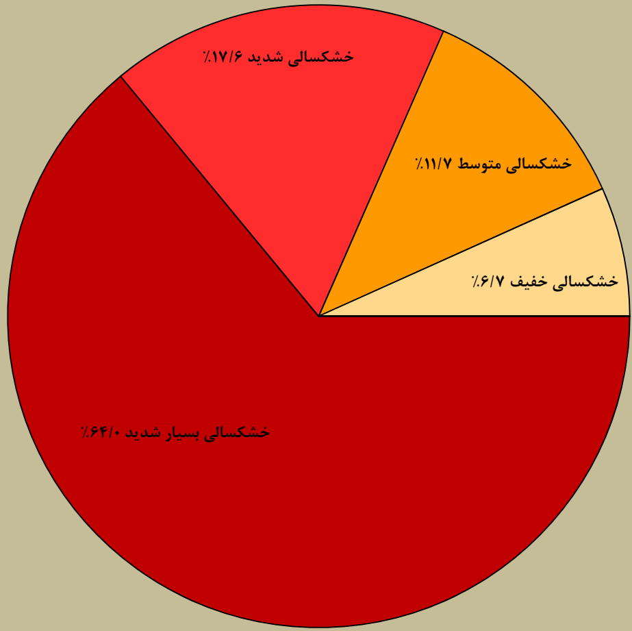
درصد جمعیت تحت تاثیر خشکسالی براساس شاخص SPEI دوره ده ساله تا پایان شهریور ماه ۱۳۹۸ در سطح استان خراسان جنوبی
