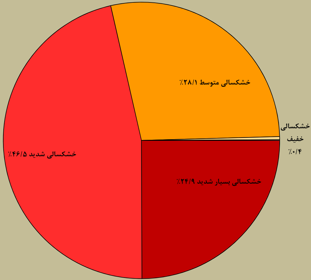
درصد جمعیت تحت تاثیر خشکسالی براساس شاخص SPEI دوره ده ساله تا پایان مهر ماه ۱۳۹۸ در سطح استان سیستان و بلوچستان
